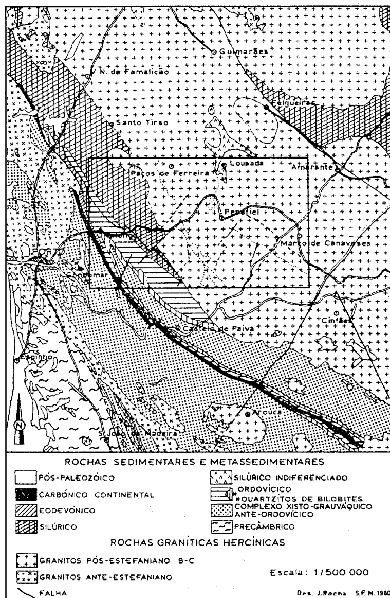
Fig. 2.12. – Enquadramento geológico regional da Carta Geológica (9D) extraído da Carta Geológica de Portugal (4ª edição, de 1972) (In. A.C. Medeiros, E. Pereira & A. Moreira, 1980)
