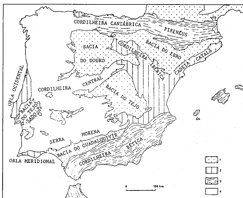
Fig. 2.7. – Unidades morfo-estruturais da Península Ibérica, segundo H. Lautensach (In. A.M. Galopim de Carvalho, 1984)
