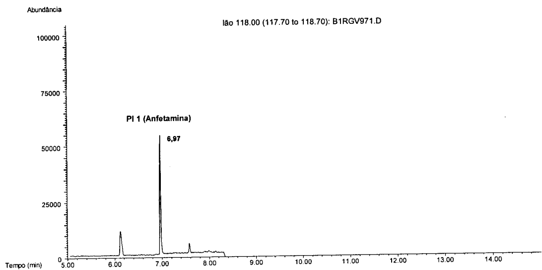
Figura 4.5. Cromatograma de massa do ião m/z 118, usado para a "quantificação" da anfetamina (padrão interno 1).
