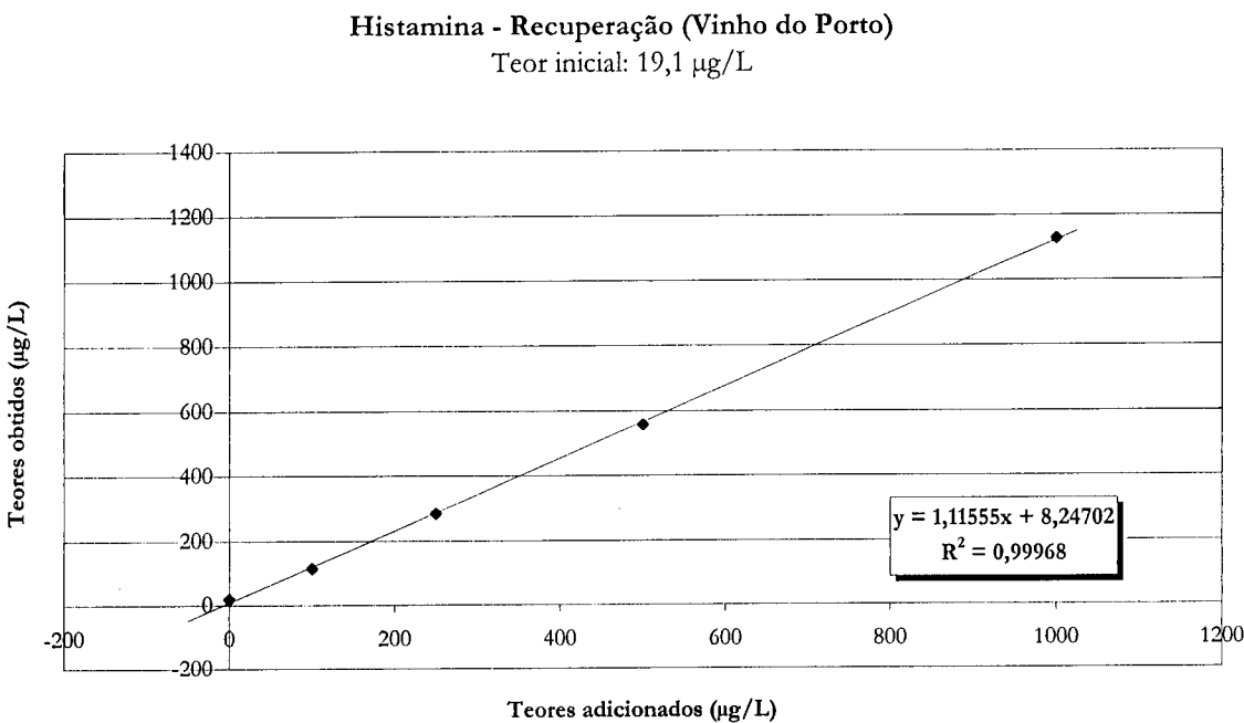
Figura 5.4. Curva de recuperação obtida pela adição de quantidades conhecidas de histamina a uma amostra de vinho do Porto.
