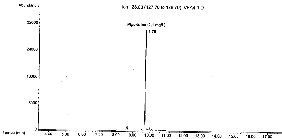
Figura 6.14. Cromatograma de massa do íon m/z 128, usado para a quantificação da piperidina.
