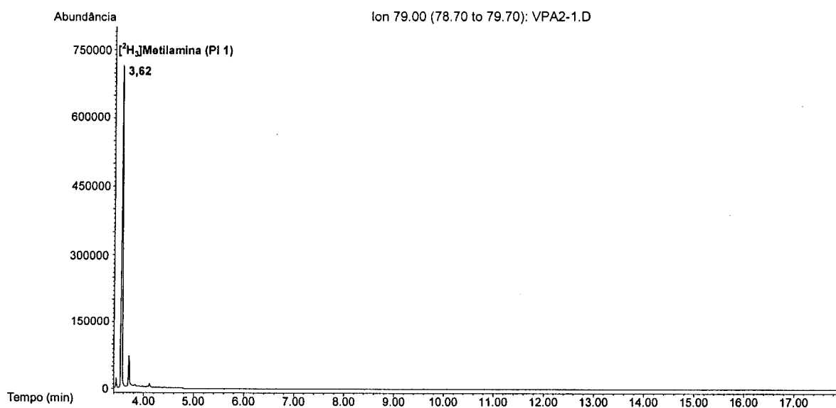
Figura 6.21. Cromatograma de massa do íon m/z 79, usado para a "quantificação" da [^2\text{H}_3] metilamina (PI 1).
