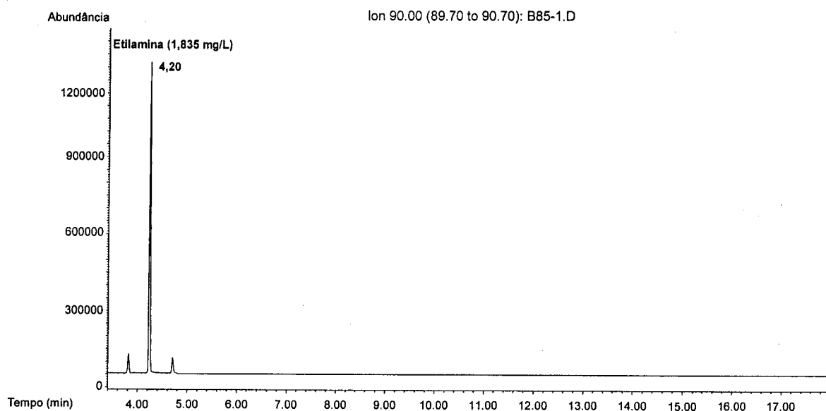
Figura 6.32. Cromatograma de massa do íon m/z 90, usado para a quantificação da etilamina.
