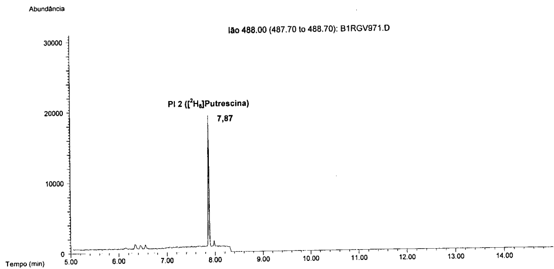
Figura 4.9. Cromatograma de massa do íon m/z 488, usado para a quantificação da [ ^2\text{H}_8 ]Putrescina (padrão interno 2).
