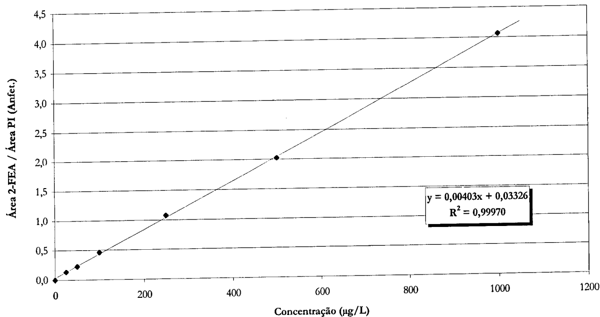
2-Feniletilamina - Curva de Calibração (1)
