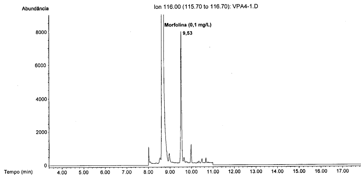
Figura 6.12. Cromatograma de massa do íon m/z 116, usado para a quantificação da morfolina.
