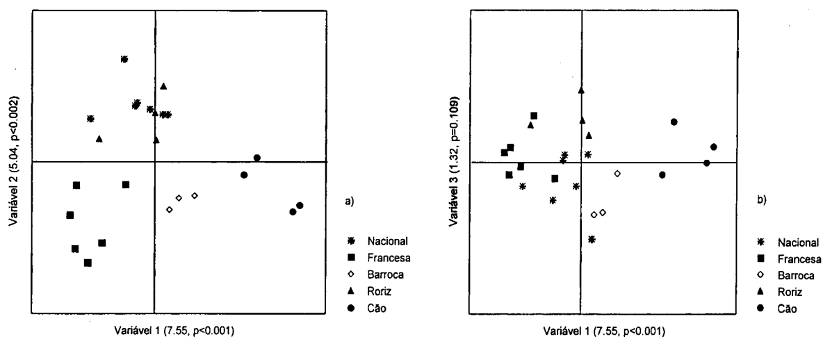
Figura 7.1. Análise discriminante de mostos por castas — a) variáveis canónicas 1 e 2; b) variáveis canónicas 1 e 3. Os valores entre parêntesis correspondem ao valor próprio e à significância de cada variável.
