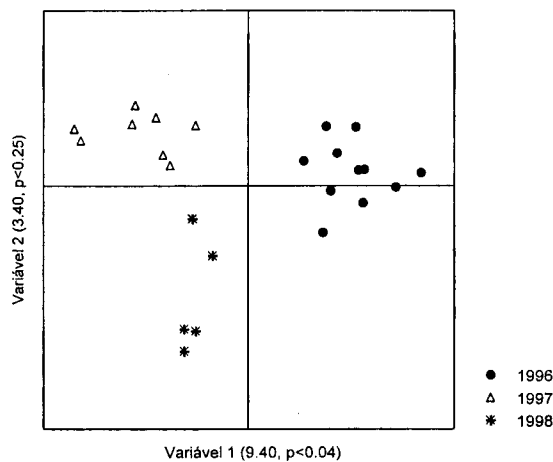
Figura 7.2. Análise discriminante de mostos por anos. Os valores entre parêntesis correspondem ao valor próprio e à significância de cada variável.
