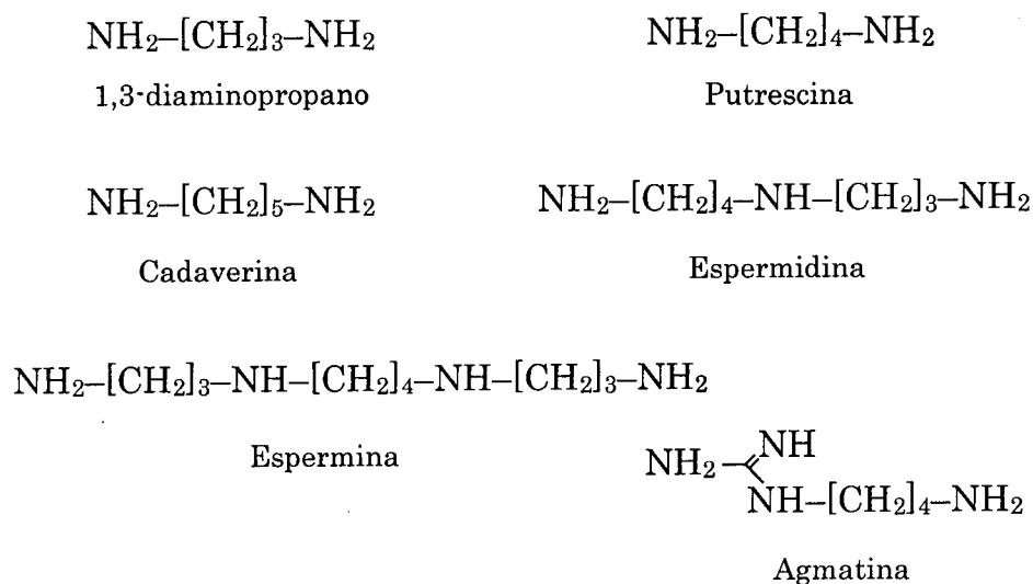
Figura 1.6. Estrutura das diaminas e poliaminas: 1,3-diaminopropano, putrescina, cadaverina, espermidina, espermina e agmatina
