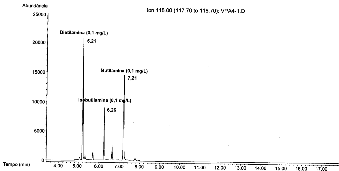
Figura 6.6. Cromatograma de massa do ião m/z 118, usado para a quantificação da dietilamina, da isobutilamina e da butilamina.
