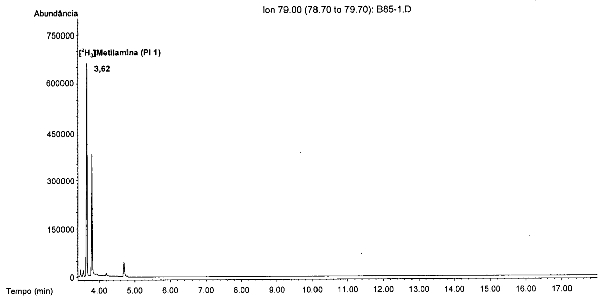
Figura 6.39. Cromatograma de massa do íon m/z 79, usado para a "quantificação" da [ ^2\text{H}_3 ]metilamina (PI 1).
