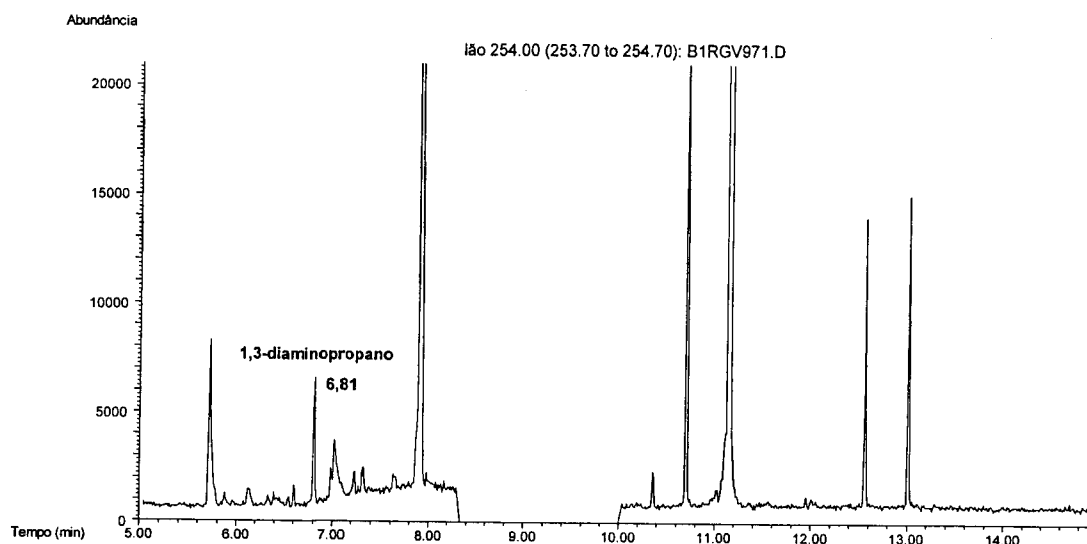
Figura 4.6. Cromatograma de massa do íon m/z 254, usado para a quantificação do 1,3-diaminopropano.
