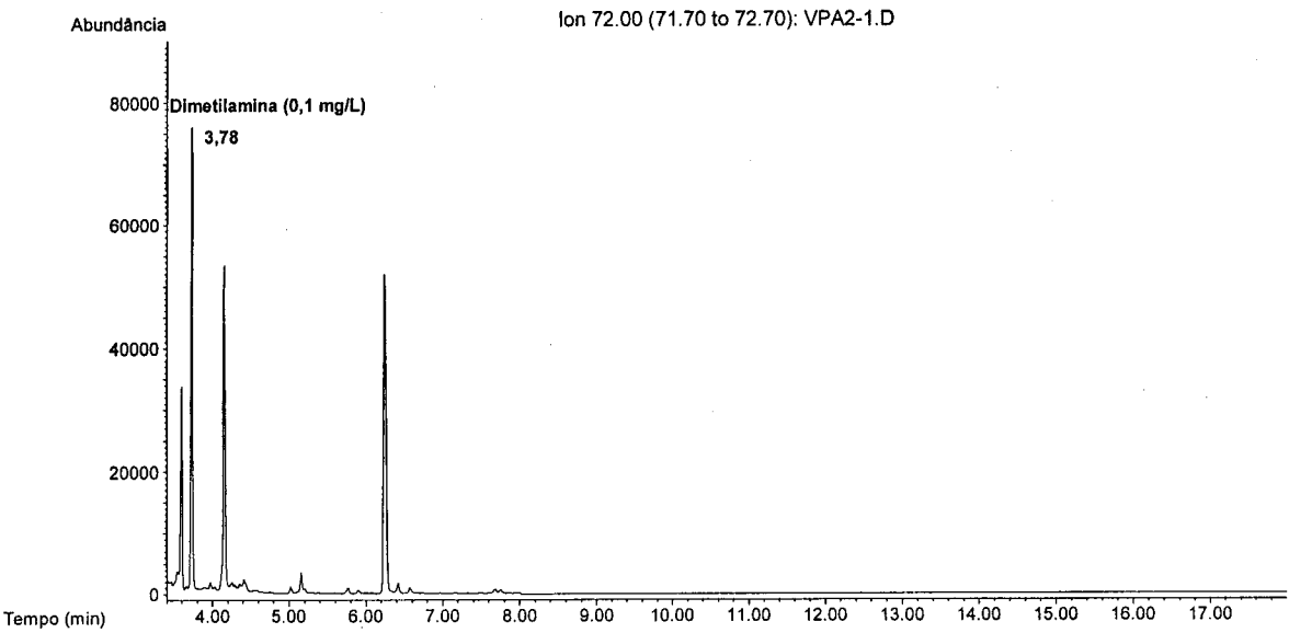
Figura 6.4. Cromatograma de massa do ião m/z 72, usado para a quantificação da dimetilamina.
