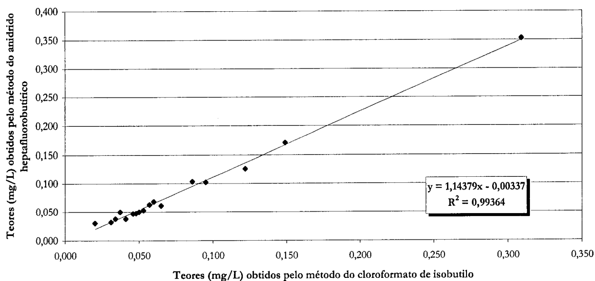
Figura 6.52. Correlação entre os resultados obtidos na determinação dos teores de tiramina em amostras de vinhos e de mostos pelo método descrito neste capítulo (derivatização com cloroformato de isobutilo) e pelo método descrito no capítulo 4 (derivatização com anidrido heptafluorobutírico).
