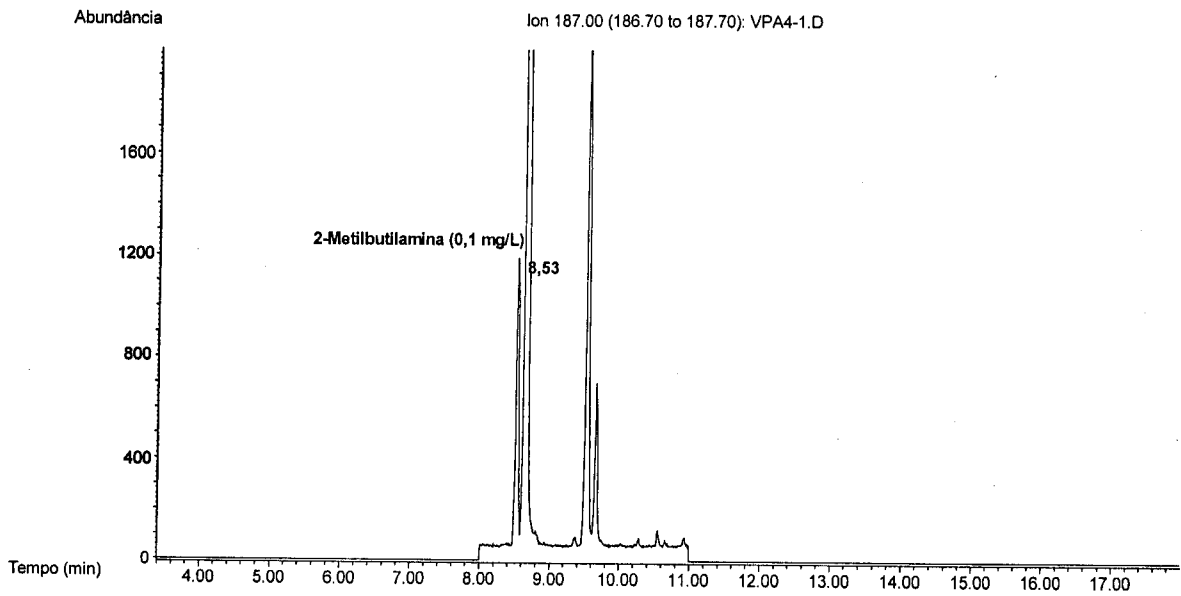
Figura 6.9. Cromatograma de massa do ião m/z 187, usado para a quantificação da 2-metilbutilamina.
