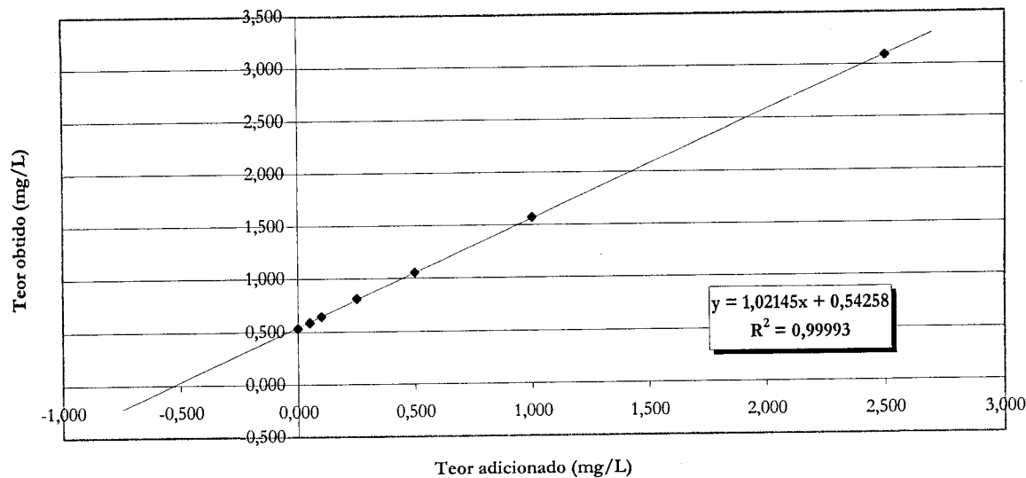
2-Feniletilamina - Recuperação (Mosto) Teor inicial: 0,535 mg/L
