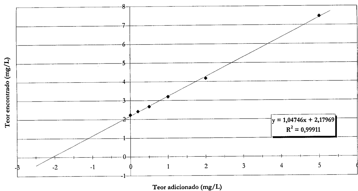
Putrescina - Recuperação (Mosto) Teor inicial: 2,239 mg/L
