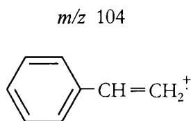
2-Feniletilamina
