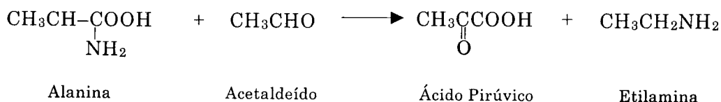
Figura 1.8. Formação da etilamina por transaminação
