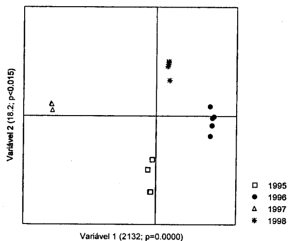
Figura 7.4. Análise discriminante de vinhos por anos. Os valores entre parêntesis correspondem ao valor próprio e à significância de cada variável.
