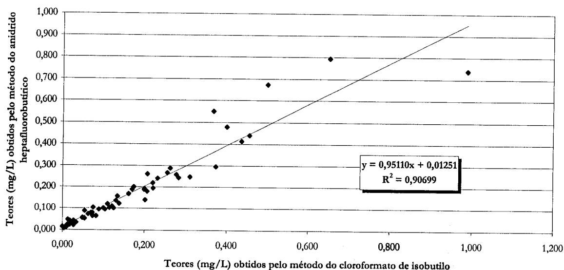
Figura 6.50. Correlação entre os resultados obtidos na determinação dos teores de cadaverina em amostras de vinhos e de mostos pelo método descrito neste capítulo (derivatização com cloroformato de isobutilo) e pelo método descrito no capítulo 4 (derivatização com anidrido heptafluorobutírico).
