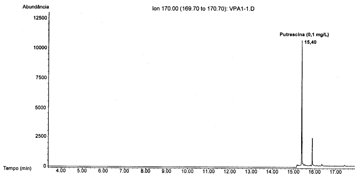
Figura 6.18. Cromatograma de massa do íon m/z 170, usado para a quantificação da putrescina (este cromatograma corresponde a uma solução de calibração com 0,100 mg/L de putrescina e 0,010 ou 0,025 mg/L das outras aminas).
