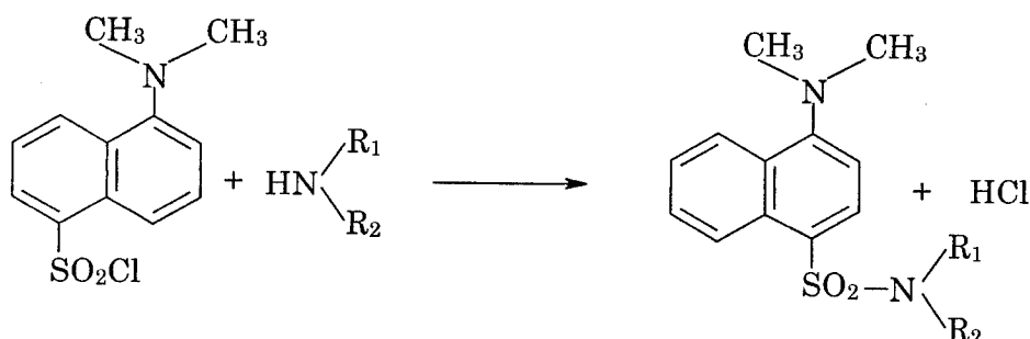
Figura 4.3. Reacção de derivatização de aminas primárias e secundárias por acção do cloreto de dansilo
