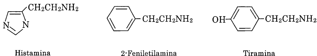
Figura 1.1. Estrutura das aminas aromáticas: histamina, 2-feniletilamina e tiramina.
