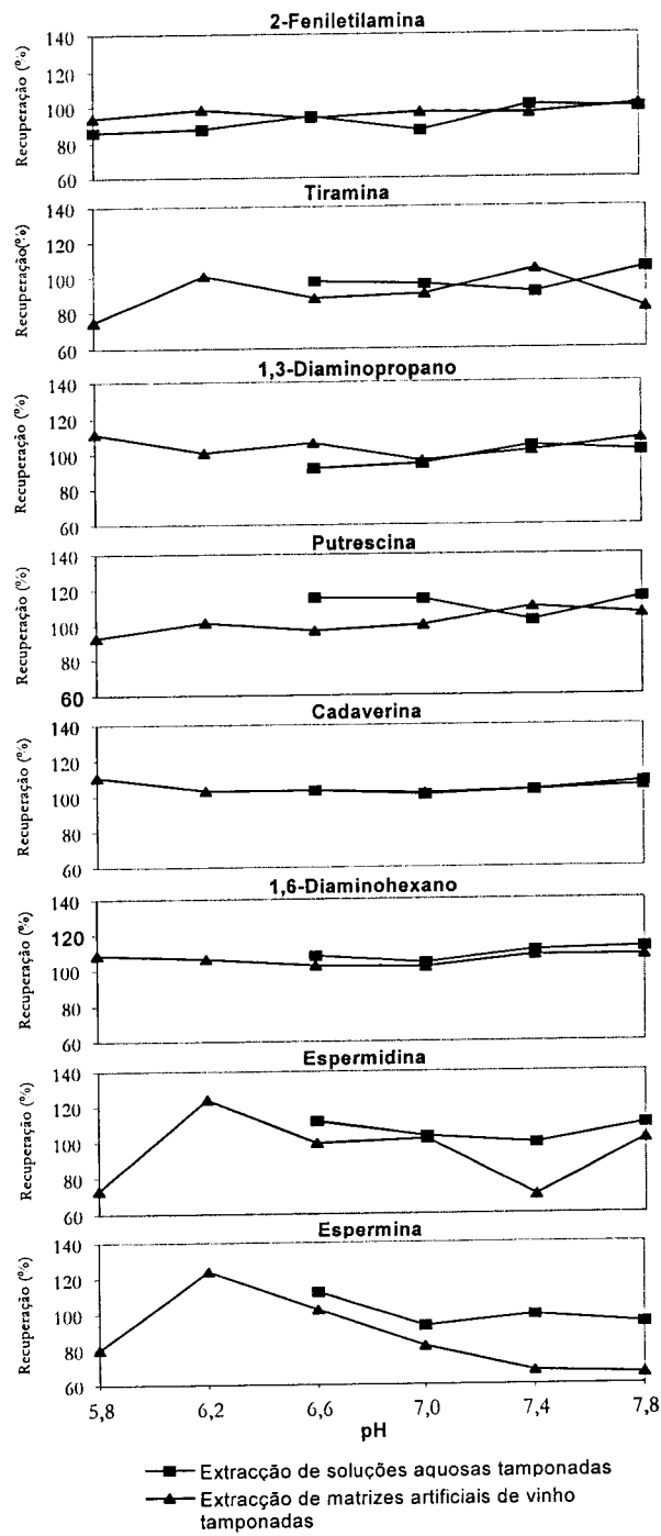
Figura 4.1. Rendimento do processo de extracção para as diferentes aminas estudadas a diferentes valores de pH
