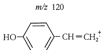
Tiramina
