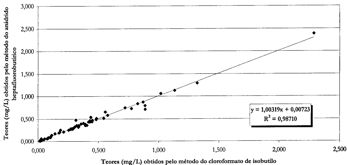
Figura 6.51. Correlação entre os resultados obtidos na determinação dos teores de 2-feniletilamina em amostras de vinhos e de mostos pelo método descrito neste capítulo (derivatização com cloroformato de isobutilo) e pelo método descrito no capítulo 4 (derivatização com anidrido heptafluorobutírico).
