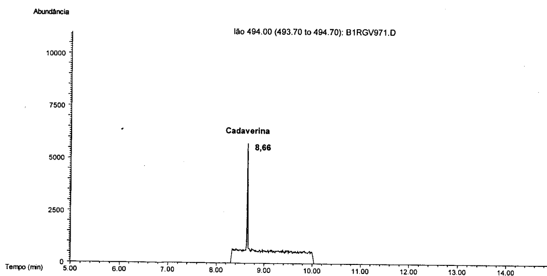
Figura 4.7. Cromatograma de massa do íon m/z 494, usado para a quantificação da cadaverina.
