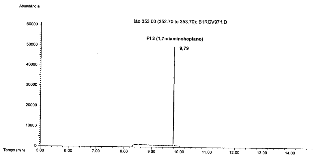
Figura 4.11. Cromatograma de massa do ião m/z 353, usado para a "quantificação" do 1,7-diaminoheptano (padrão interno 3).
