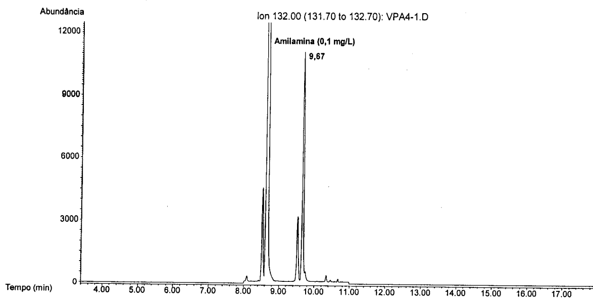
Figura 6.13. Cromatograma de massa do íon m/z 132, usado para a quantificação da amilamina.
