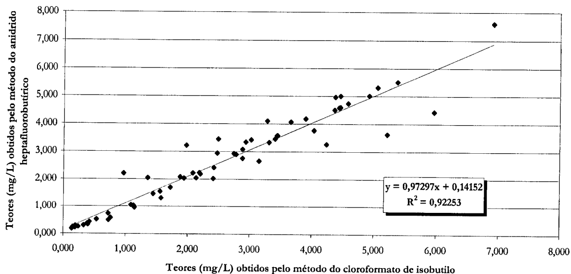
Figura 6.49. Correlação entre os resultados obtidos na determinação dos teores de putrescina em amostras de vinhos e de mostos pelo método descrito neste capítulo (derivatização com cloroformato de isobutilo) e pelo método descrito no capítulo 4 (derivatização com anidrido heptafluorobutírico).
