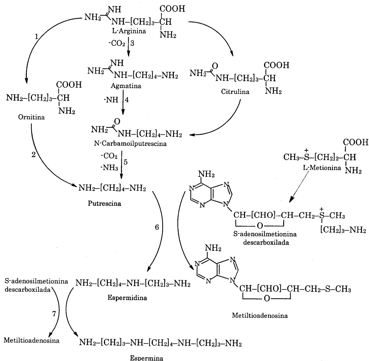
Figura 1.7. Vias metabólicas que regulam a produção de putrescina, espermidina e espermina. (1-arginase; 2-ornitina-descarboxilase; 3-arginina-descarboxilase; 4-agmatina-iminohidrolase; 5-putrescina-carbamoil-transferase; 6-espermidina-sintase; 7-espermina-sintase)*.
