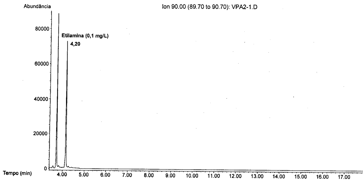
Figura 6.5. Cromatograma de massa do ião m/z 90, usado para a quantificação da etilamina.
