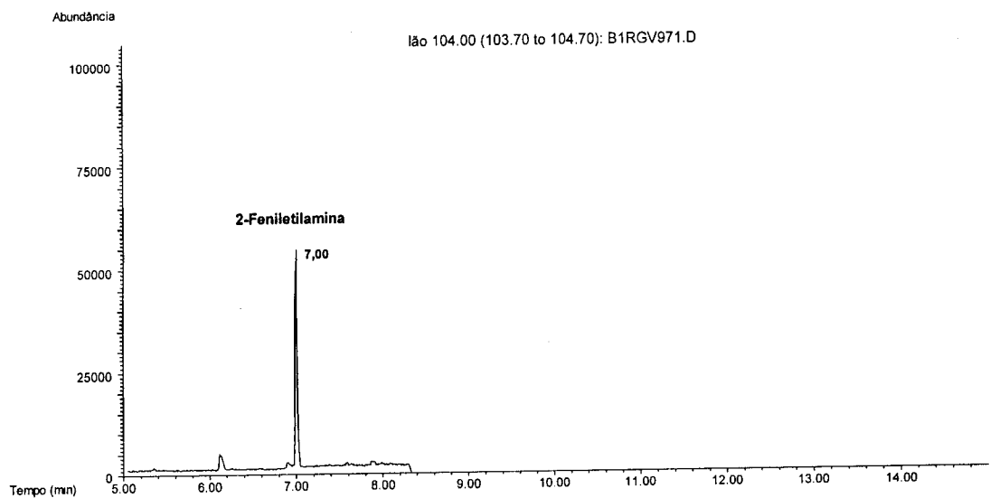
Figura 4.4. Cromatograma de massa do ião m/z 104, usado para a quantificação da 2-feniletilamina.
