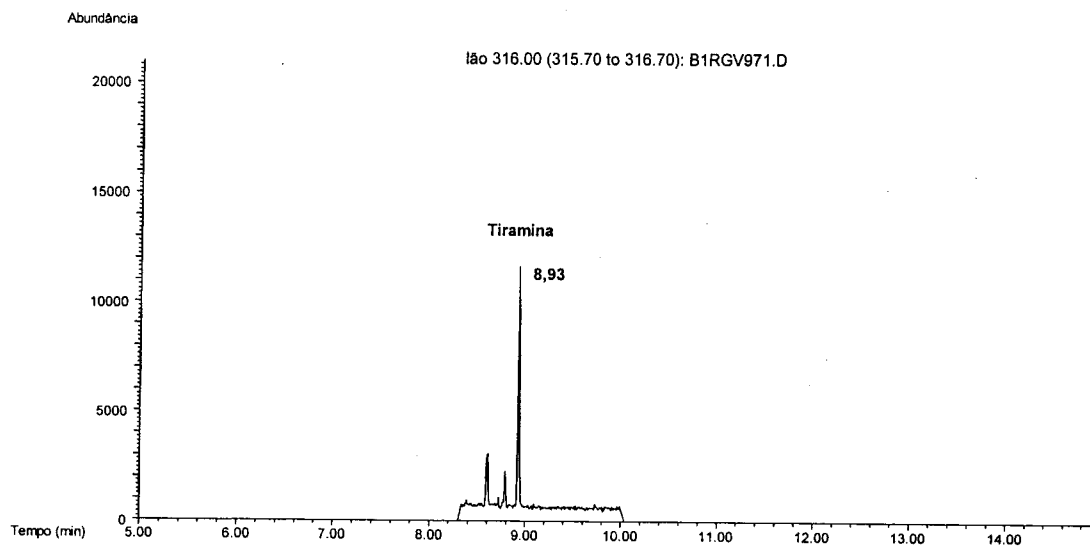
Figura 4.10. Cromatograma de massa do ião m/z 316, usado para a quantificação da tiramina.
