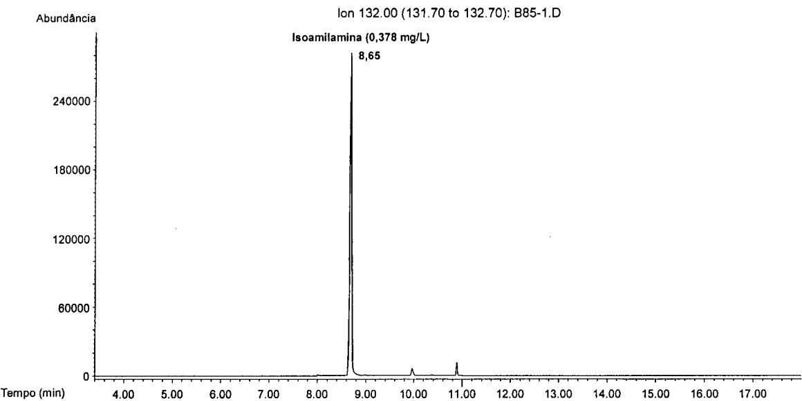
Figura 6.34. Cromatograma de massa do íon m/z 132, usado para a quantificação da isoamilamina.
