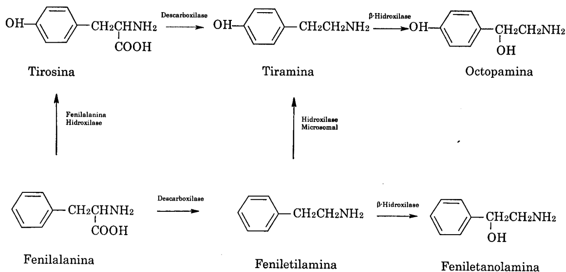
Figura 1.4. Inter-relações metabólicas entre a 2-feniletilamina e a tiramina.
