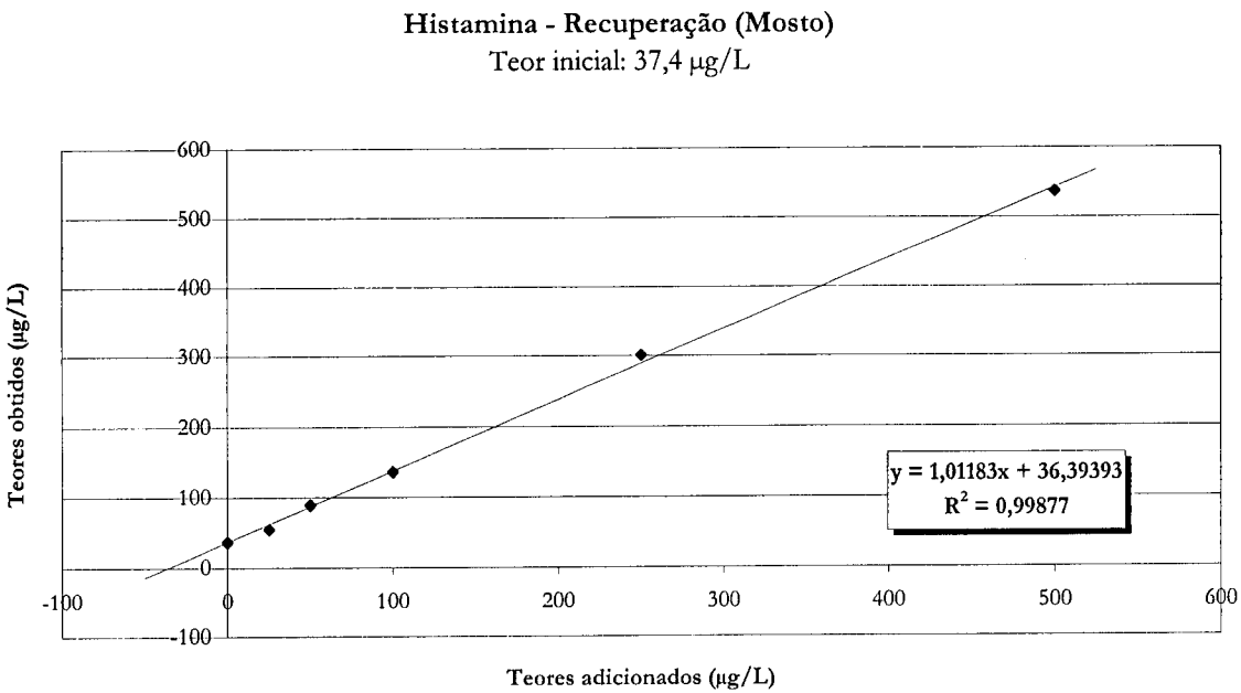
Figura 5.5. Curva de recuperação obtida pela adição de quantidades conhecidas de histamina a uma amostra de mosto.
