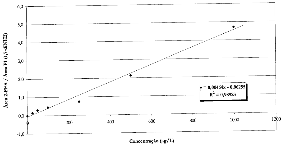
2-Feniletilamina - Curva de Calibração (2)
