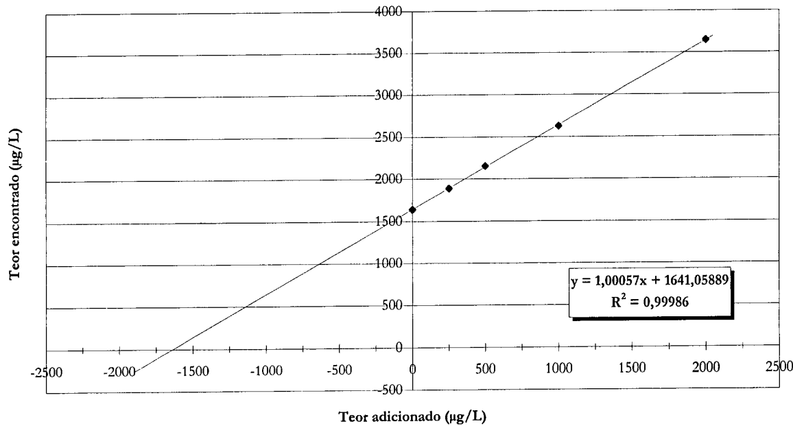
Putrescina - Recuperação (Vinho do Porto) Teor inicial: 1,639 mg/L
