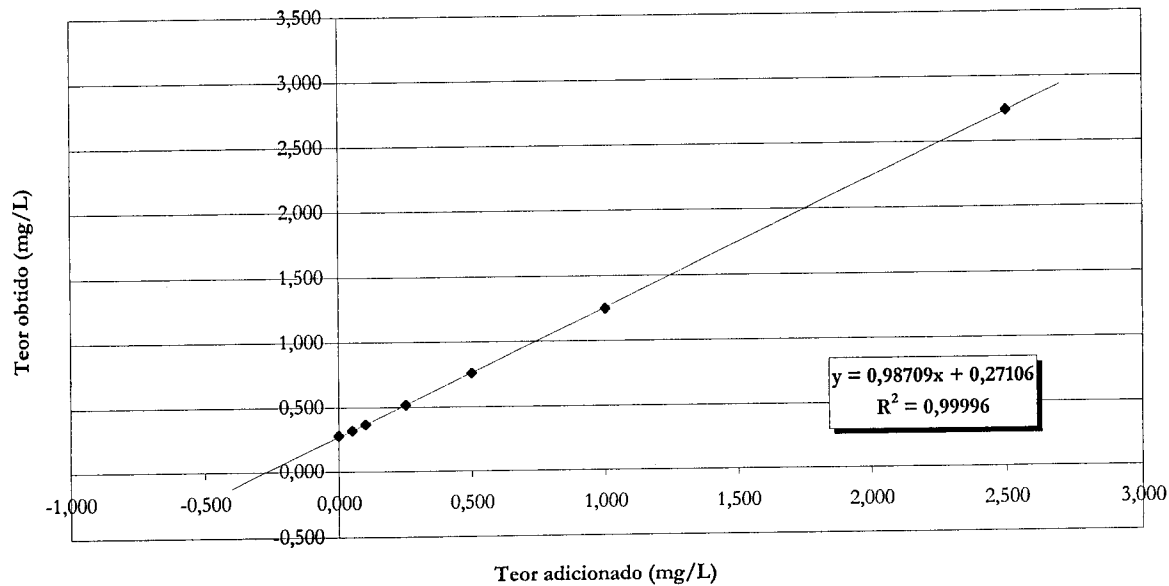
2-Feniletilamina - Recuperação (Vinho do Porto) Teor inicial: 0,281 mg/L
