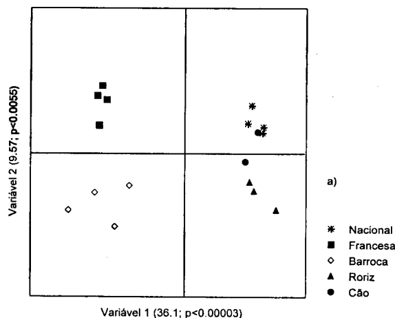
Figura 7.3. Análise discriminante de vinhos por castas. Os valores entre parêntesis correspondem ao valor próprio e à significância de cada variável.
