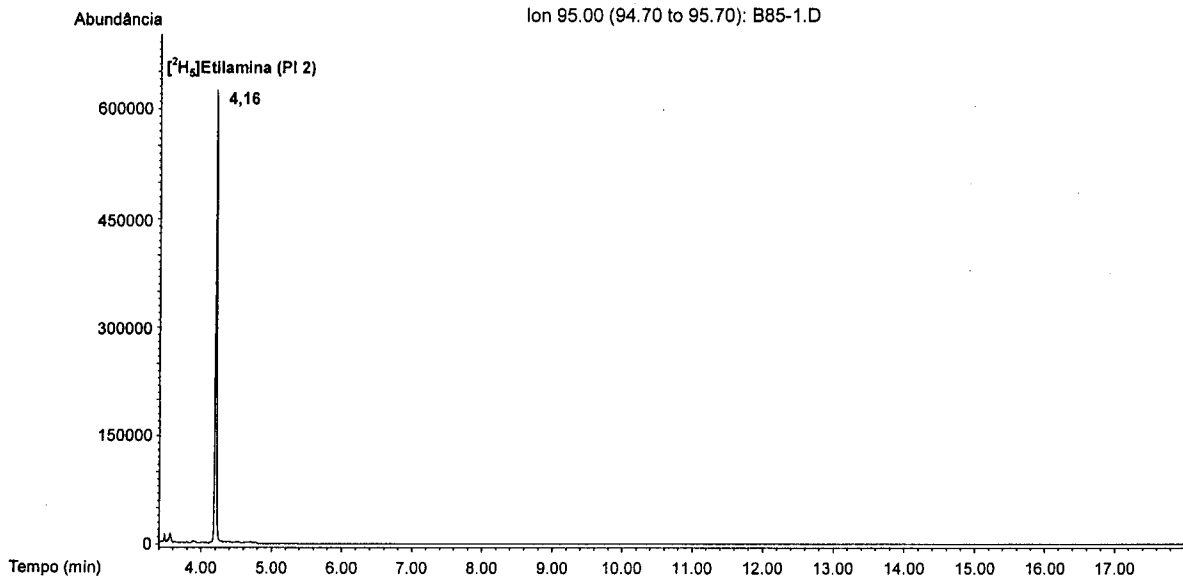
Figura 6.40. Cromatograma de massa do íon m/z 95, usado para a "quantificação" da [^2\text{H}_3] etilamina (PI 2).
