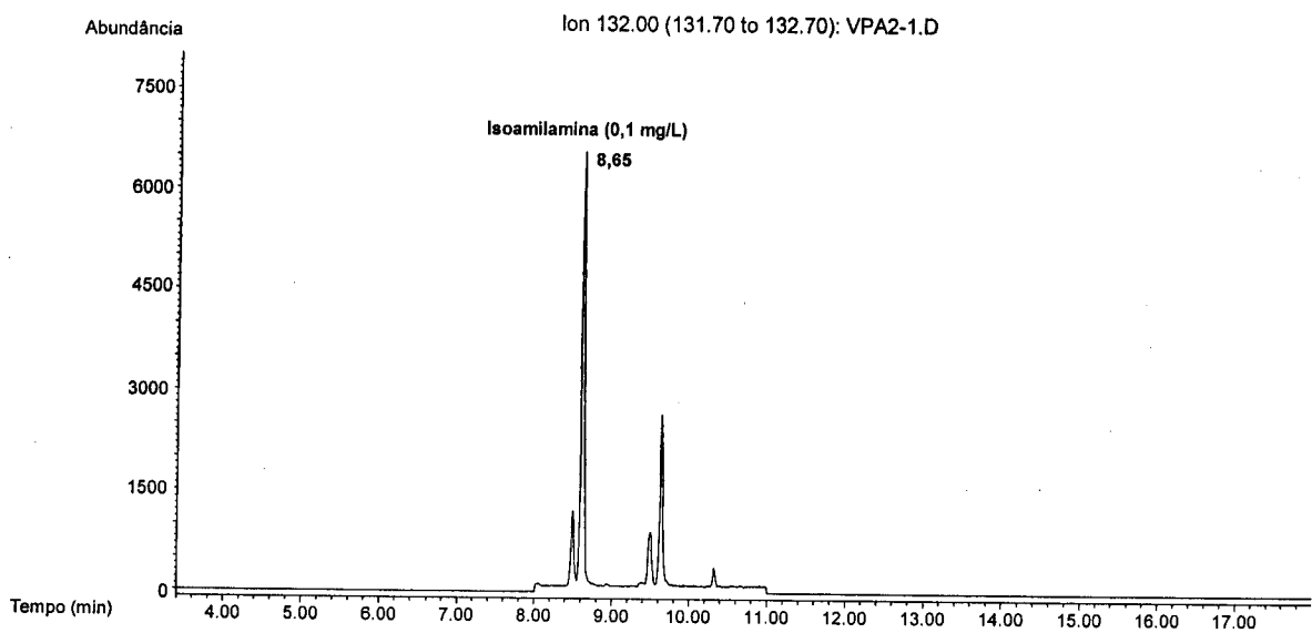
Figura 6.10. Cromatograma de massa do ião m/z 132, usado para a quantificação da isoamilamina.
