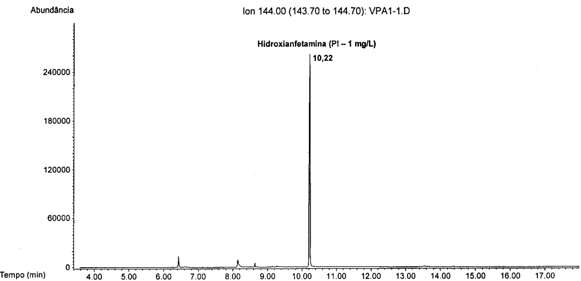
Figura 6.28. Cromatograma de massa do ião m/z 144 (correspondente à mesma solução de calibração da figura anterior) usado para a "quantificação" da hidroxianfetamina (PI).
