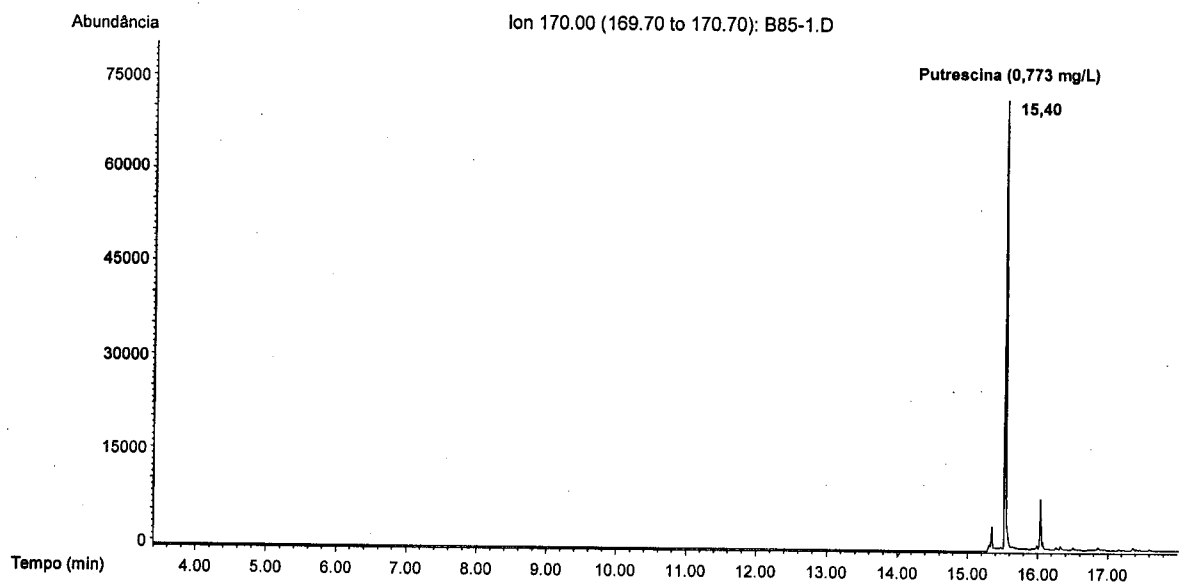
Figura 6.37. Cromatograma de massa do íon m/z 170, usado para a quantificação da putrescina.
