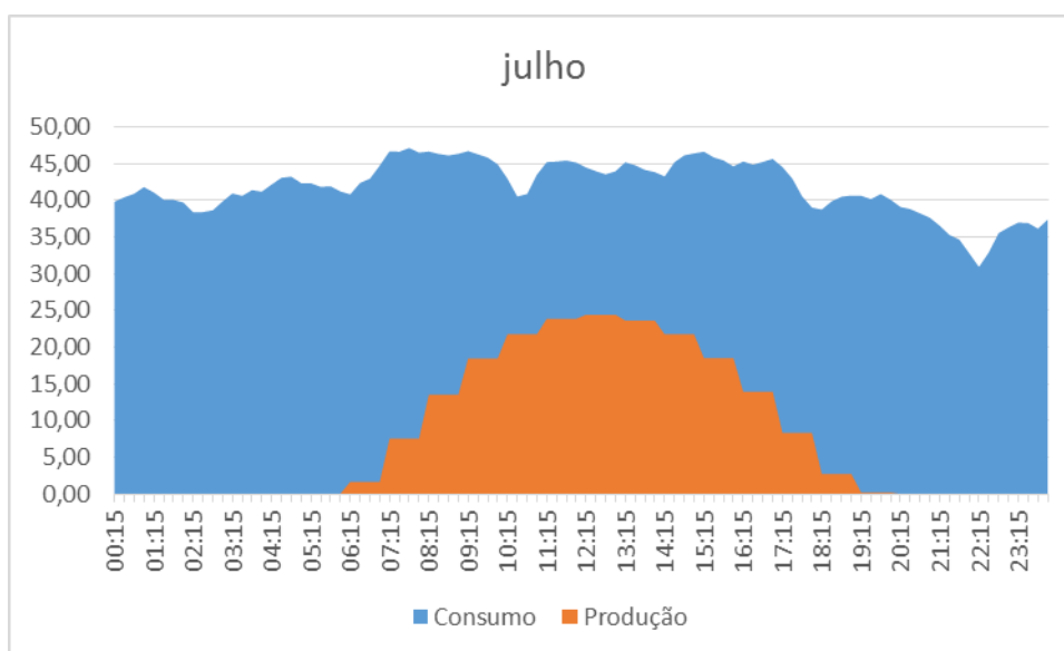
Figura 5.14 - Gráfico de consumo e produção média diária em julho, em kWh a cada período de 15 min
