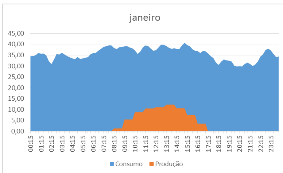
Figura 5.8 - Gráfico de consumo e produção média diária em janeiro, em kWh a cada período de 15 min
