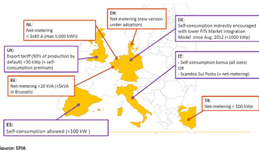
Figura 4.12 - Esquemas de net-metering e autoconsumo na Europa, relativos ao ano 2013 [34]
