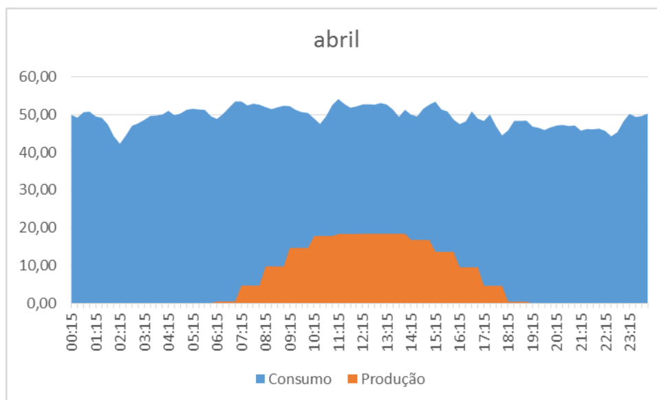
Figura 5.11 - Gráfico de consumo e produção média diária em abril, em kWh a cada período de 15 min
