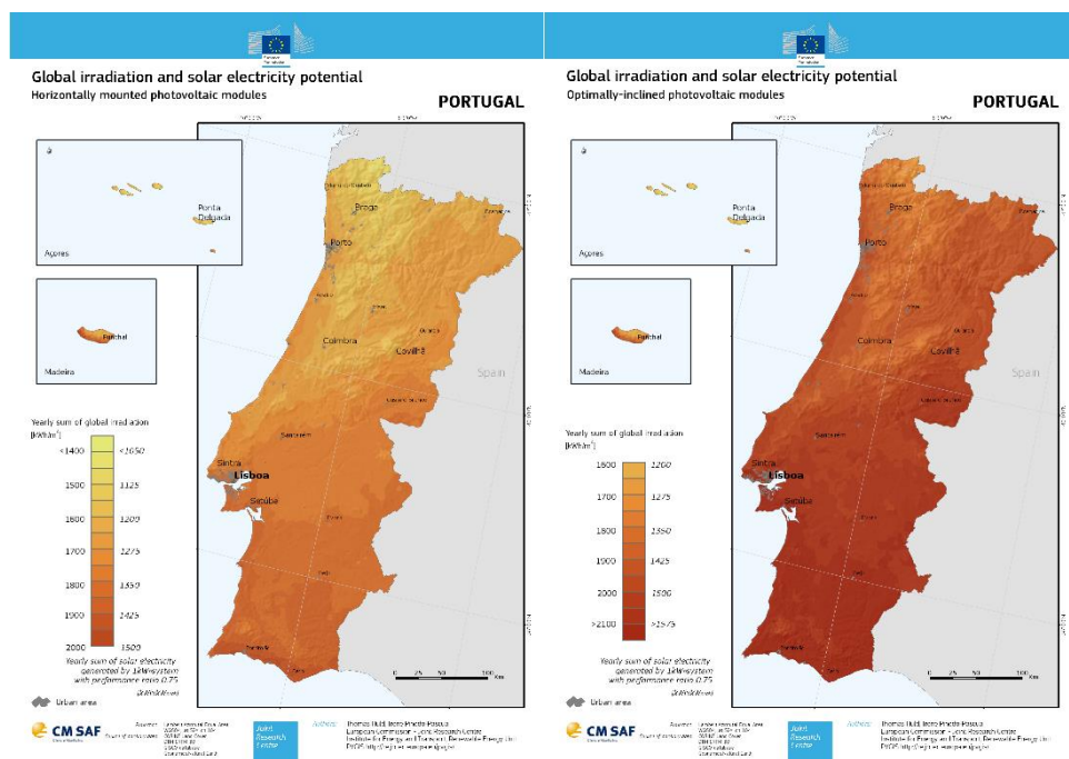
Figura 2.2 - Irradiação global para inclinação horizontal (esq.) e ótima (dir.) [2]
