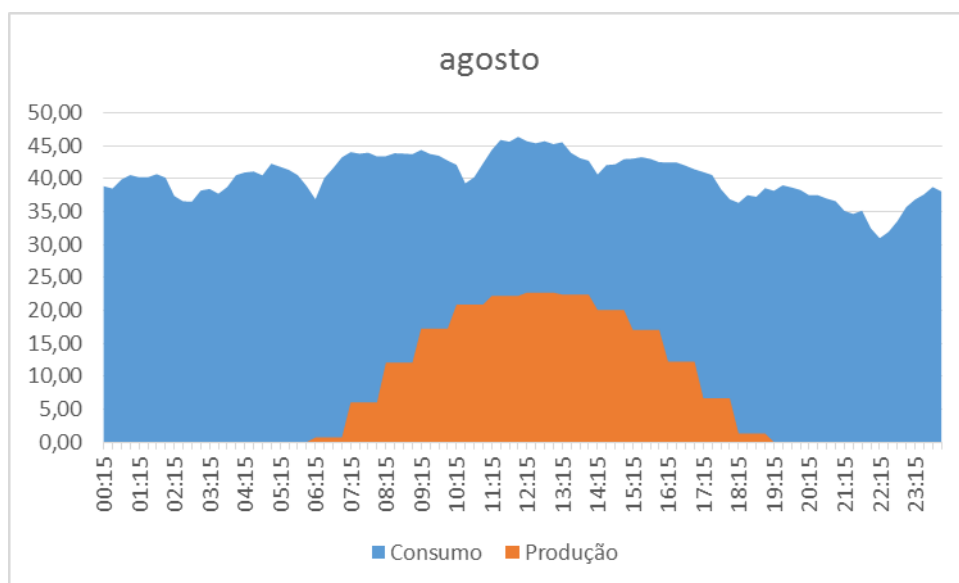
Figura 5.15 - Gráfico de consumo e produção média diária em agosto, em kWh a cada período de 15 min
