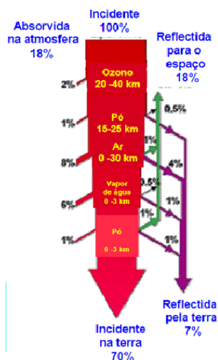
Figura 2.1 - Várias componentes da irradiação solar incidente [3]
