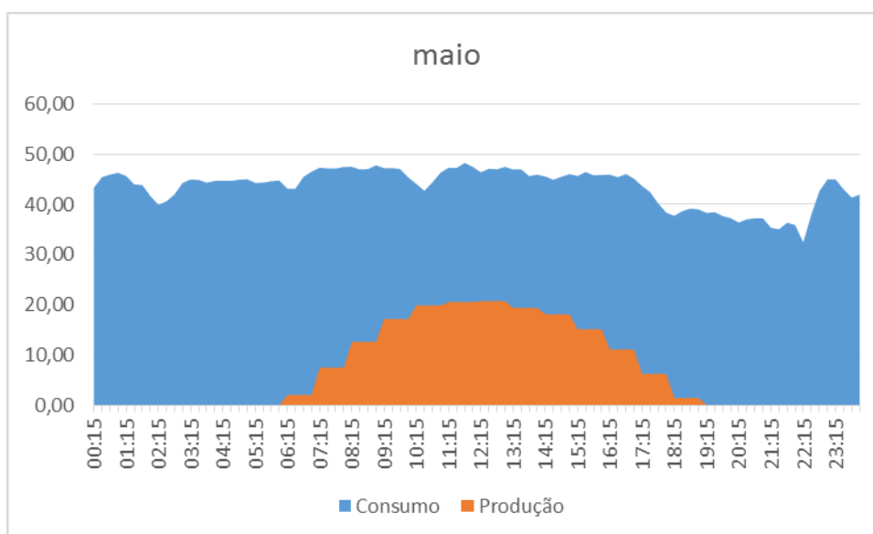
Figura 5.12 - Gráfico de consumo e produção média diária em maio, em kWh a cada período de 15 min
