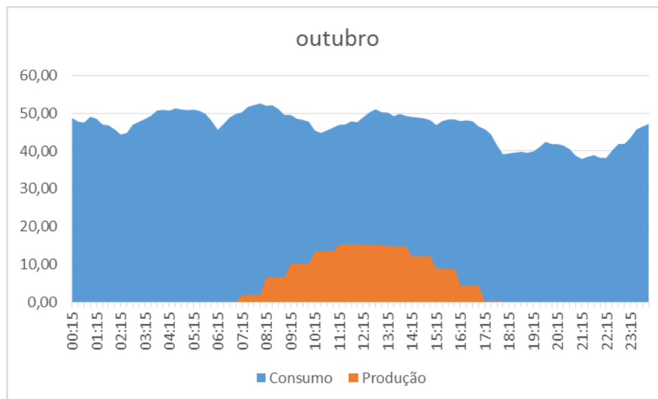
Figura 5.17 - Gráfico de consumo e produção média diária em outubro, em kWh a cada período de 15 min
