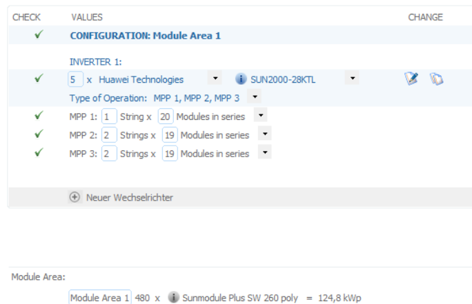
Figura 5.6 - PVSOL: Escolha e configuração do inversor para a instalação
