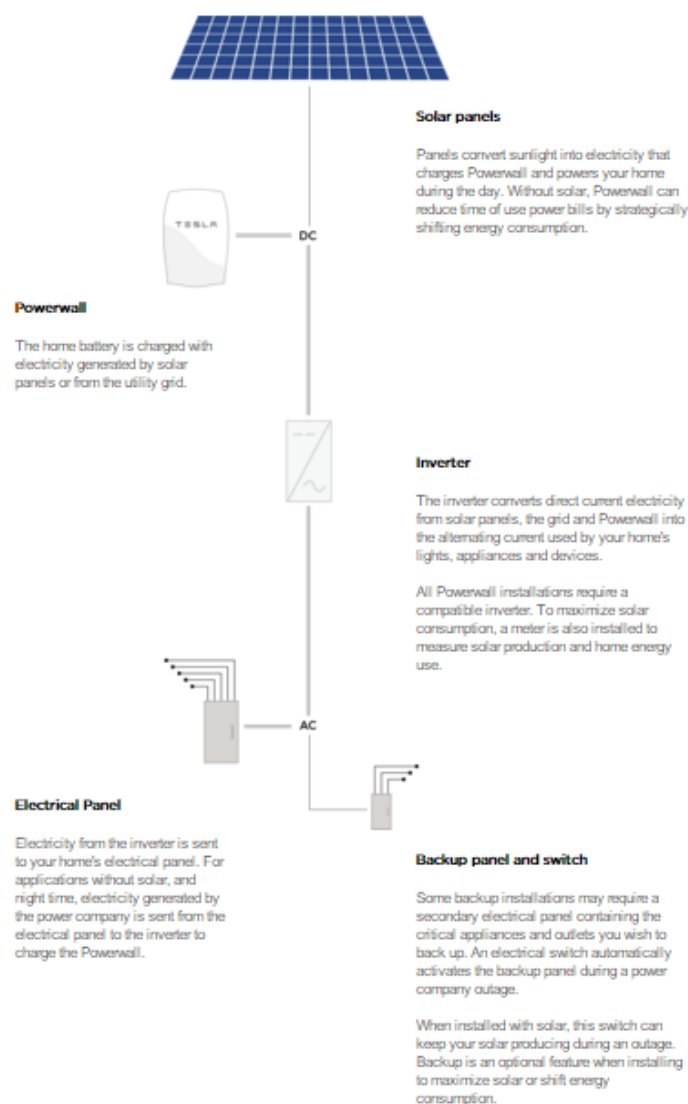
Figura 3.17 - Esquema de funcionamento da bateria Tesla Powerwall [21]
