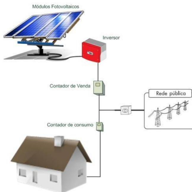
Figura 3.18 - Sistema fotovoltaico ligado à rede [22]
