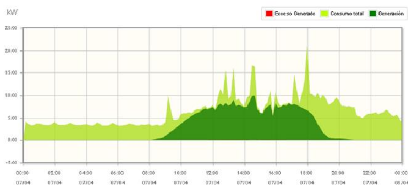
Figura 4.9 - Consumo Total (kWh), produção fotovoltaica (kWh) e preço da energia elétrica/hora (€/kWh) [30]
