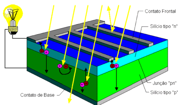
Figura 3.1 - Esquema exemplificativo do efeito fotovoltaico [6]
