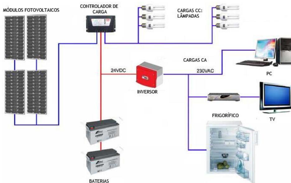
Figura 3.19 - Sistema fotovoltaico isolado [22]
