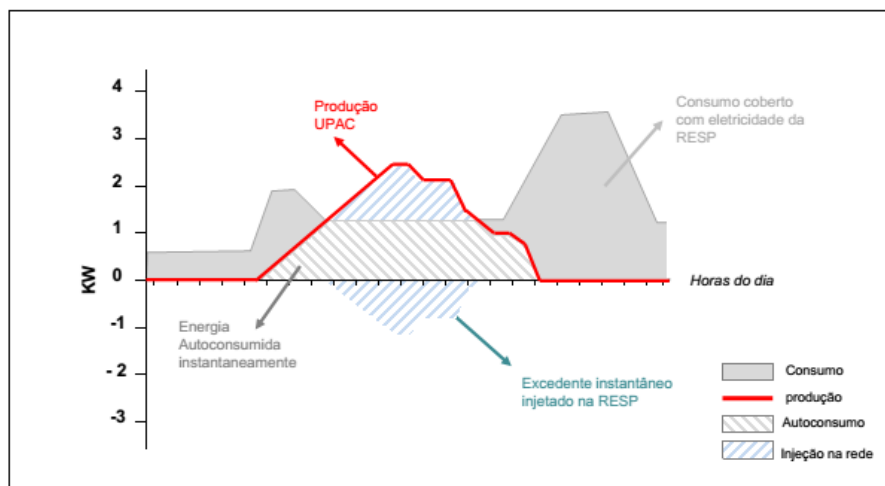
Figura 4.6 - Diagrama de produção e consumo de um consumidor doméstico, sem baterias de armazenamento [28]
