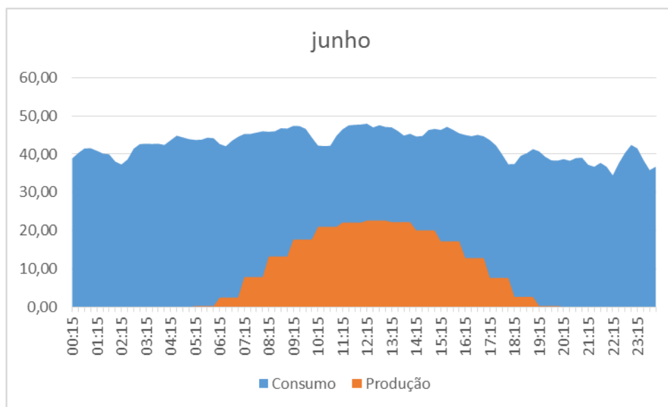
Figura 5.13 - Gráfico de consumo e produção média diária em junho, em kWh a cada período de 15 min
