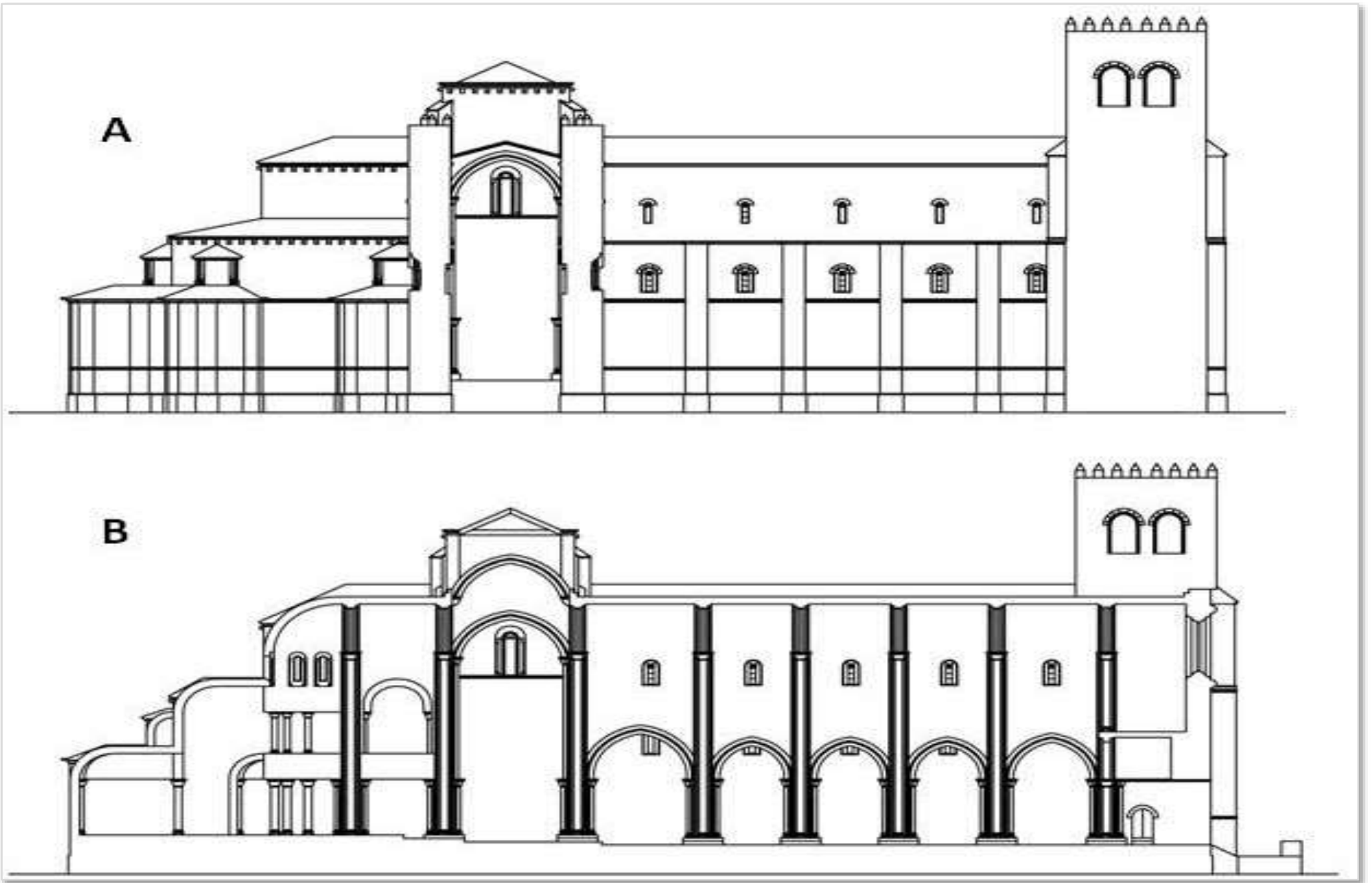
A - Corte lateral do transepto da Sé do Porto; B - Corte lateral da nave central da Sé do Porto.
