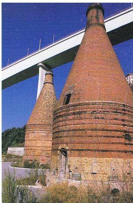
Figura 3079: Forno da Fábrica de Massarelos.
