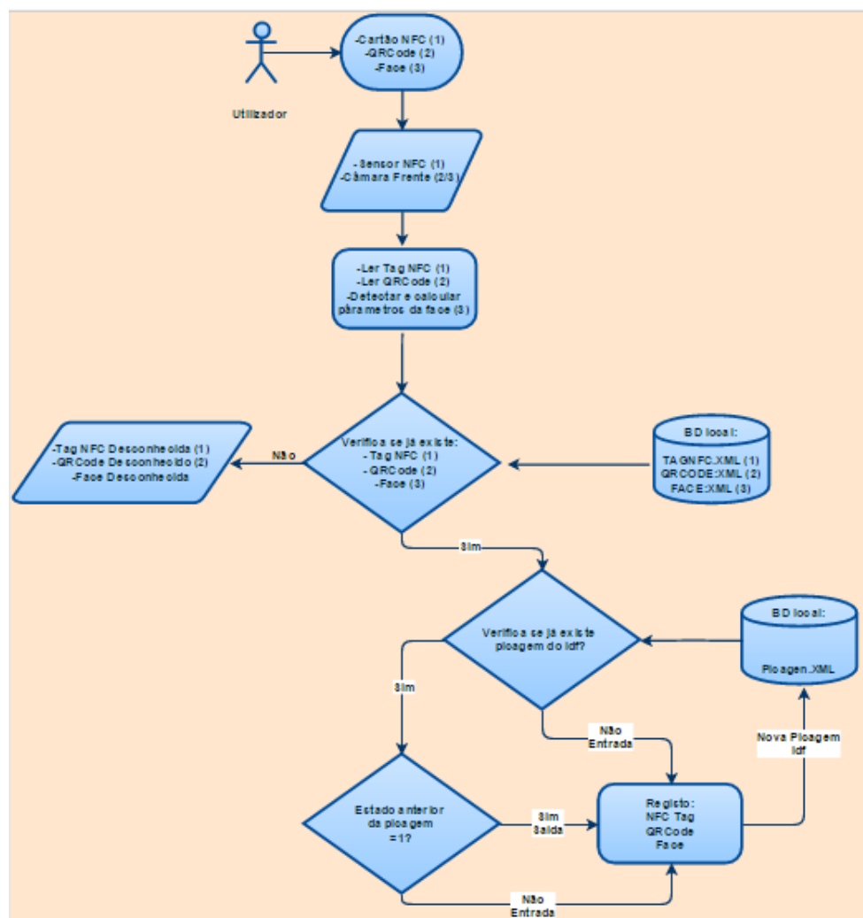
Figura 3.5: Diagrama de fluxo de dados do reconhecimento (entradas/saídas)
