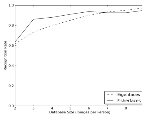
Figura 2.7: Eficácia dos métodos por número de imagens
