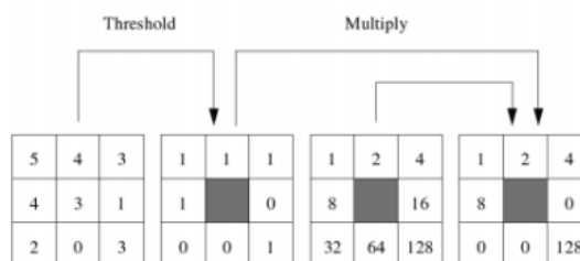
Figura 2.13: PBLH de cada pixel
