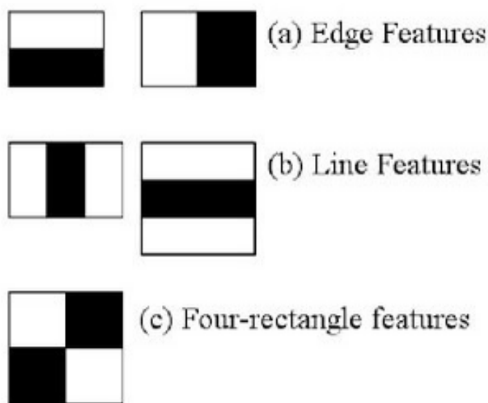
Figura 3.10: Características haar
