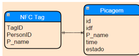
Figura 3.32: Entidade-Relação NFC-Picagem
