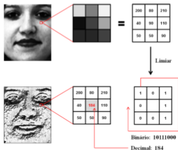
Figura 2.14: Descritores PBLH
