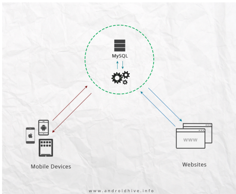
Figura 3.46: Arquitetura REST
