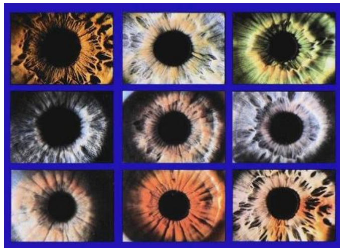
Figura 2.16: Exemplos Irís
