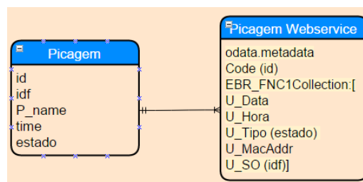
Figura 3.45: Entidade-Relação picagem.XML-Picagem.JSON
