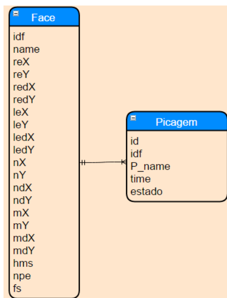
Figura 3.23: Entidade-Relação Face-Picagem
