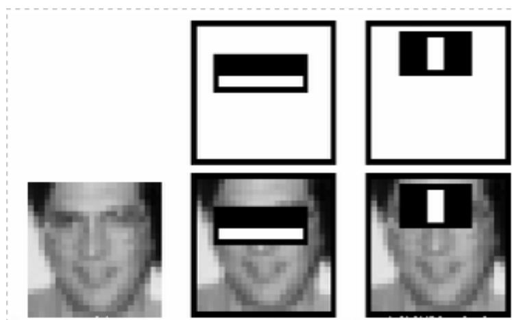
Figura 3.11: Características Faciais
