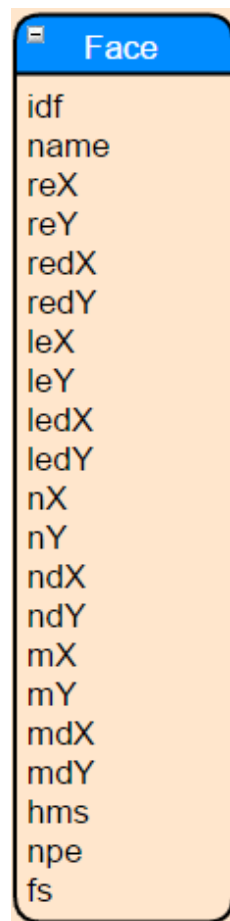
Figura 3.22: Entidade Face
