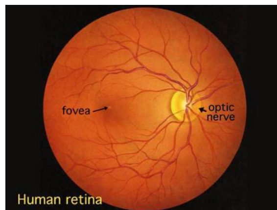
Figura 2.15: Exemplo Retina
