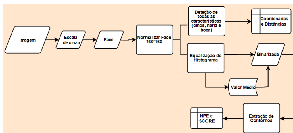
Figura 3.21: Método Reconhecimento Completo
