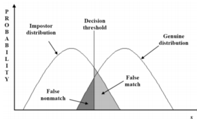
Figura 2.26: Taxas de erro em Sistemas Biométricos
