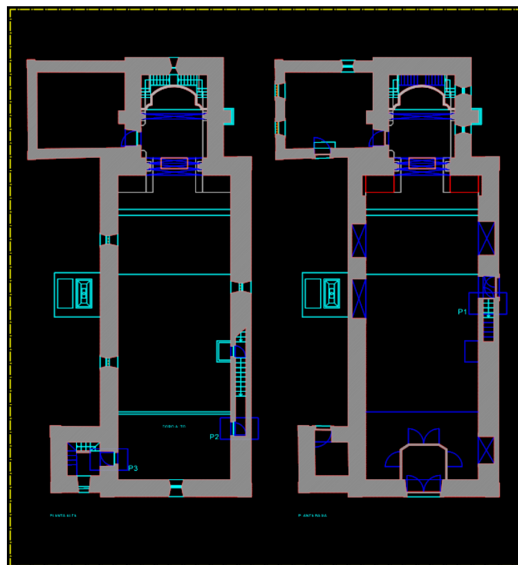
Planta da localização das portas
