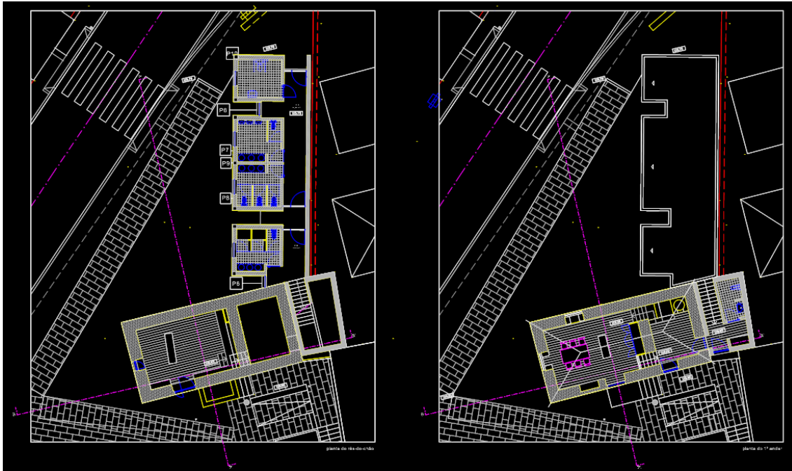
Planta de rés-do-chão
