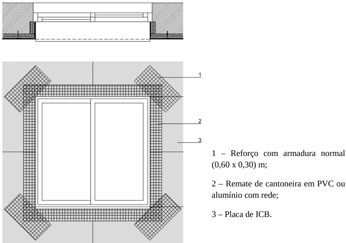
Figura 3.18 – Reforço com armadura normal nos vértices dos vãos da fachada.
