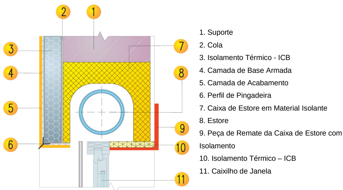
Figura 3.25 – Remate em padieira de janelas.
