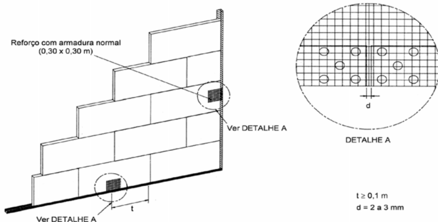
Figura 3.15 – Reforço das juntas entre perfis de arranque e laterais.
