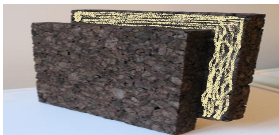
Figura 4.6 – Distribuição da cola na superfície que vai de encontro à face de outra peça.
