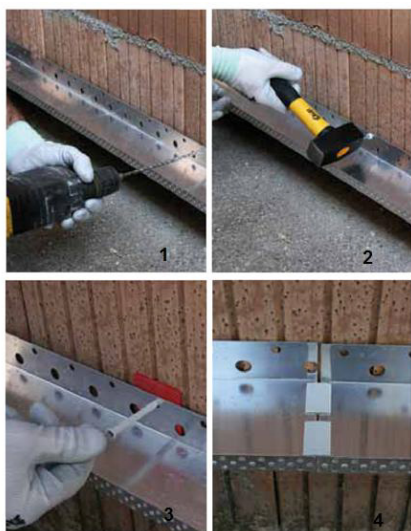
Figura 3.13 – Montagem dos perfis de arranque.
