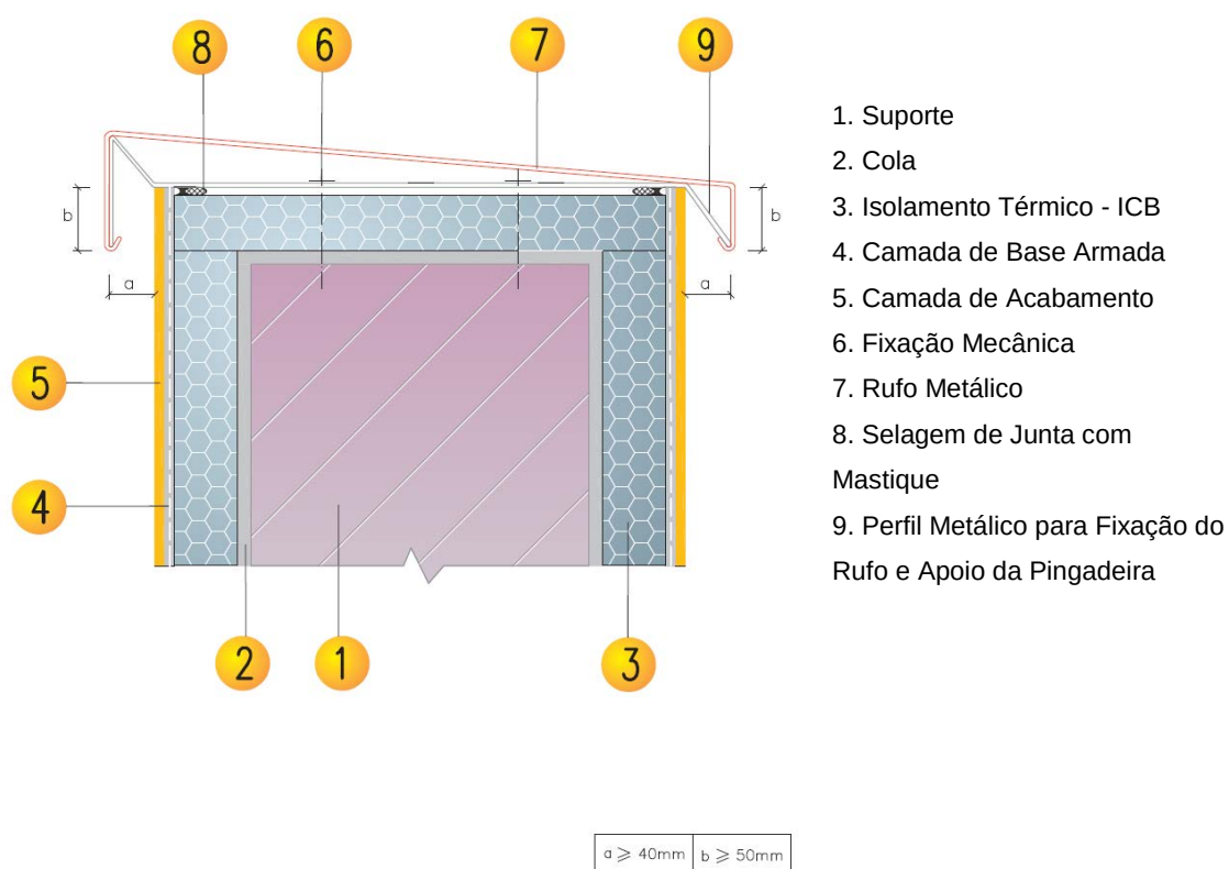
Figura 3.26 - Remate superior de parede (Platibanda).
