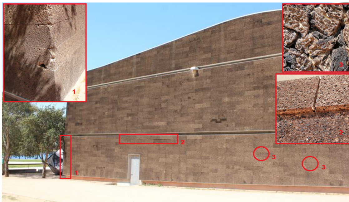
Figura 5.9 – 1- Extremidade deteriorada; 2 – blocos destacados; 3 – ressequimento de tonalidade escura, fachada sul.
