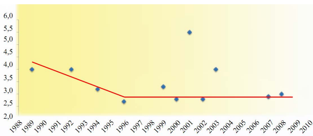
Figura 3.38 – Número médio de anomalias verificadas por fachada, segundo o ano de aplicação do sistema.
