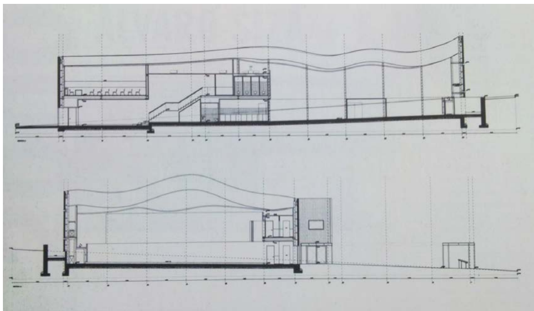
Figura 5.3– Corte lateral sul e corte lateral este do Pavilhão Centro de Portugal.
