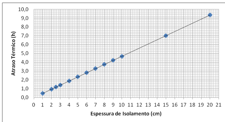
Figura 2.10 – Evolução do atraso térmico com o aumento de espessuras de isolamento (ICB).
