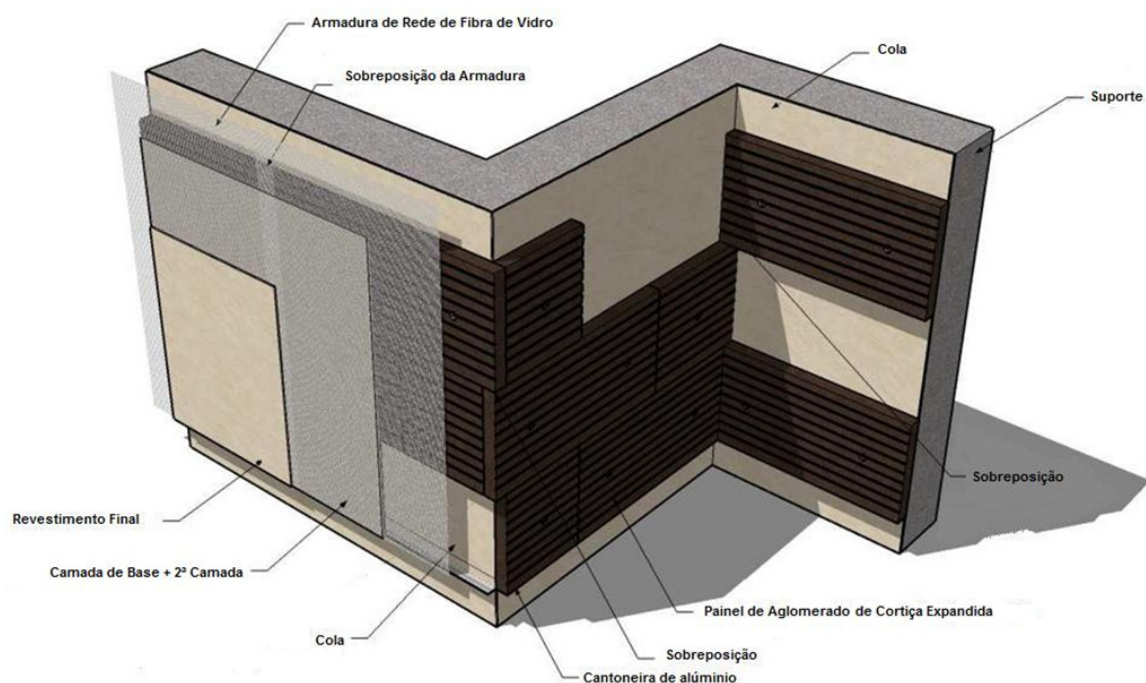
Figura 3.21 – Composição Esquemática de um ETICS – ICB, constituído por um Reboco Armado.
