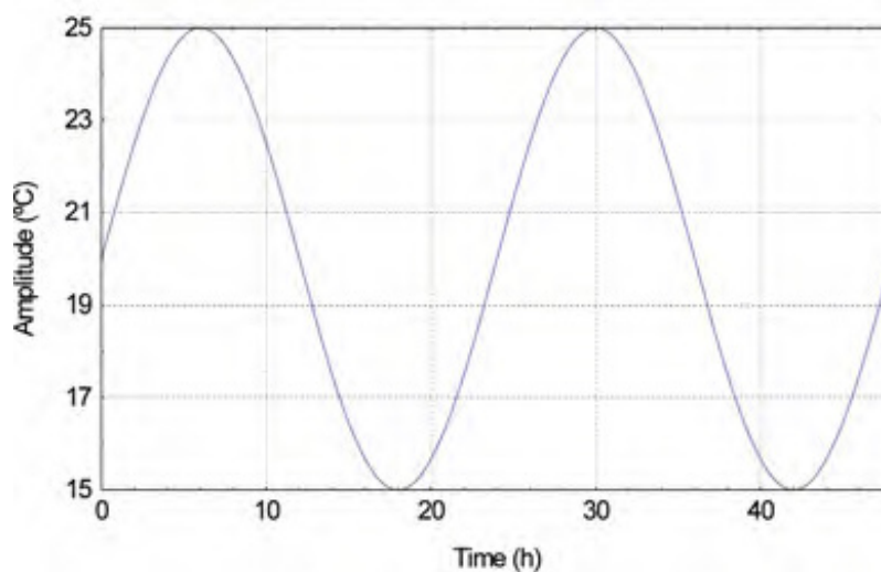
Figura 2.11 – Evolução da variação de temperatura na superfície exterior do sistema ao longo de 50 horas.
