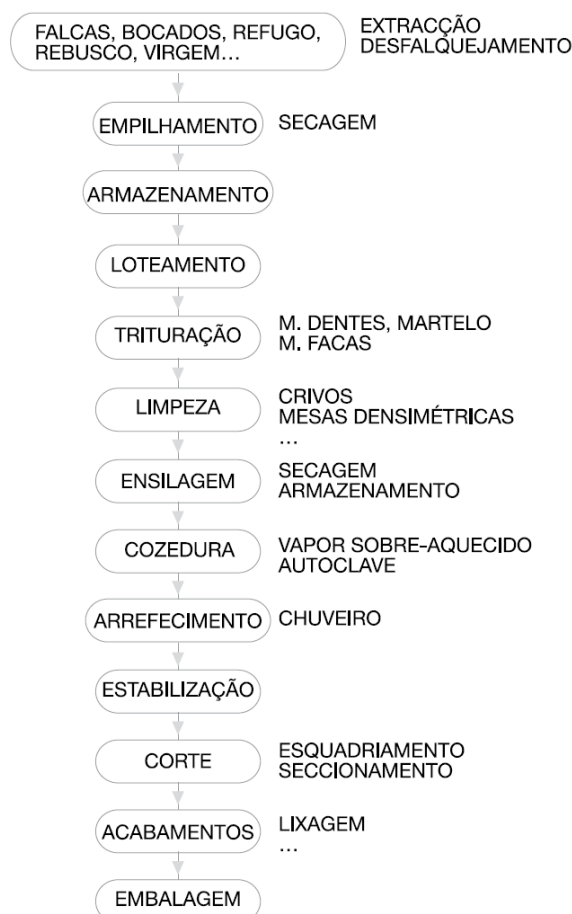
Figura 2.8 – Esquema de fabrico do ICB.
