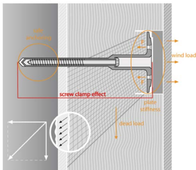
Figura 3.7 – Decomposição de esforços numa ancoragem.
