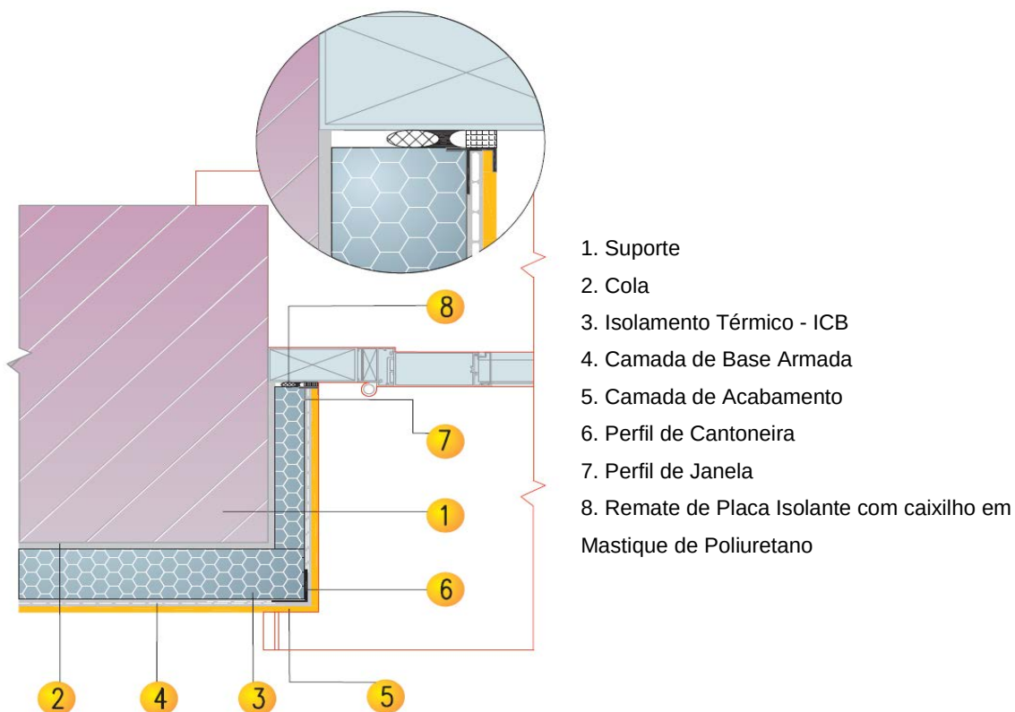
Figura 3.24 – Remate em ombreira de janelas.
