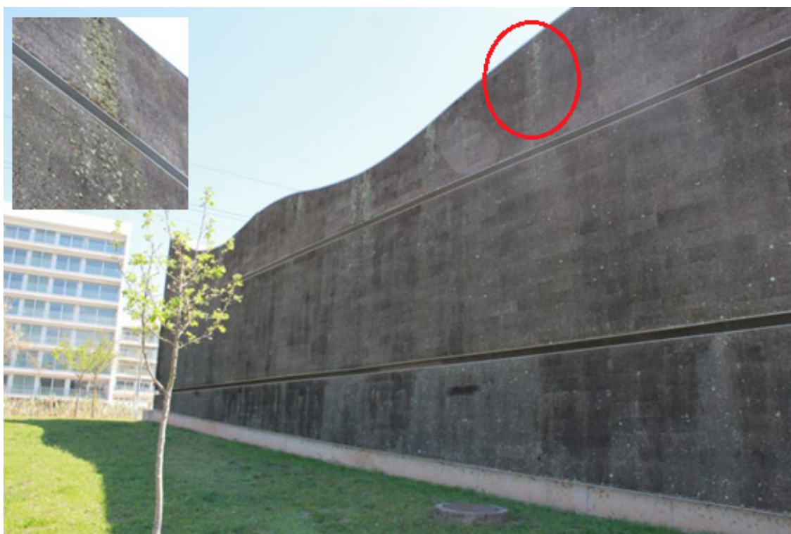
Figura 5.5 – Escorrências e distribuição de líquenes fachada norte.
