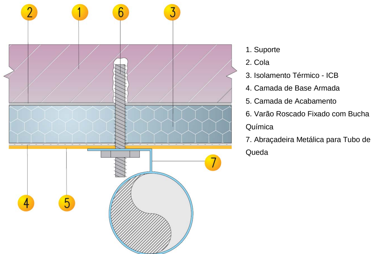
Figura 3.29 – Fixação de elementos na fachada (tubo de queda).
