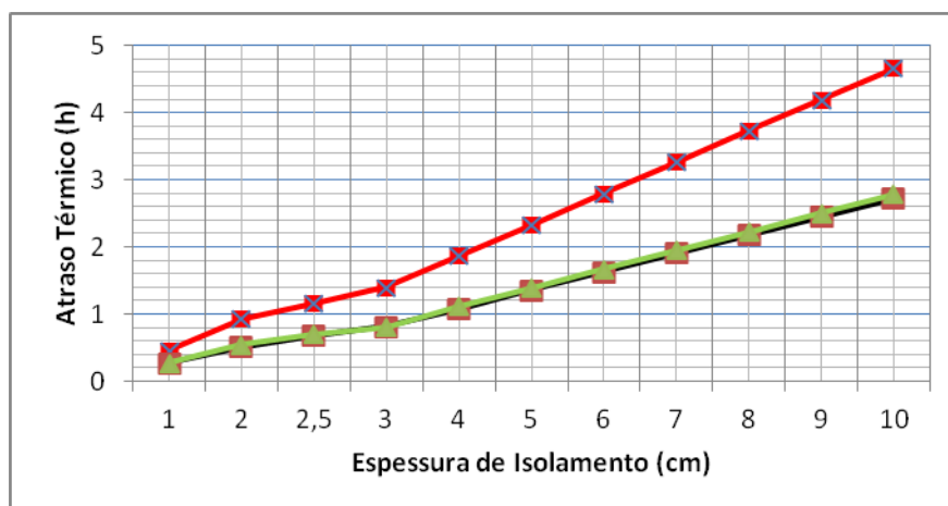
Figura 2.13 – Evolução do atraso térmico com o aumento de espessuras de isolamento (ICB, XPS, MW).
