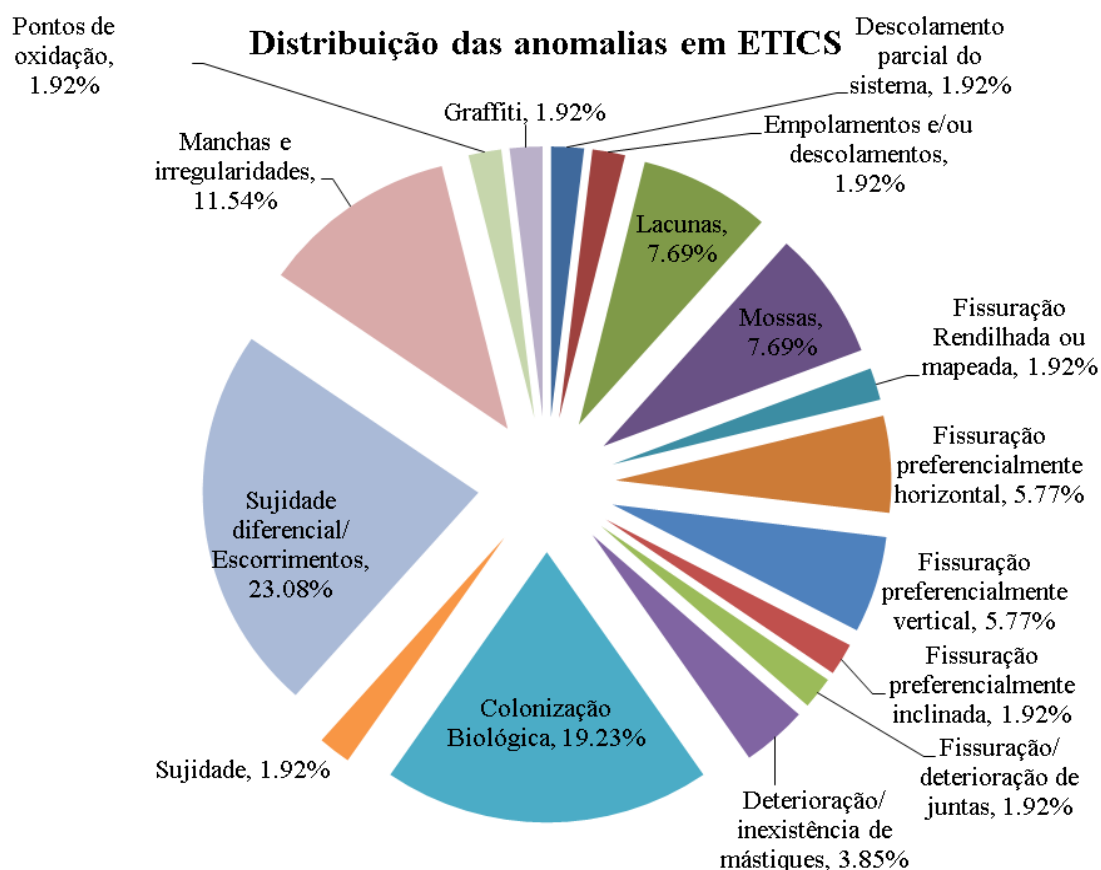
Figura 3.30 – Distribuição das patologias associadas ao sistema ETICS.
