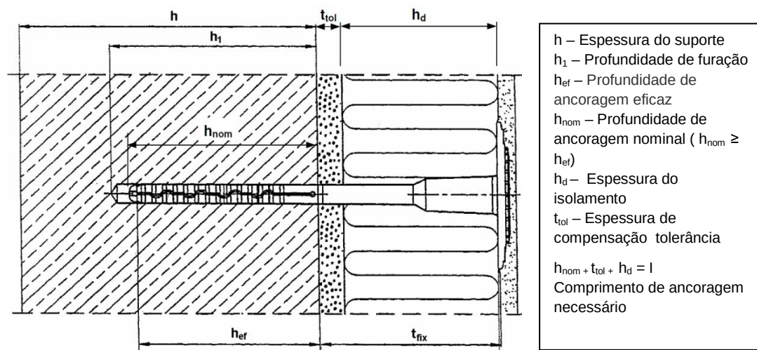
Figura 3.10 – Fixação de uma ancoragem.
