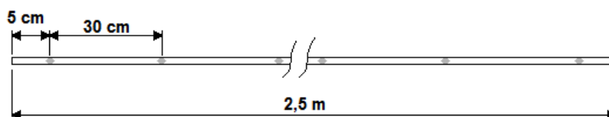
Figura 3.14 – Afastamentos das fixações.
