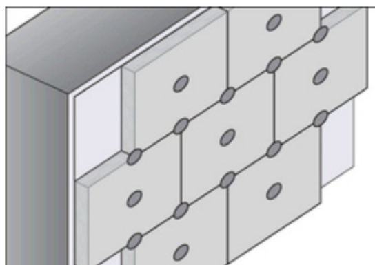
Figura 3.9 – Fixação adicional das placas de isolamento.
