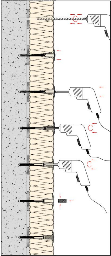
Figura 3.19 – Montagem de uma ancoragem.
