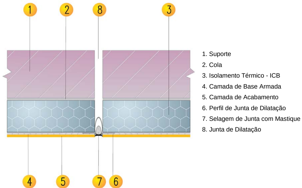
Figura 3.27 – Remate em junta de dilatação.
