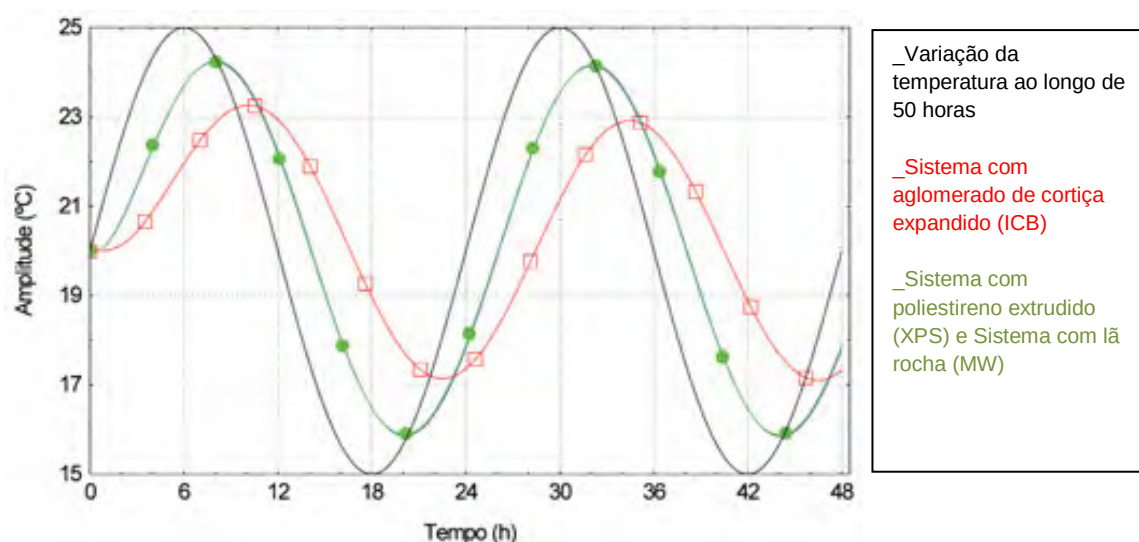
Figura 2.12 – Evolução da variação de temperatura na superfície exterior e interior dos sistemas ao longo de 50 horas.
