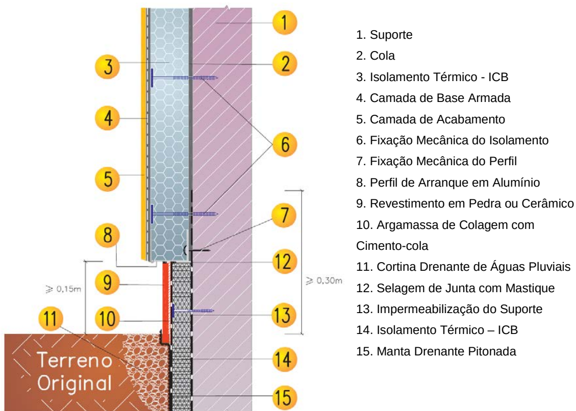
Figura 3.22 – Arranque do sistema enterrado.
