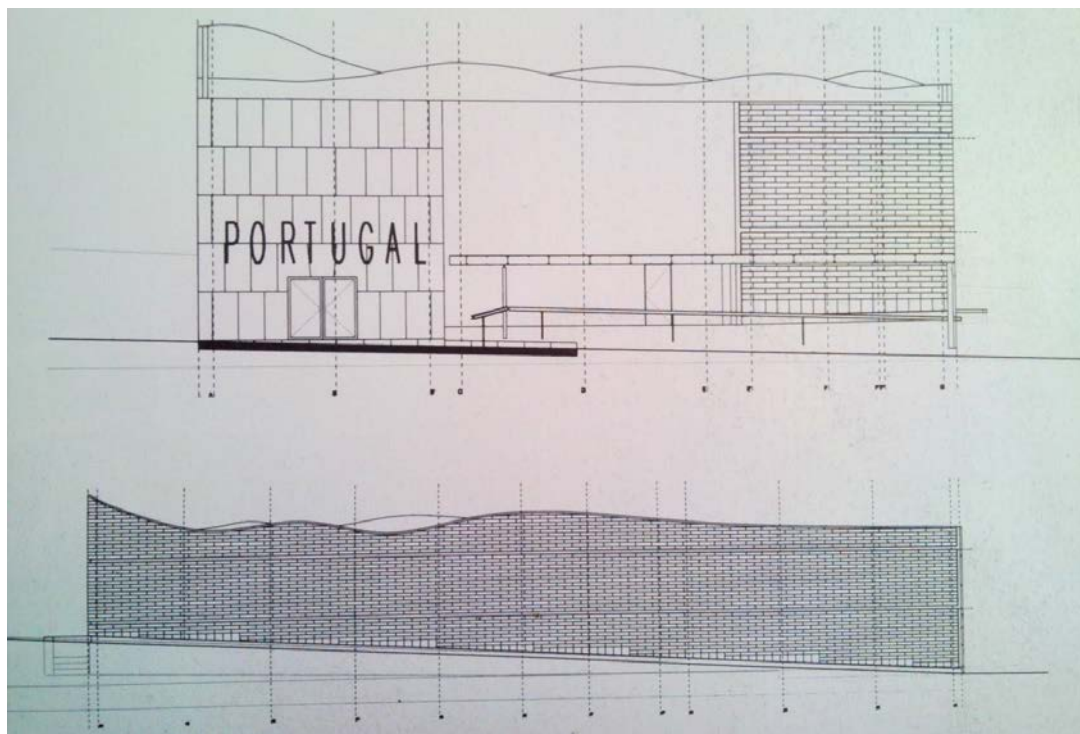
Figura 5.2 – Alçado principal oeste e lateral norte do Pavilhão Centro de Portugal.
