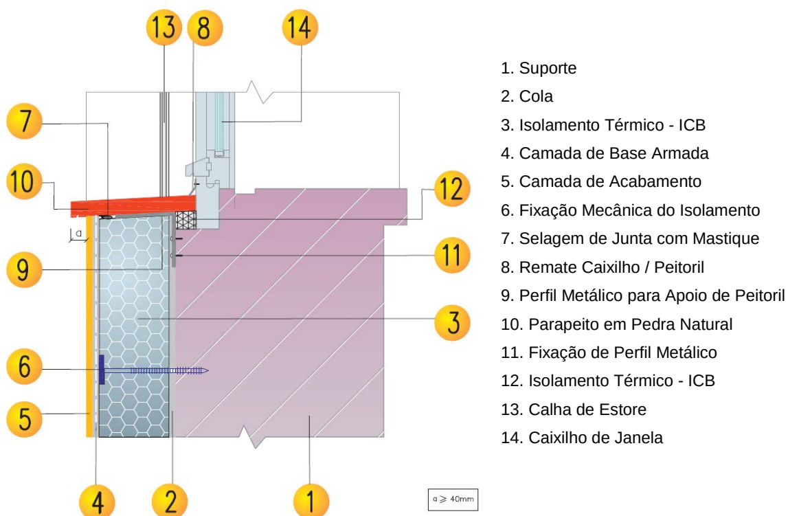
Figura 3.23 – Remate com peitoril de janela.
