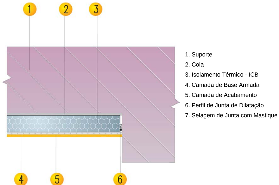
Figura 3.28 – Remate de elementos rígidos.
