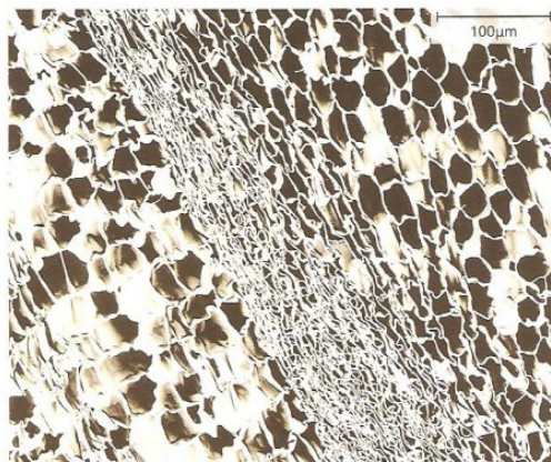
Figura 2.7 – Imagem da estrutura de um aglomerado de cortiça expandida do tipo térmico.
