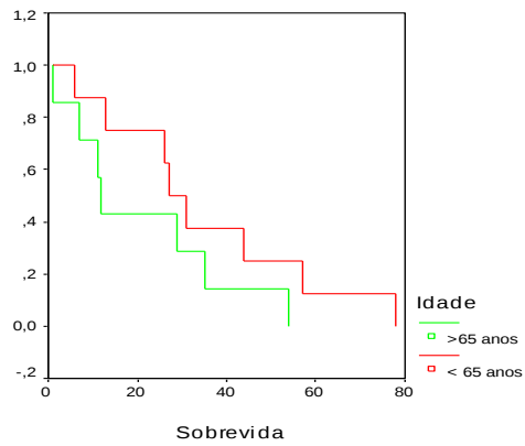
Figura 1. Sobrevivência global por grupo de idades (< 65 anos ou ≥ 65 anos).
