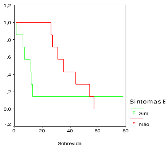
Figura 4. Curvas de sobrevivência global de acordo com a presença ou não de sintomas B (presença de febre, perda de peso e sudorese noturna) ao diagnóstico
