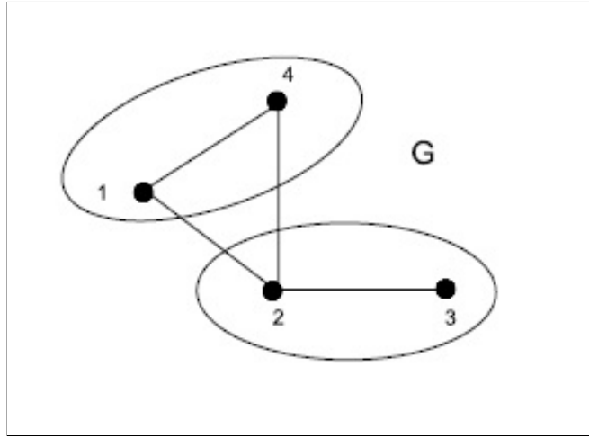
Figura 3.3: Bissecção do grafo(retirado de [16])
