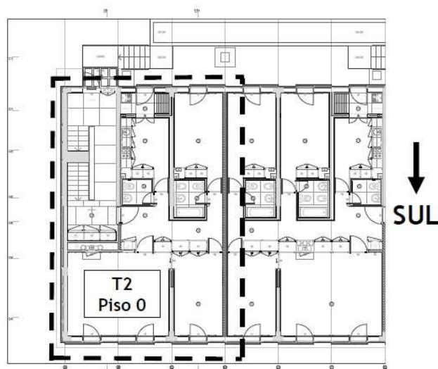
Figura 4.3 – Planta da fração autónoma estudada referente ao Caso de Estudo III (Freitas, V., 2012)
