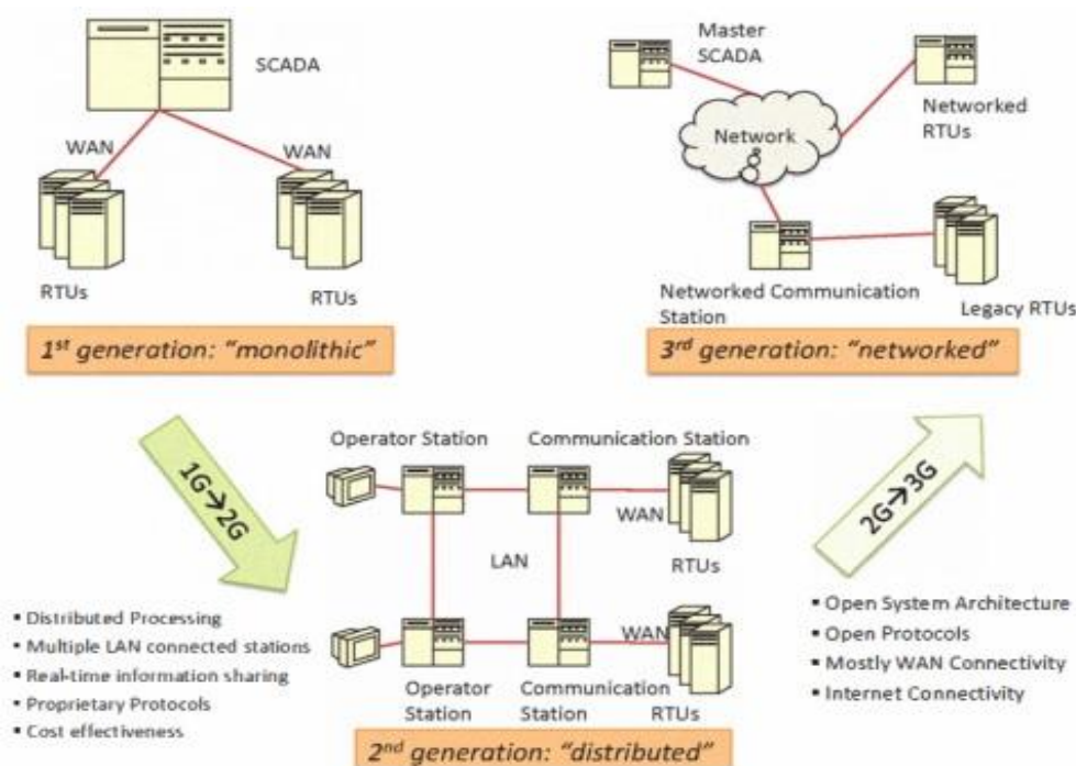
Figura 4.5 - Evolução do sistema SCADA [26].
