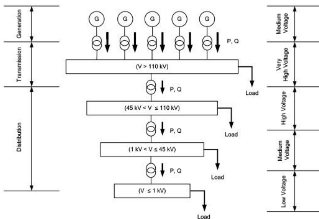
Figura 2.1 - Organização do Sistema Elétrico de Energia Tradicional [2].
