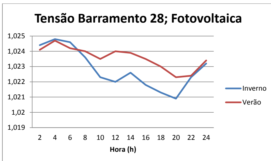
Figura 5.16 - Tensão no Inverno e no Verão, no barramento 28, PD fotovoltaica.
