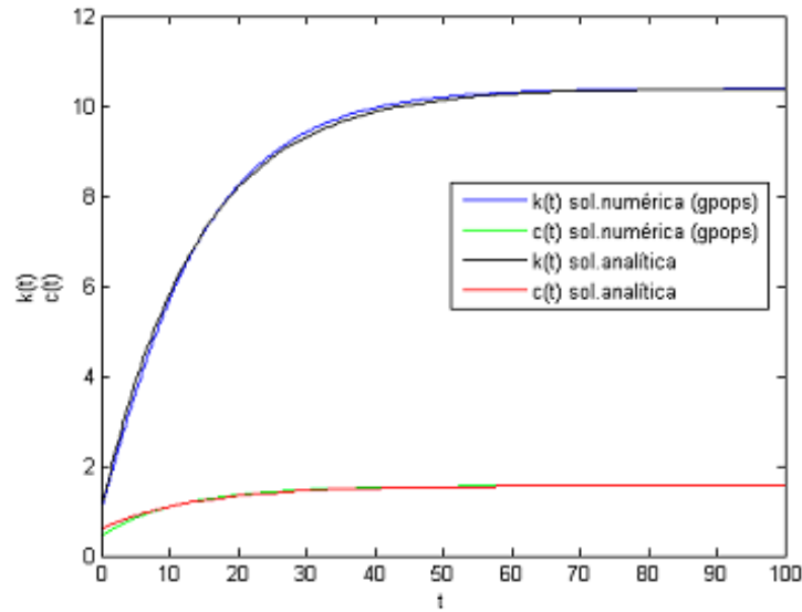
Figura 3: Solução analítica com a numérica (glops).
