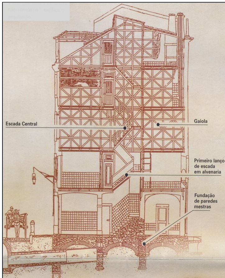
Modelo de Gaiola (pormenor)
