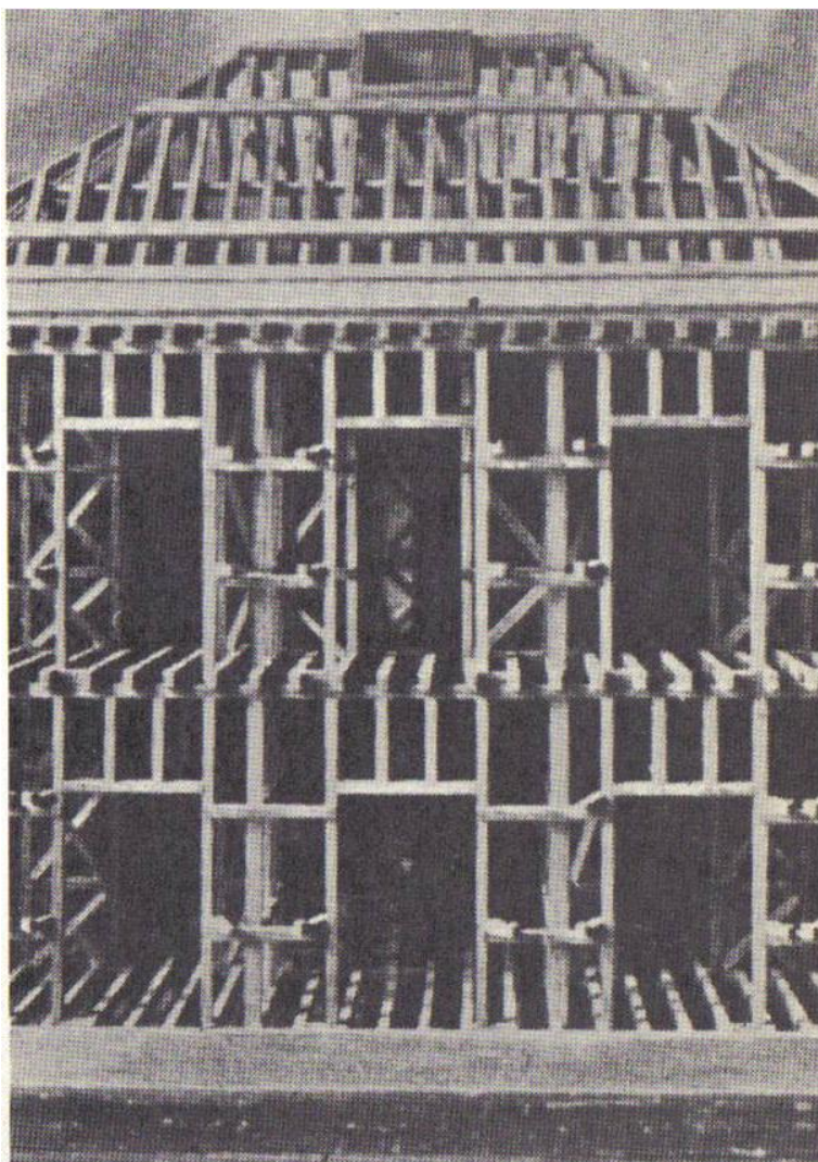
Modelo de Gaiola (pormenor), (FRANÇA,1978).
