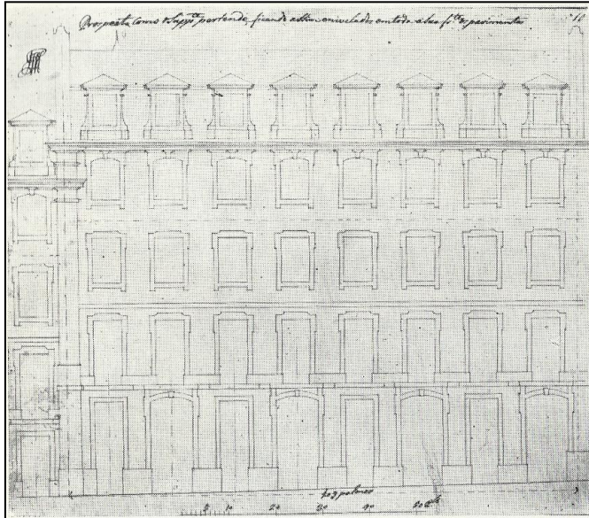
Fachada de tipo A
