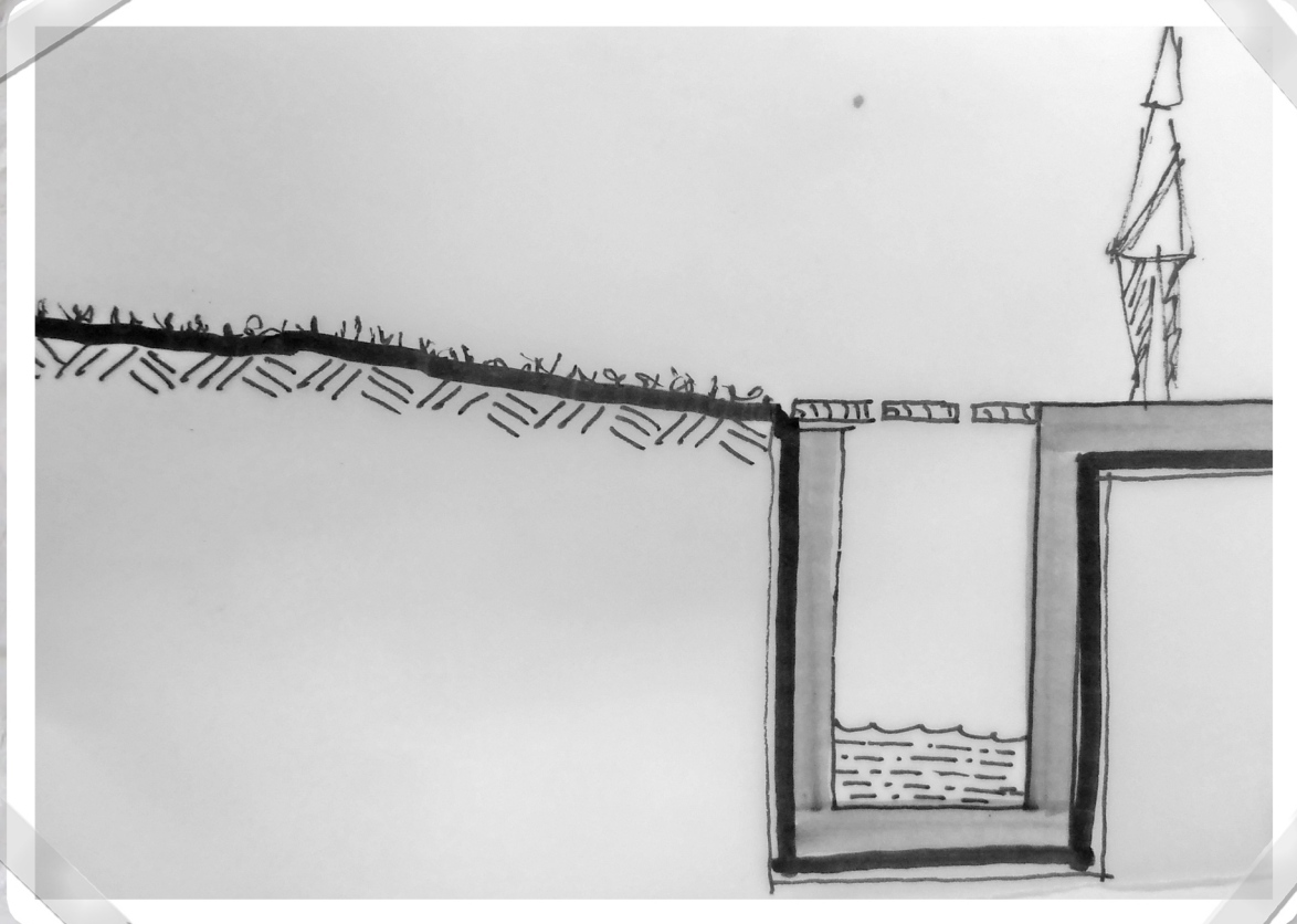
Proposta em corte - ribeira (desenho por José Miguel Lemeiras)
