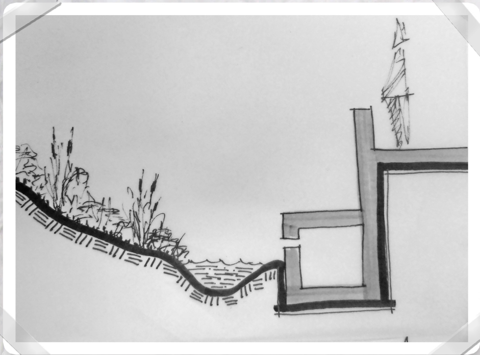
Proposta em corte - ribeira (desenho por José Miguel Lemeiras)
