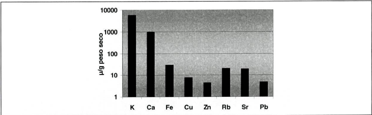
Gráfico 8 – Concentração média dos elementos metálicos nas uvas. Nota: Escala logarítmica.
