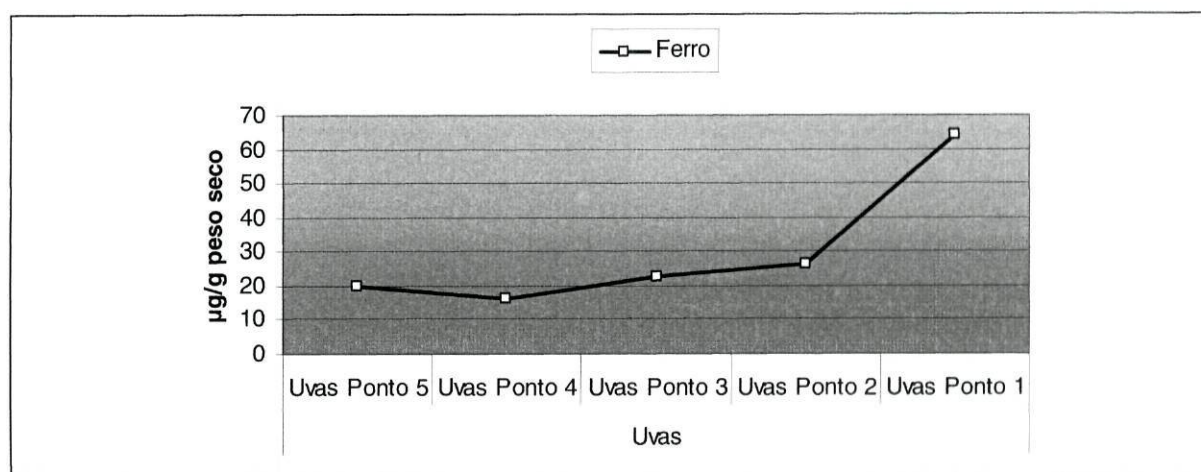
Gráfico a7 – Evolução dos teores de Ferro nas uvas da PM ao longo dos vários pontos de recolha de amostras. Ponto 5 é o ponto mais alto da parcela, e o ponto 1 é o mais baixo.
