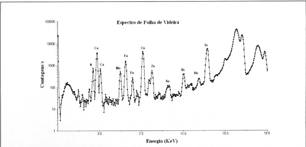
Gráfico a1 – Espectro de uma amostra de folhas de videira. Estão identificados os elementos traço e seus picos correspondentes.
