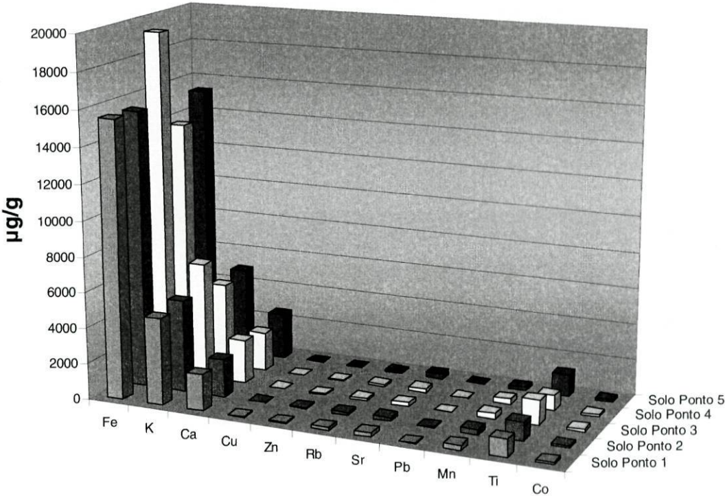
Gráfico a2 – Evolução dos teores dos elementos metálicos no solo da PM a diferentes altitudes de recolha de amostras. Ponto 5 é o ponto mais alto da parcela, e o ponto 1 é o mais baixo.
