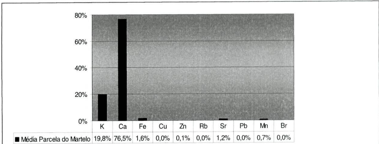
Gráfico 5 – Percentagem dos elementos metálicos na constituição das folhas.
