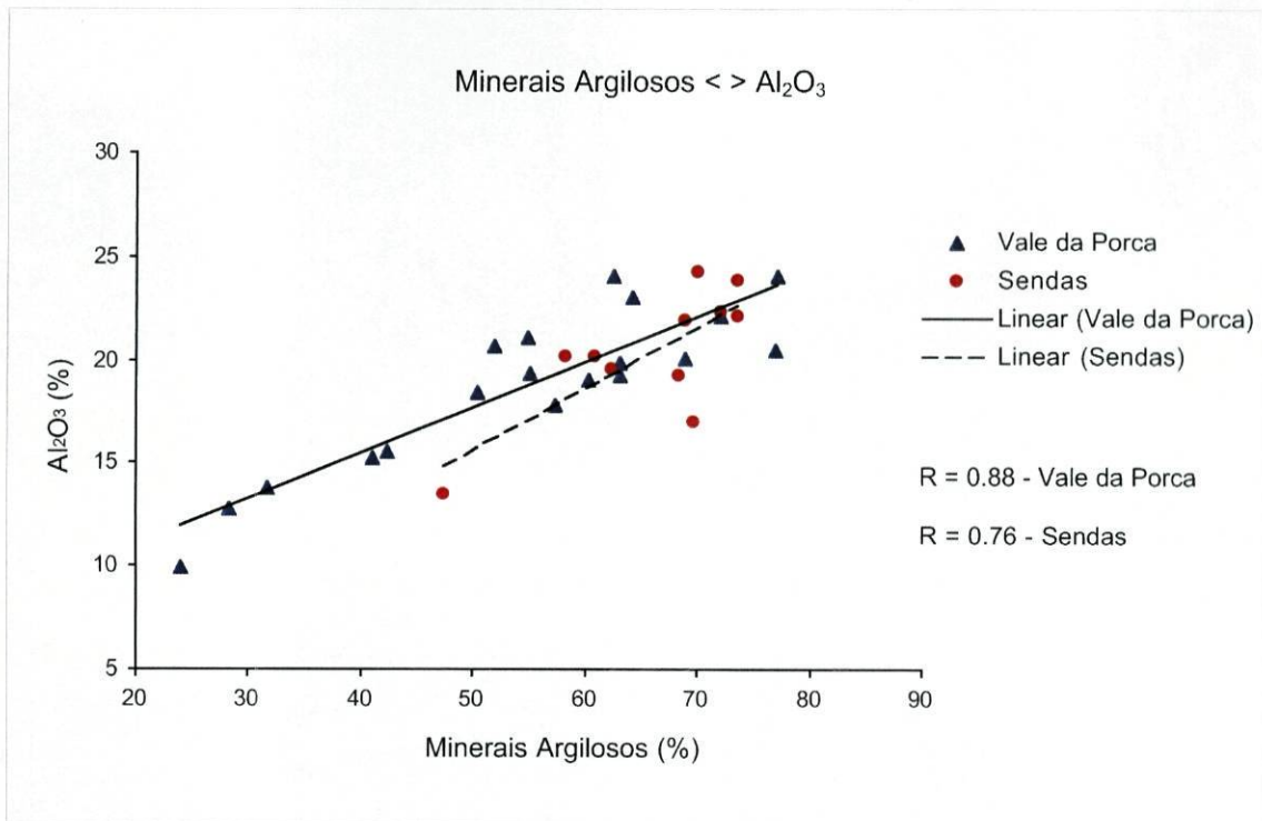
Figura 8.2 – Gráfico de correlação entre o teor de minerais argilosos (esmectite, ilite e caulinite) e o teor de Al 2 O 3 presente nos resíduos de exploração.
