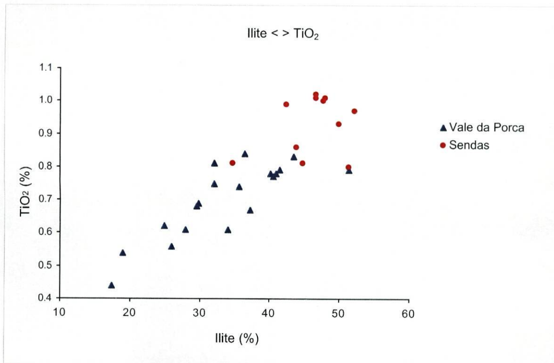
Figura 8.4 – Gráfico de correlação entre o teor de illite e o teor de \text{TiO}_2 .
