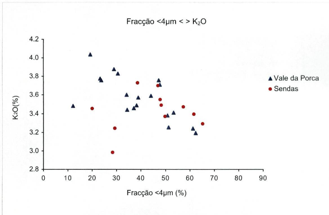
Figura 8.10 – Gráfico de correlação entre o teor de K_2O e a percentagem da fracção <4\mu m .
