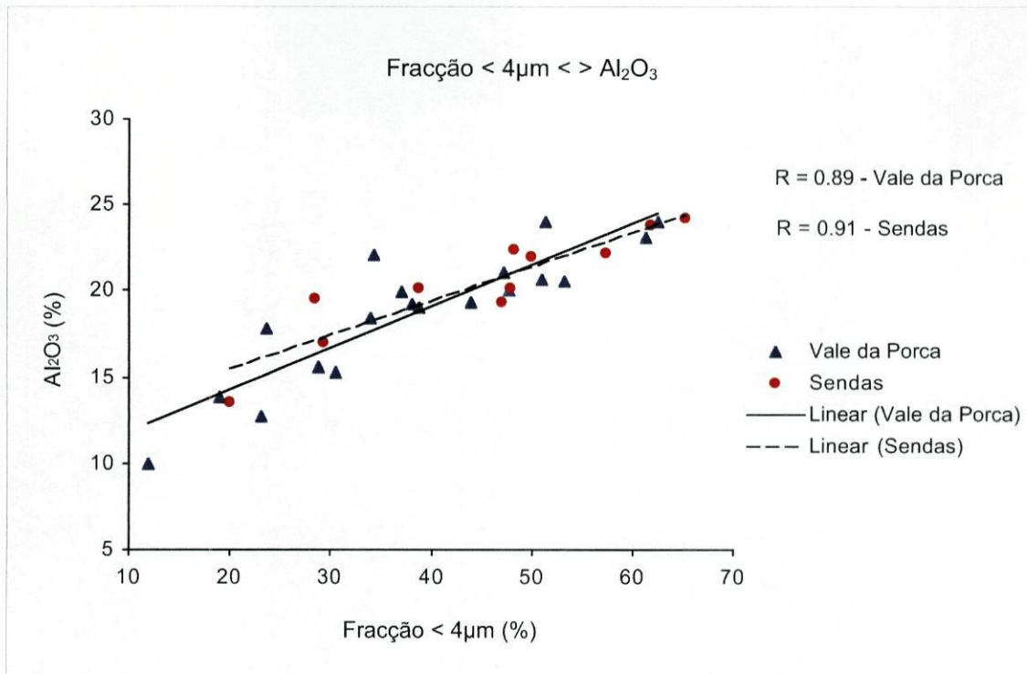
Figura 8.8 – Gráfico de correlação entre o teor de Al 2 O 3 e a percentagem da fracção < 4µm.
