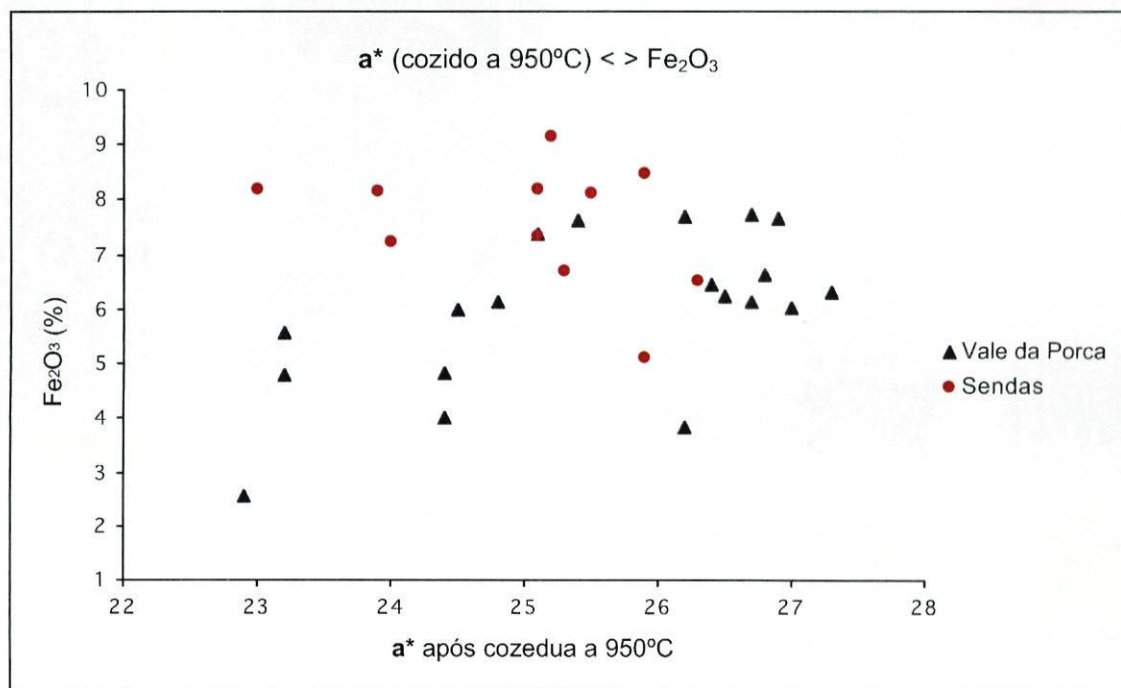
Figura 8.31. – Correlação entre os parâmetros cromáticos a^* após cozimento cerâmica a 950°C e o teor do Fe_2O_3 das amostras.
