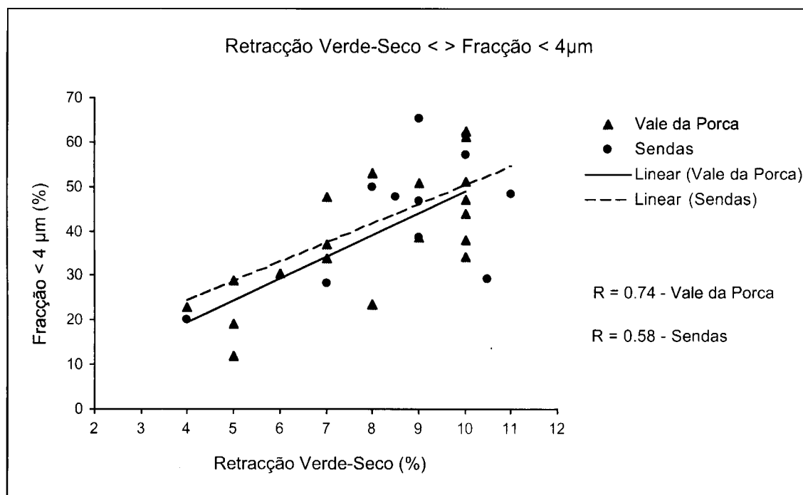
Figura 8.16 - Gráfico de correlação entre a retracção verde-séco e a percentagem da fracção < 4µm.
