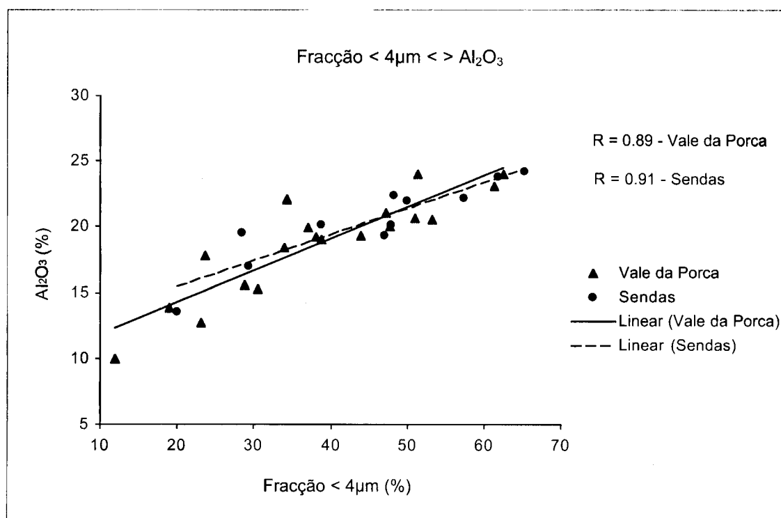
Figura 8.8 – Gráfico de correlação entre o teor de Al 2 O 3 e a percentagem da fracção < 4 \mu m.
