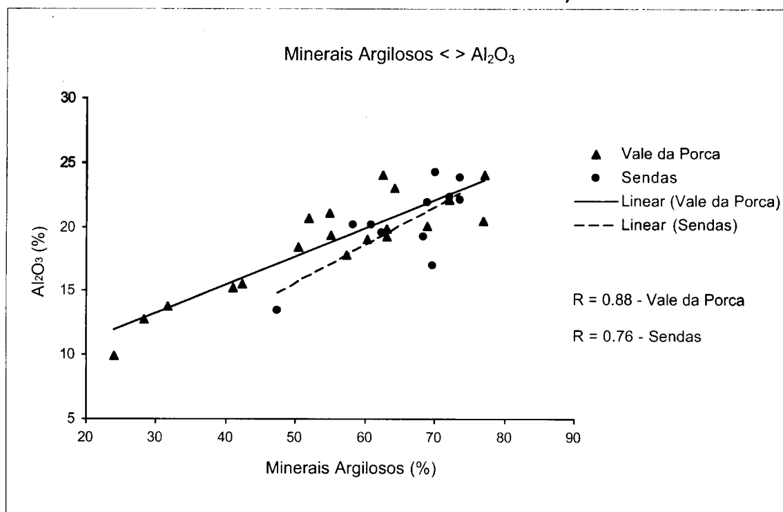
Figura 8.2 – Gráfico de correlação entre o teor de minerais argilosos (esmectite, ilite e caulinite) e o teor de \text{Al}_2\text{O}_3 presente nos resíduos de exploração.
