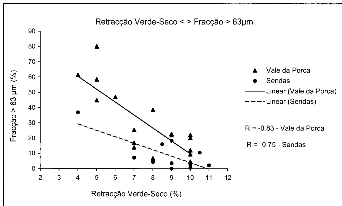
Figura 8.15 – Gráfico de correlação entre a retracção verde-séco e a percentagem da fracção > 63 µm.
