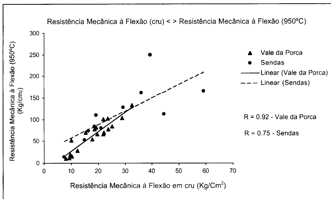
Figura 8.27 – Correlação entre a resistência mecânica à flexão em cru e a resistência mecânica à flexão após cozedura cerâmica a 950^{\circ}\text{C} .
