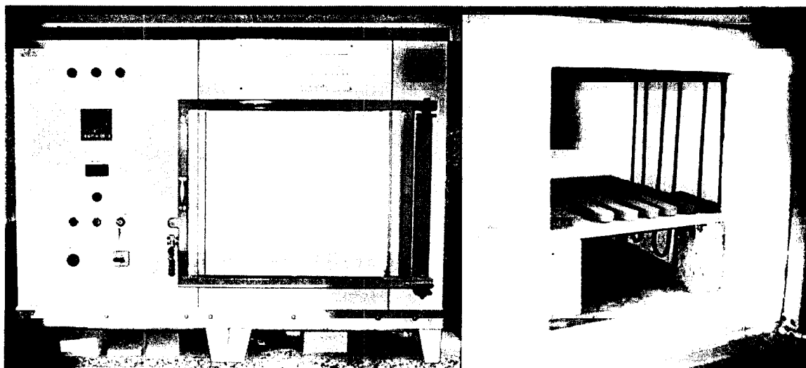
Figura 7.7 – Aspecto do forno cerâmico utilizado no laboratório do INETI, em São Mamede Infesta, para o processamento dos provetes a utilizar nos ensaios tecnológicos.
