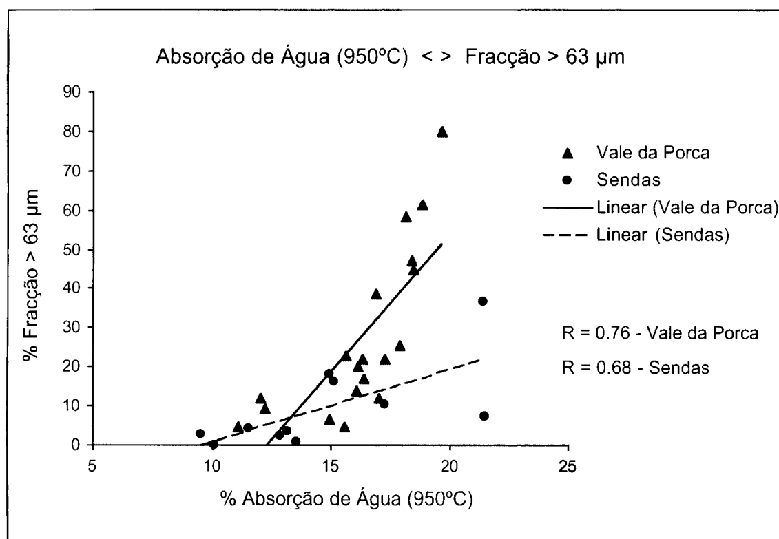
Figura 8.32 – Correlação entre a absorção de água em provetes cozidos a 950°C e a percentagem da fracção > 63 µm.
