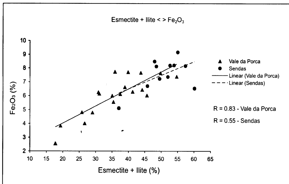
Figura 8.3 – Gráfico de correlação entre o teor de esmectite + ilite presente nos resíduos de exploração e o teor de \text{Fe}_2\text{O}_3 .
