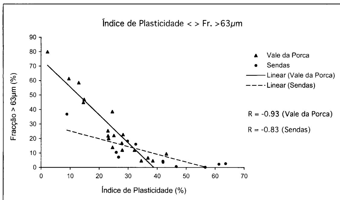
Figura 8.13 – Gráfico de correlação entre o índice de plasticidade e a percentagem de fracção > 63µm das amostras estudadas.
