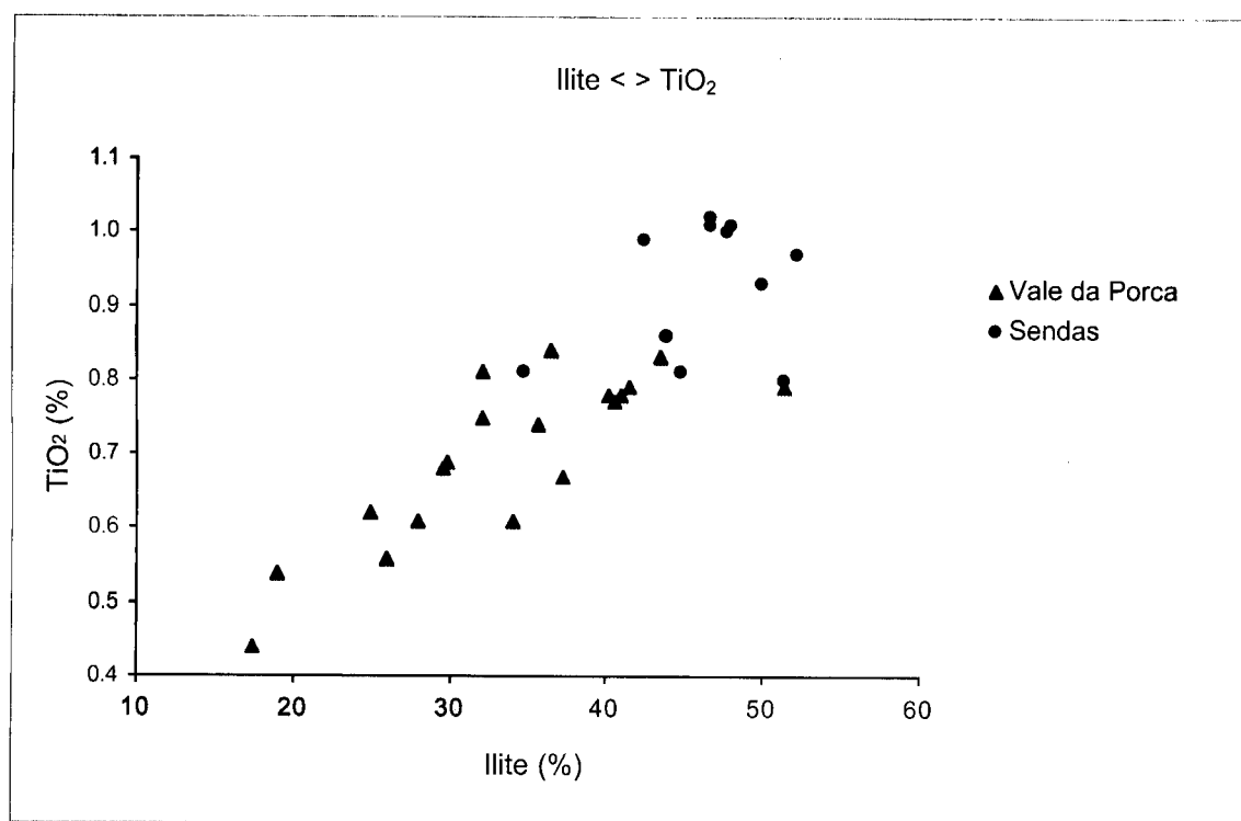
Figura 8.4 – Gráfico de correlação entre o teor de ilite e o teor de \text{TiO}_2 .
