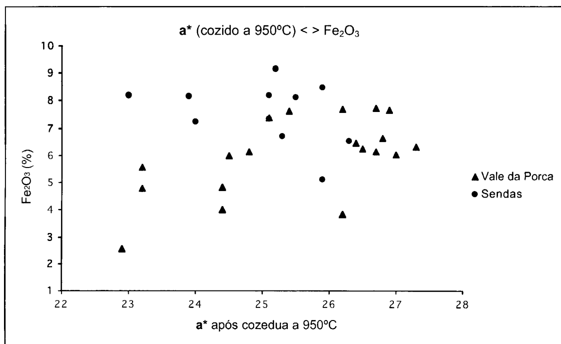
Figura 8.31. – Correlação entre os parâmetros cromáticos a^* após cozedura cerâmica a 950°C e o teor do \text{Fe}_2\text{O}_3 das amostras.
