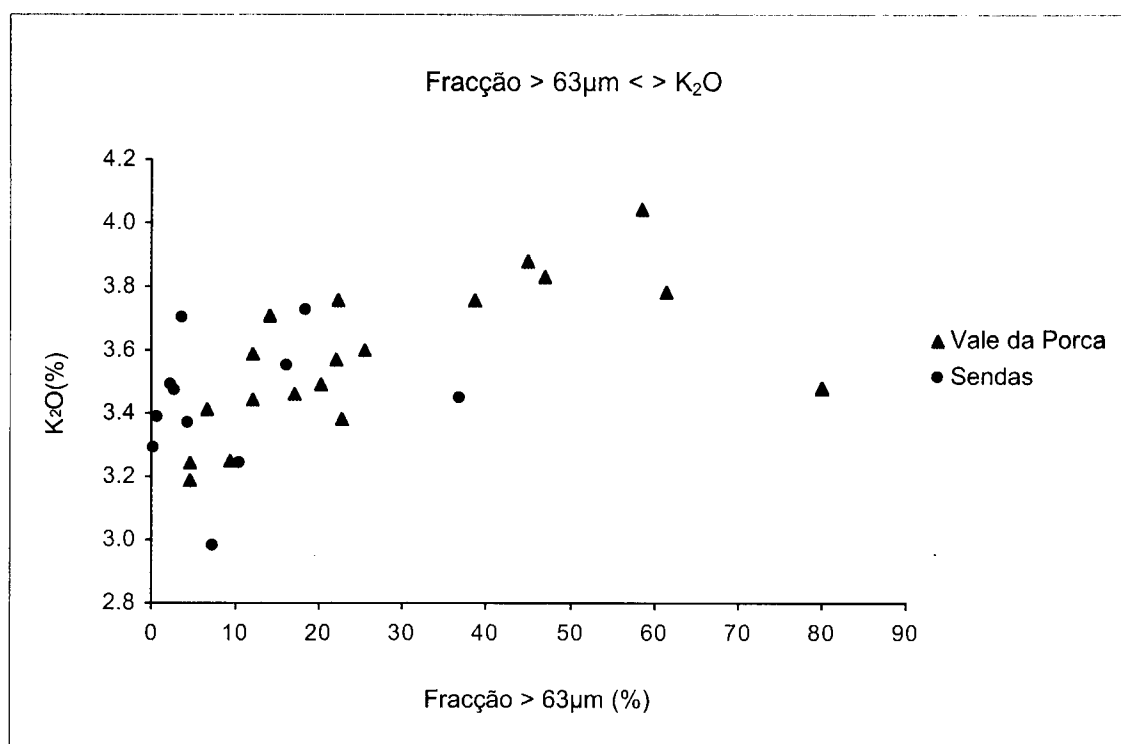
Figura 8.9 – Gráfico de correlação entre o teor de K 2 O e a percentagem da fracção > 63 \mu m.
