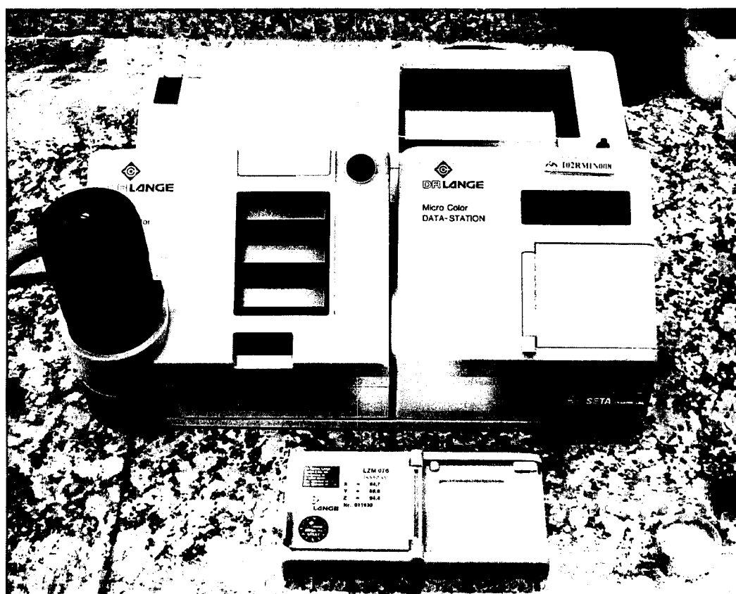
Figura 7.9 – Aspecto do colorímetro Micro Color II (V. 2.6) data station da Dr. Lange, utilizado no laboratório do INETI, em São Mamede Infesta.
