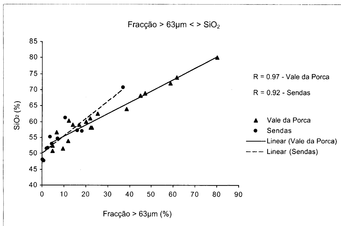
Figura 8.7 – Gráfico de correlação entre o teor de \text{SiO}_2 e a percentagem da fracção > 63\mu\text{m} .
