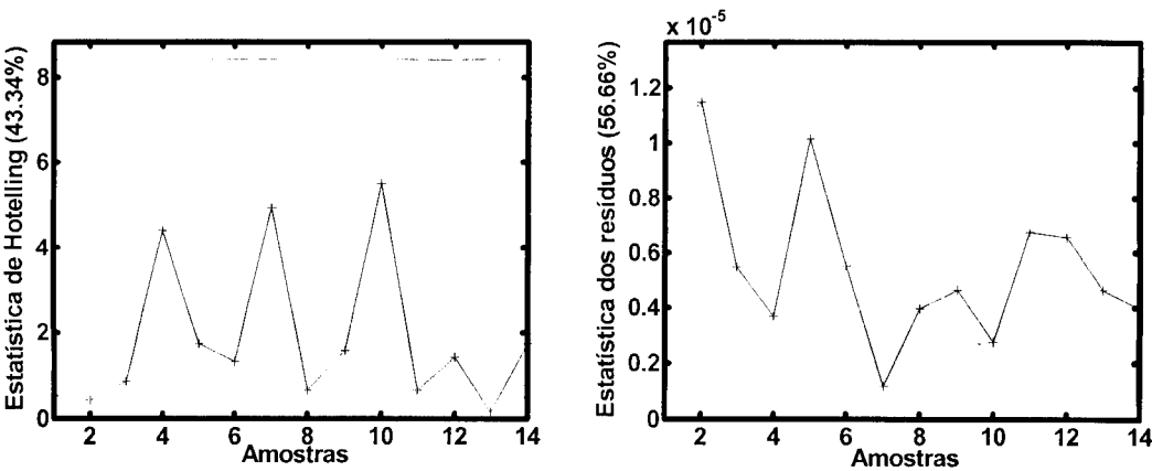
Figura 35. Valores das estatísticas de Hotelling e resíduos em função das amostras.
