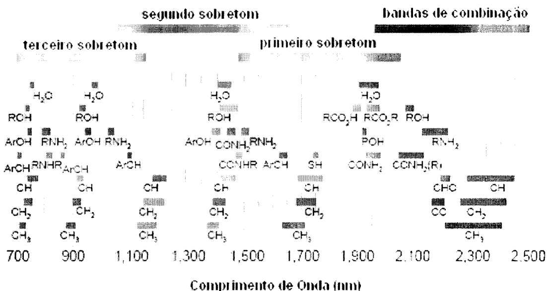
Figura 5. Mapa das principais bandas analíticas e localização no espectro na zona NIR (adaptado de Arnold et al., 2002).
