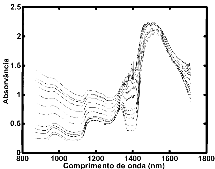
Figura 17. Espectros normais obtidos do efluente a diferentes concentrações
