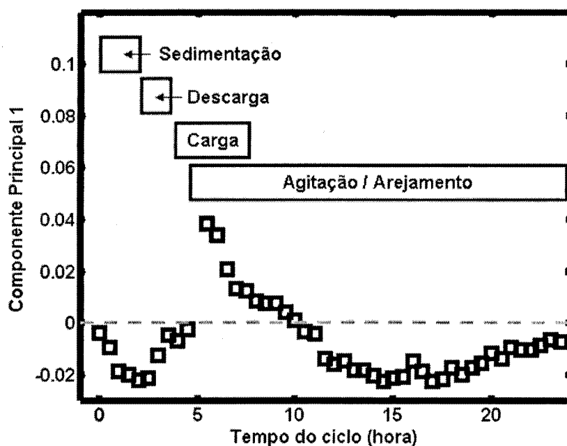
Figura 44. Primeiro componente principal relativo ao ensaio de 10.05.06. Os espectros foram pré-processados com um filtro de Savitzsky-Golay (27,2,1) e centrados na média. As barras no topo do gráfico indicam as fases do ciclo.
