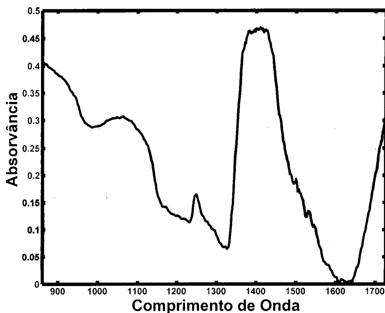
Figura 42. Espectro NIR de transfectância obtido para o ensaio 1 às 0:00 horas (final da fase de reacção/início da fase de sedimentação).
