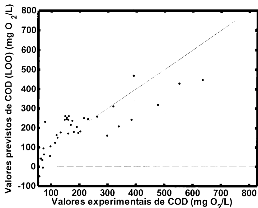
Figura 28. Valores de COD medidos em função dos valores de COD previstos pelo modelo PLS com três componentes resultado da validação (LOO).
