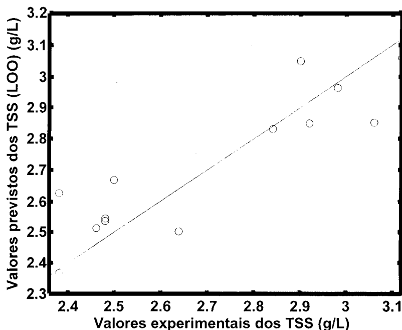
Figura 36. Valores de TSS medidos em função valores de TSS previstos pela validação cruzada.
