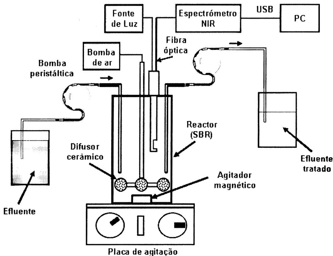
Figura 12. Esquematização do sistema utilizado para tratamento do efluente (reactor SBR).
