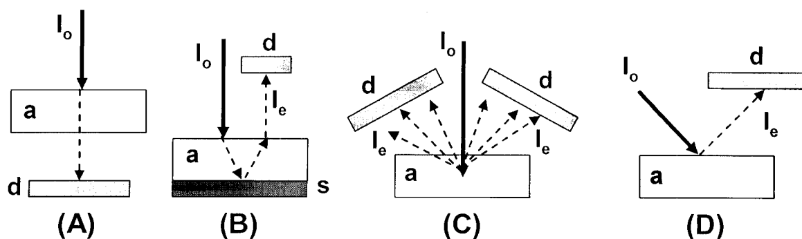
Figura 7. Modos de medição tipicamente utilizados em espectroscopia NIR ( I_o -feixe incidente, I_e -feixe emergente, a-amostra, s-superfície reflectora, d-detector).
