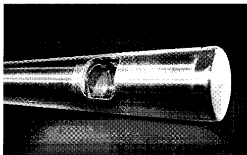
Figura 8. Ampliação da ponta de uma sonda de transfectância (adaptado de www.oceanoptics.com ).
