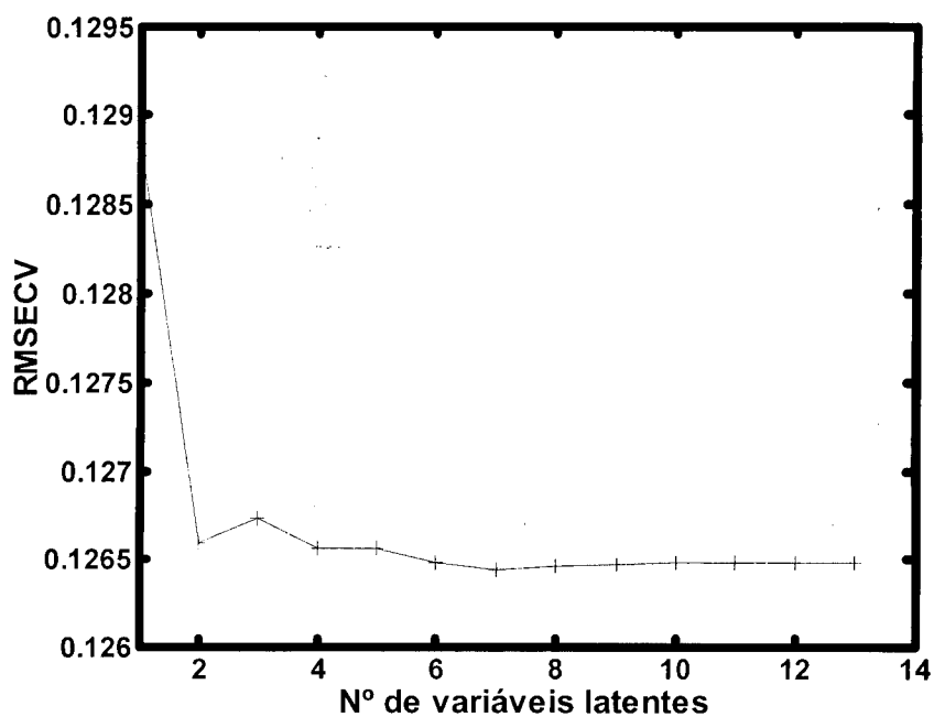
Figura 32. Erro da validação cruzada em função do número de variáveis latentes
