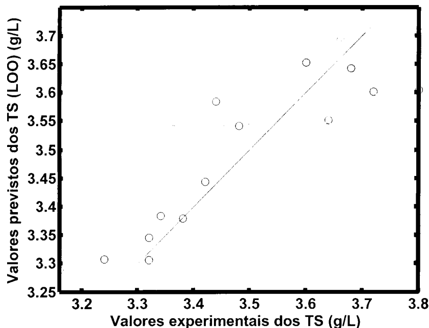
Figura 41. Valores de TS experimentais em função valores de TS previstos pela validação cruzada.
