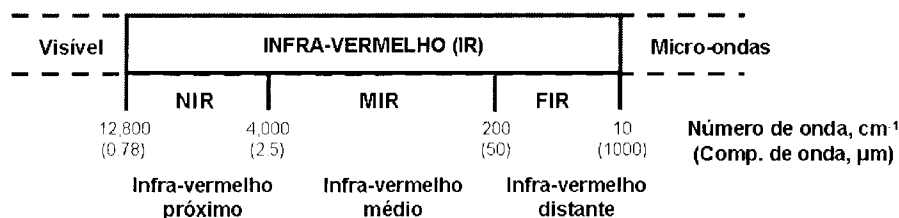
Figura 4. Divisão da região do espectro electromagnético relativo ao infra-vermelho nas componentes infra-vermelho próximo (NIR), médio (MIR) e distante (FIR).
