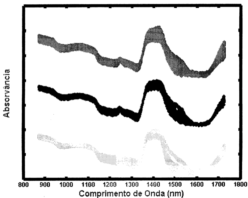
Figura 43. Representação dos espectros sobrepostos correspondentes aos ensaios de calibração (topo), ensaio A1 (meio) e ensaio atípico A2 (baixo).
