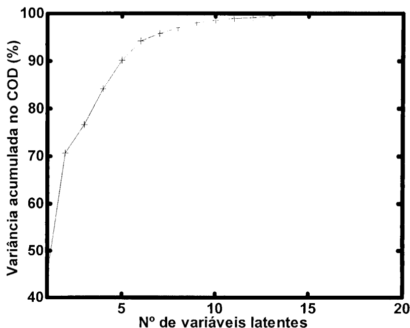
Figura 26. Percentagem da variância cumulativa capturada de COD em função do número de variáveis latentes.
