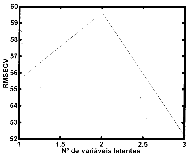
Figura 29. Gráfico do erro da validação cruzada para o modelo PLS de previsão do COD.
