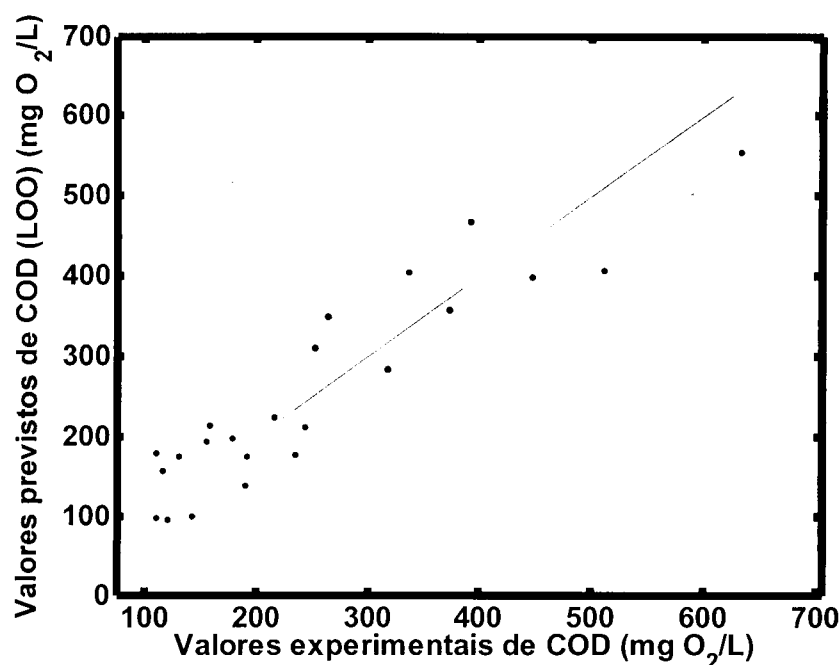
Figura 31. Valores de COD medidos em função dos valores de COD previstos pelo modelo MLR com utilização dos comprimentos de onda de 285 e 510 nm (resultado de validação LOO).
