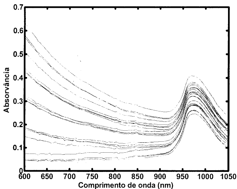
Figura 14. Espectros normais obtidos do efluente a diferentes concentrações em 4 dias.
