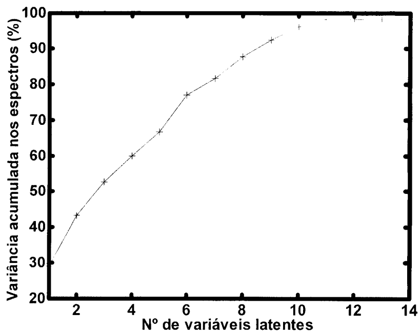
Figura 33. Percentagem da variância cumulativa capturada nos espectros em função do número de variáveis latentes.
