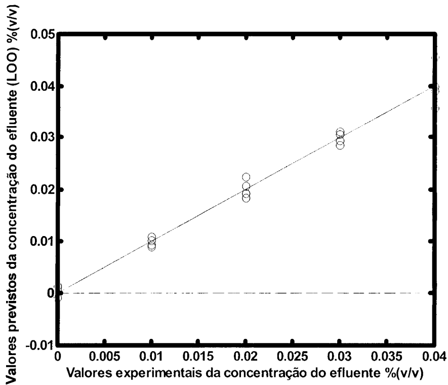
Figura 16. Valores de concentração do efluente em % (v/v) medidos em função valores de concentração do efluente previstos pelo modelo PLS (valores da validação cruzada)
