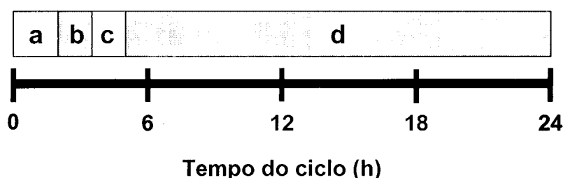
Figura 13. Esquema descritivo das fases do ciclo do reactor SBR.
