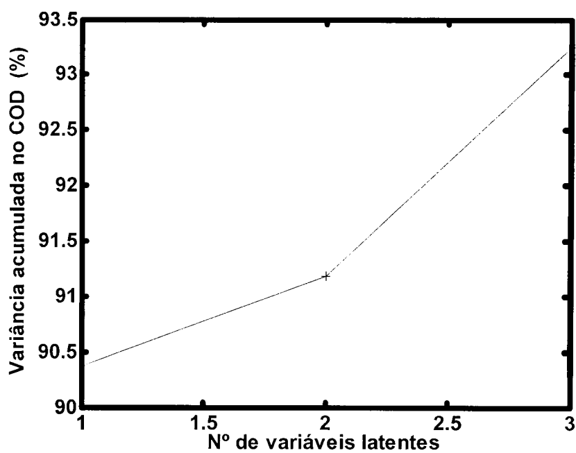
Figura 30. Percentagem de variância cumulativa capturada do COD em função do número de variáveis latentes para um modelo PLS.
