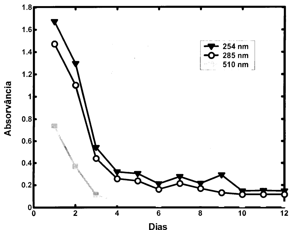
Figura 20. Valores de absorvâncias a 3 comprimentos de onda das amostras recolhidas do efluente tratado no final do ciclo do SBR (depois de centrifugadas).
