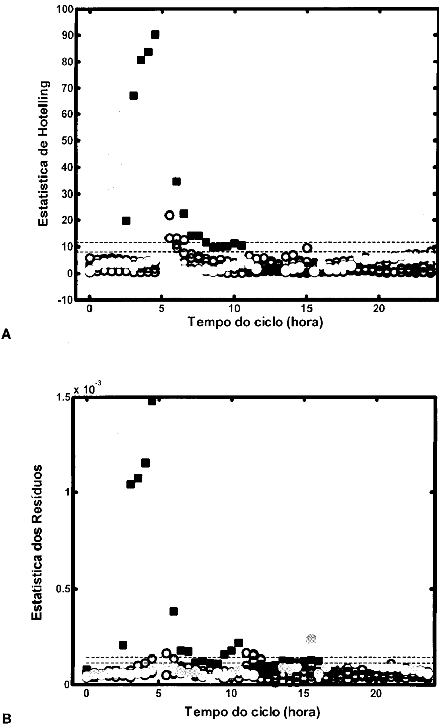
Figura 48. Estatísticas de Hotelling (A) e dos resíduos (B) em função do tempo para os ensaios nominais e para os dois ensaios projectados.
