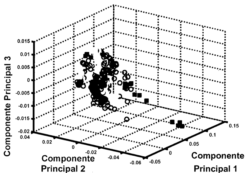
Figura 46. Mapa de componentes principais para os ensaios monitorizados com a sonda NIR in-situ . Os ensaios de calibração (1-6) foram usados para geração do modelo (pré-processamento com Savitzky-Golay (27,2,1) e centro na média). A variância capturada nos três componentes principais é de 95.6%. Projectam-se os ensaios A1 e A2.
