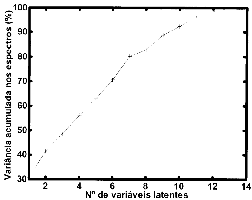
Figura 38. Percentagem da variância cumulativa capturada nos espectros em função do número de variáveis latentes.
