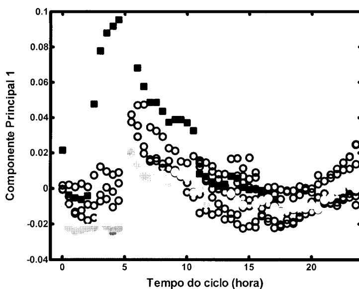
Figura 47. Evolução do primeiro componente principal em função do tempo para os ensaios nominais e para os dois ensaios projectados.
