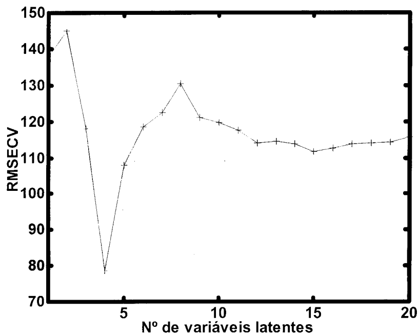
Figura 24. Gráfico do erro da validação cruzada para o modelo PLS de previsão do COD.
