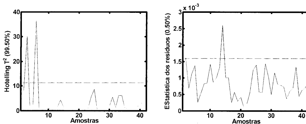
Figura 27. Valor da estatística de Hotelling e resíduos obtido em função das amostras.
