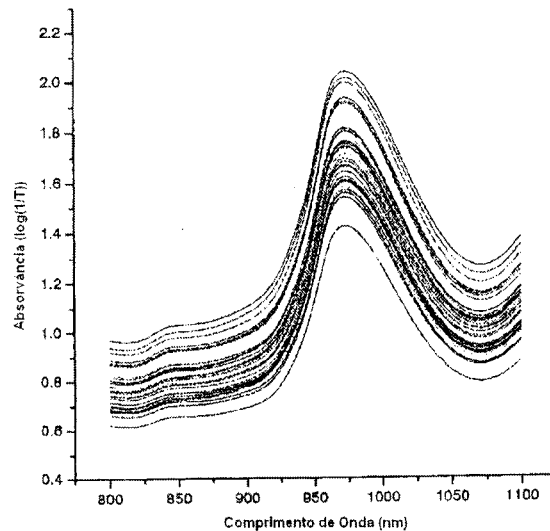
Figura 9. Espectros de infravermelho próximo (onda curta) obtidos para amostras de leite (adaptado de Sasic e Ozaki, 2001).
