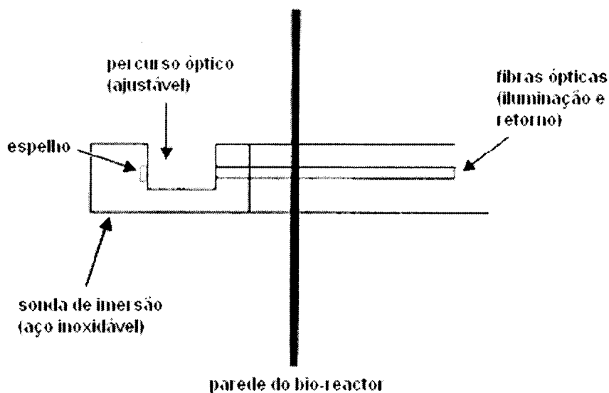
Figura 10. Esquema da sonda de transfectância usada para monitorização in-situ do reactor de lamas activadas.
