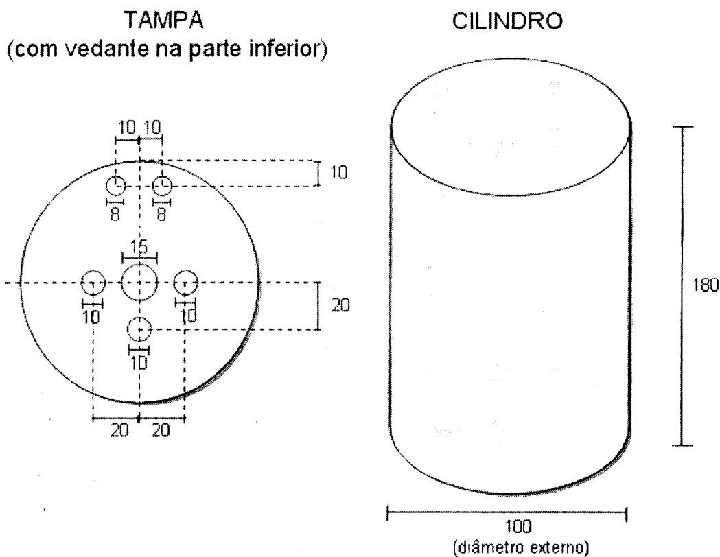
Figura 11. Esquema do reactor de escala laboratorial utilizado para execução dos ensaios de tratamento de resíduos lácteos por lamas activadas.
