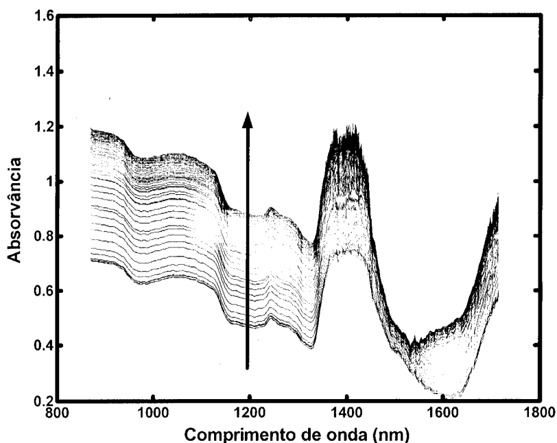
Figura 22. Influência da agitação na aquisição dos espectros NIR no reactor com inóculo (aproximadamente 3 g/L)
