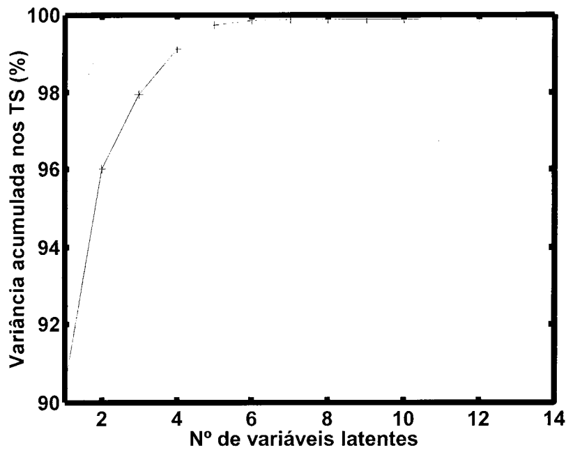
Figura 39. Percentagem da variância cumulativa capturada nos TS em função do número de variáveis latentes.
