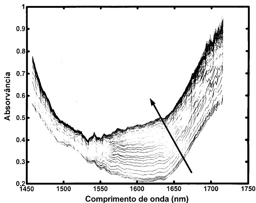
Figura 23. Ampliação da zona entre 1450 nm e 1750 nm mostrando o deslocamento do mínimo de uma banda espectral.
