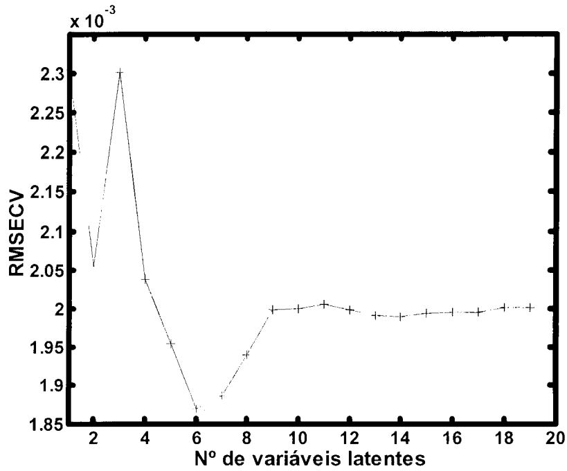
Figura 15. Erro da validação cruzada em função do número de variáveis latentes
