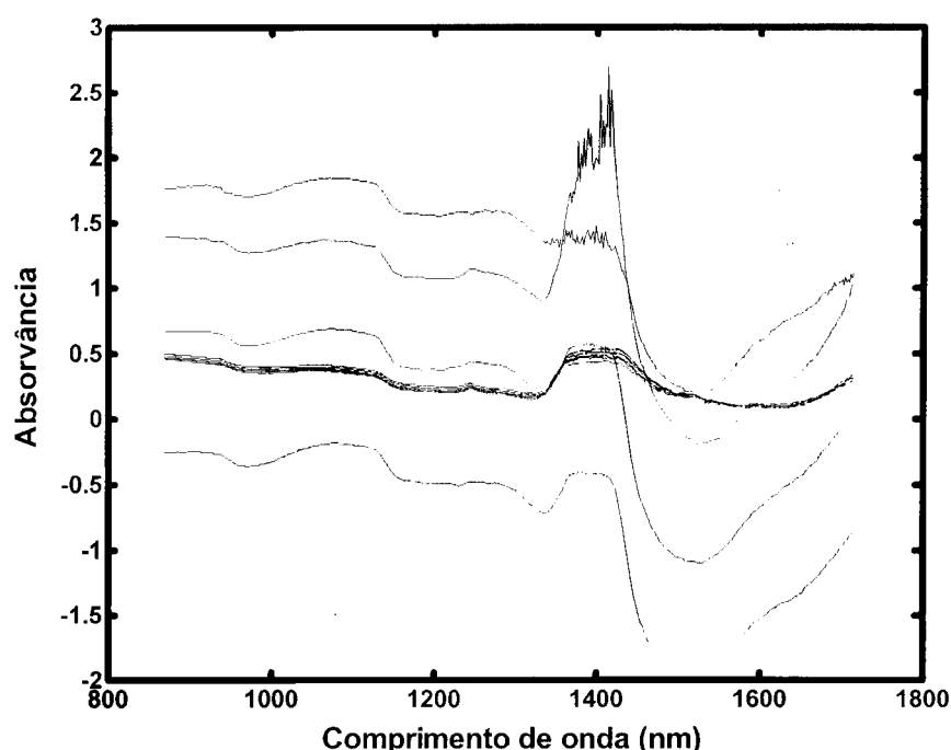
Figura 21. Influência da presença de bolhas de ar no percurso óptico da sonda devidas ao sistema de arejamento no reactor com inóculo (aproximadamente 3 g/L de TS).
