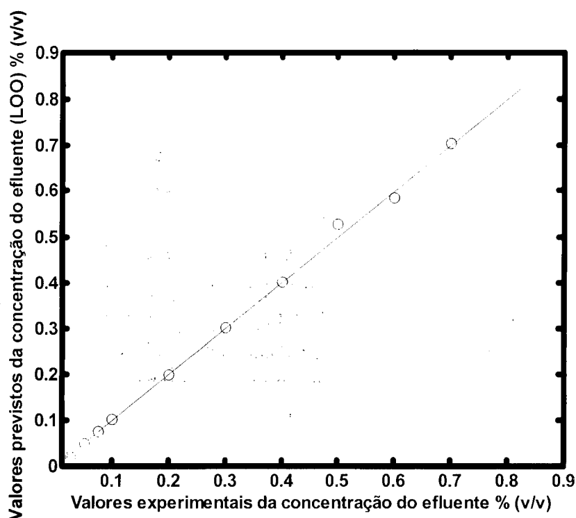
Figura 19. Valores de concentração do efluente em % (v/v) medidos em função valores de concentração do efluente previstos pela validação cruzada
