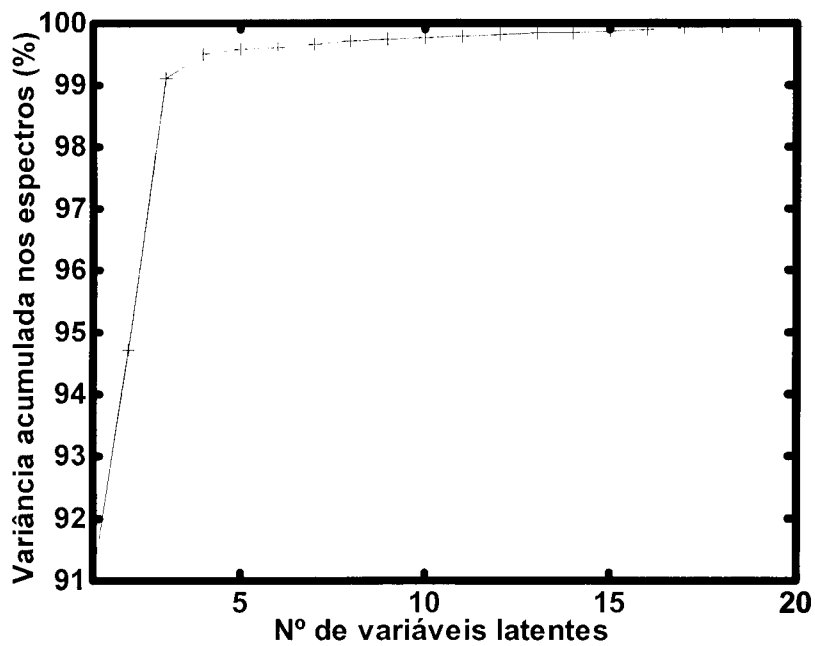
Figura 25. Percentagem de variância cumulativa capturada dos espectros NIR em função do número de variáveis latentes.
