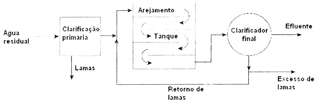
Figura 1. Esquematização sumária de um processo contínuo de tratamento de efluentes por lamas activadas.
