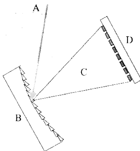
Figura 6. Esquema de um equipamento dispersivo com policromador (detector linear de foto-díodos, PDA).
