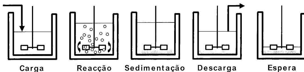
Figura 2. Esquema das diferentes etapas de um reator do tipo SBR. O último passo (de espera) justifica-se quando existem diferentes tanques e é necessário um período de tempo para mudança de tanque.
