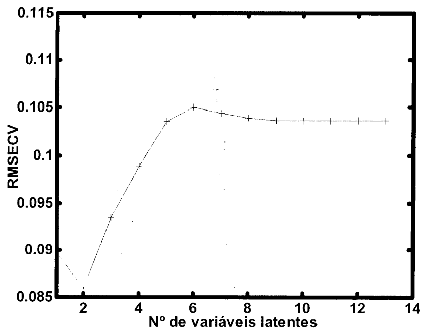
Figura 37. Erro da validação cruzada em função do número de variáveis latentes.
