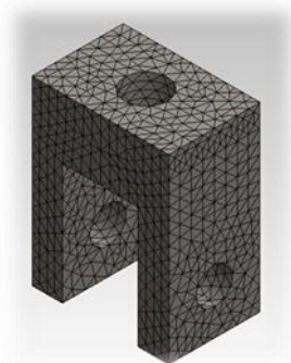
Figura 41 - Representação esquemática da malha utilizada no actuador
