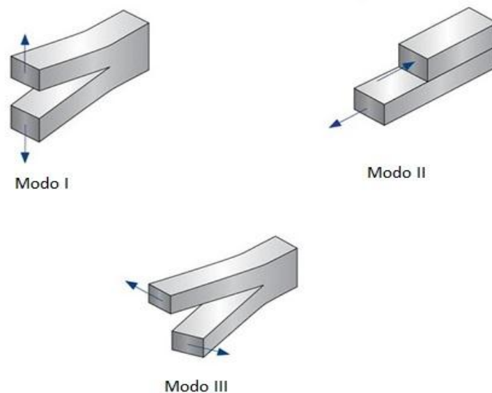
Figura 2- Representação dos diferentes modos de fractura
