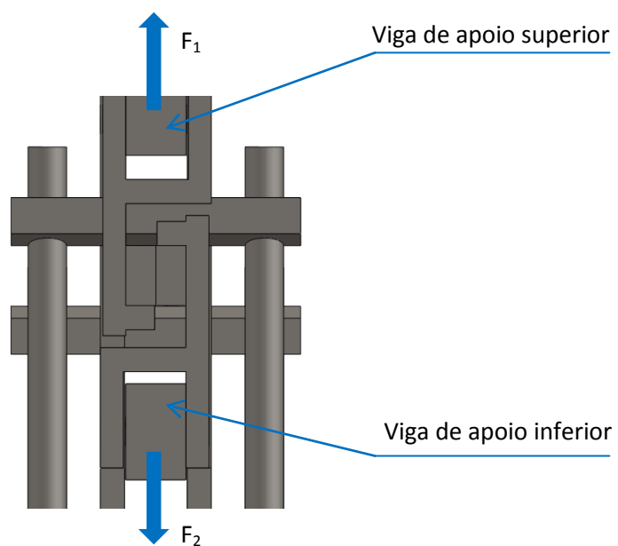
Figura 55 - Modo como actuam as forças com adaptação para modo III
