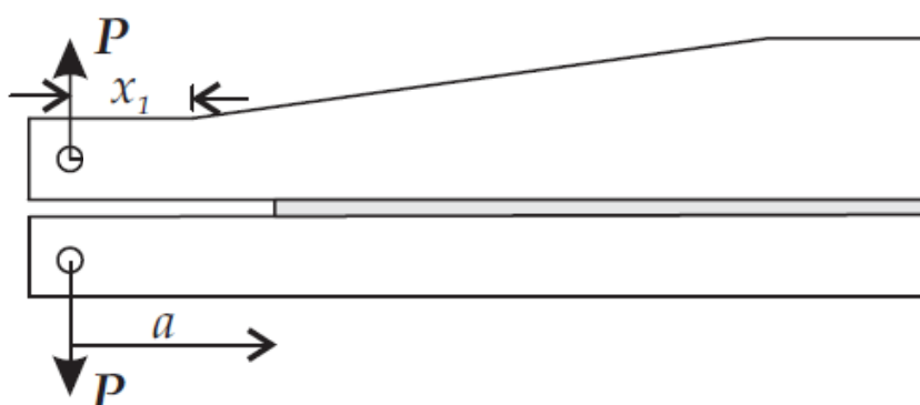
Figura 19 - Representação esquemática do ensaio ATDCB [5]
