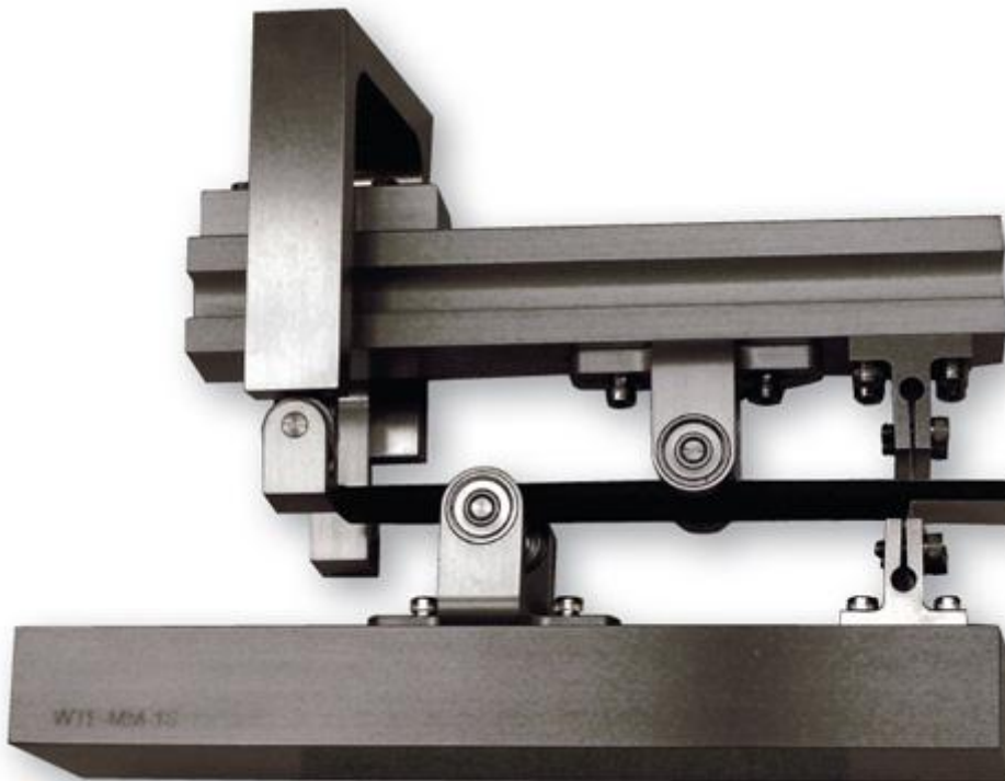
Figura 21 – Representação de um dispositivo para efectuar o ensaio MMB [30]
