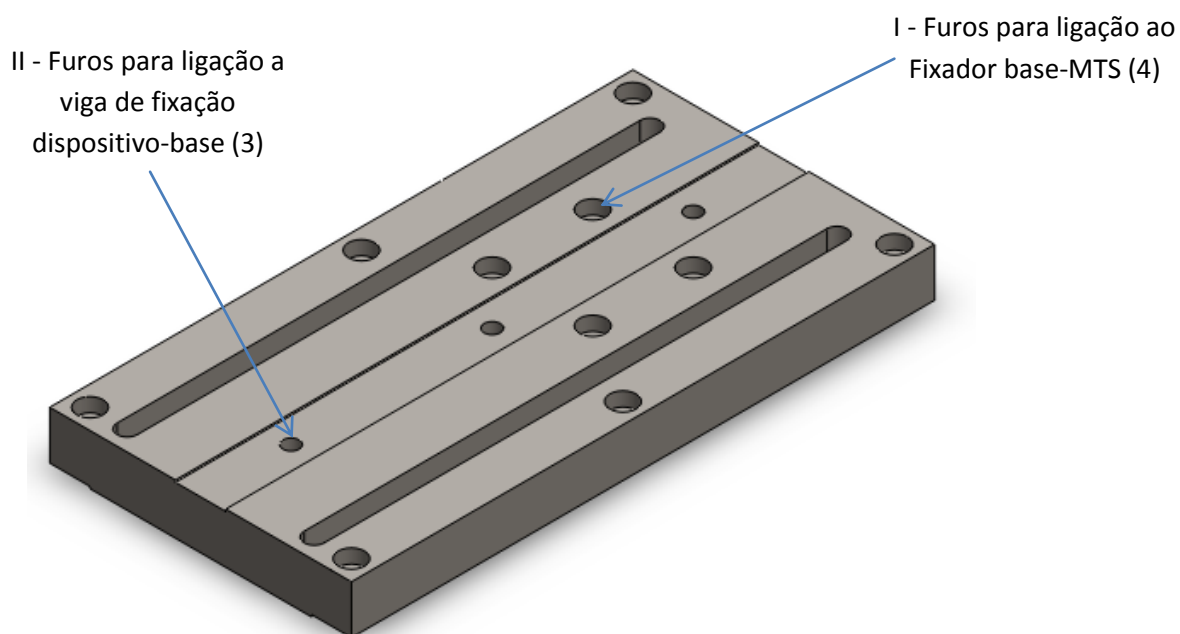
Figura 51 - Representação da base
