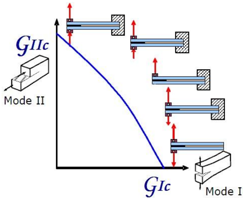
Figura 16- Variação da geração do modo misto com assimetria da carga aplicada em provetes DCB [28]
