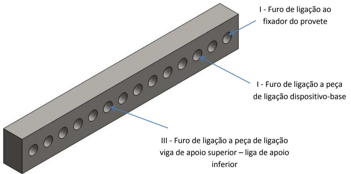
Figura 48 - Representação da viga se apoio superior
