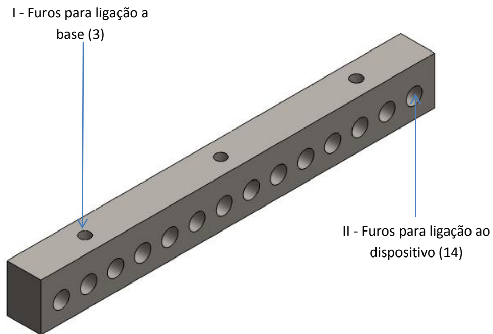
Figura 50 - Representação da viga de fixação dispositivo-base
