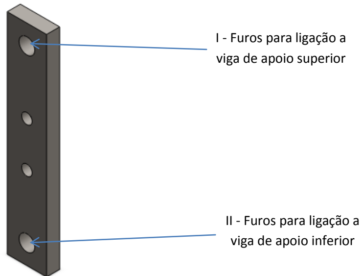
Figura 47 - Representação da peça de ligação viga de apoio superior – liga de apoio inferior
