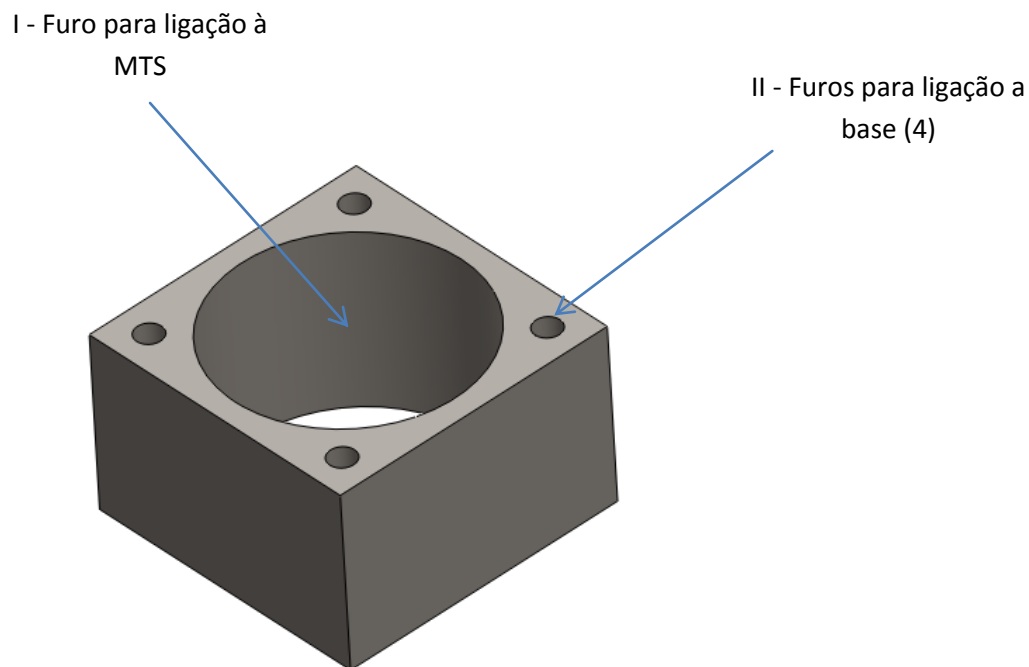
Figura 52 - Representação do fixador base-MTS
