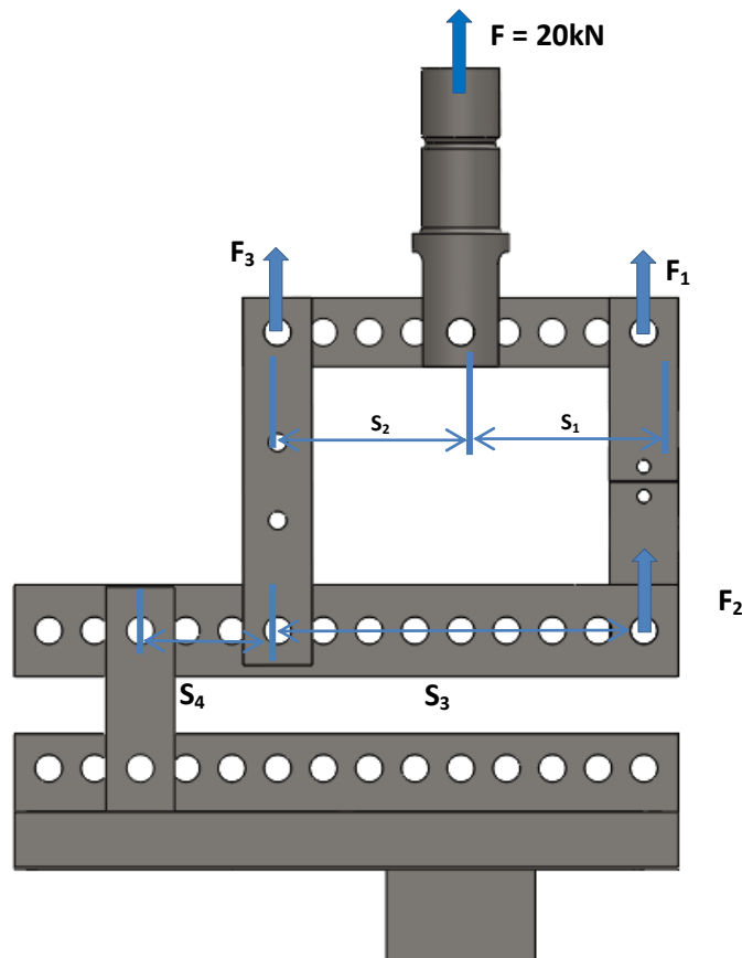
Figura 37 - Representação esquemática das forças que actuam no provete
