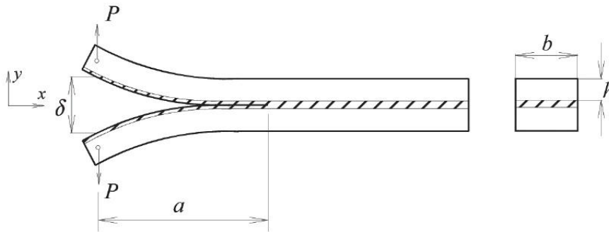
Figura 4 - Representação esquemática do ensaio DCB [6]
