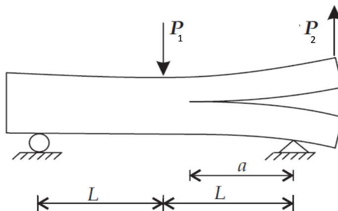
Figura 23 - Representação esquemática da aplicação das forças num ensaio MMB [31]
