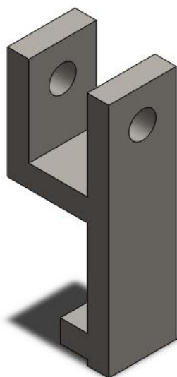
Figura 53 - Fixador da barra de ensaio para modo III
