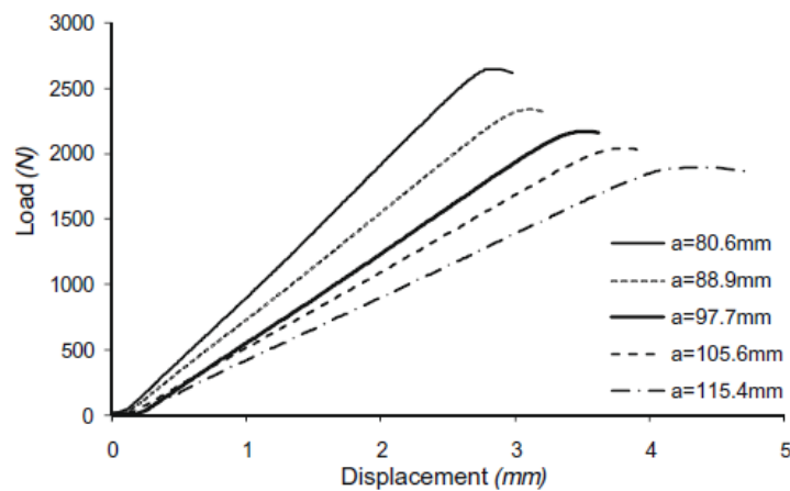
Figura 36 - Forças obtidas para o ensaio Fernlund-Spelt [36]
