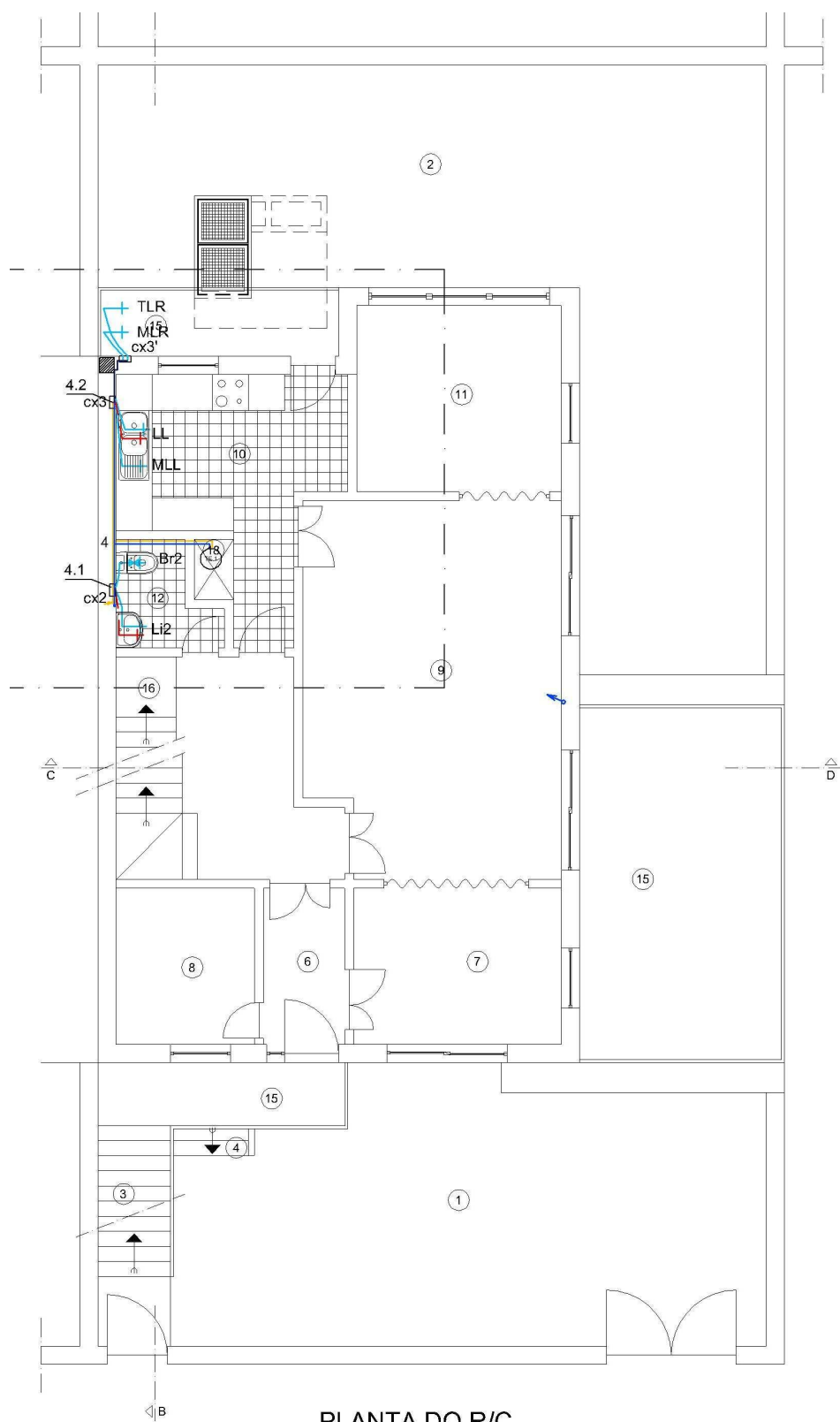
PLANTA DO R/C
