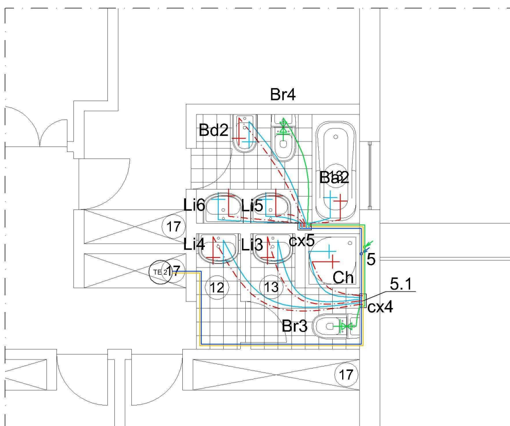
Figura B2.6: HIPÓTESE I – Pormenor do WC da cave
