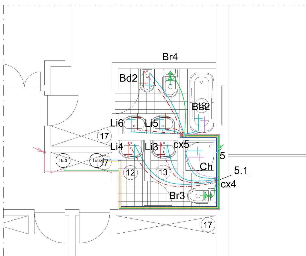
Figura B3.7: HIPÓTESE 1 – Pormenor dos WC's do rés-do-chão
