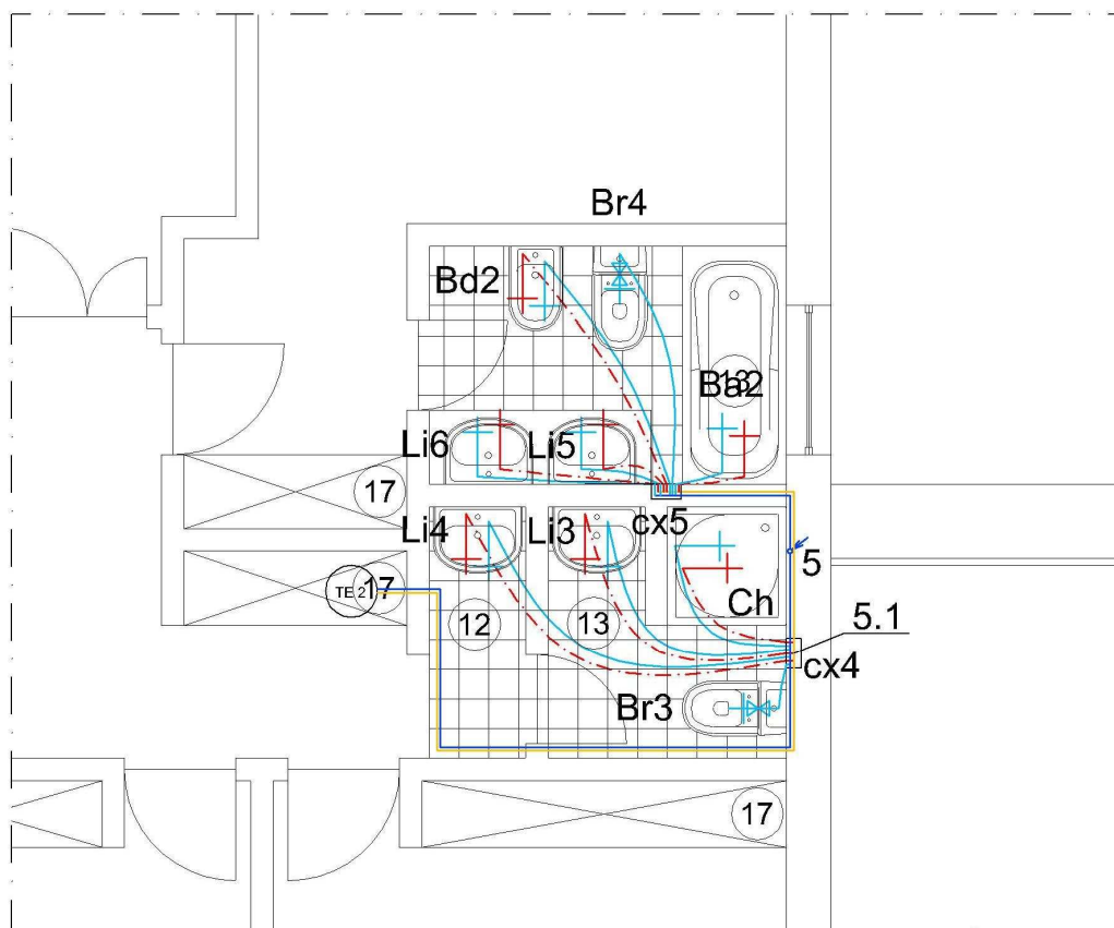
Figura B1.6: HIPÓTESE 0 – Pormenor do WC da cave
