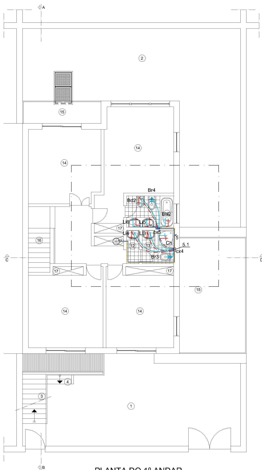
PLANTA DO 1º ANDAR
