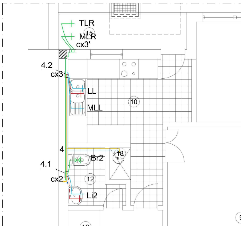
Figura B2.8: HIPÓTESE I – Pormenor da cozinha
