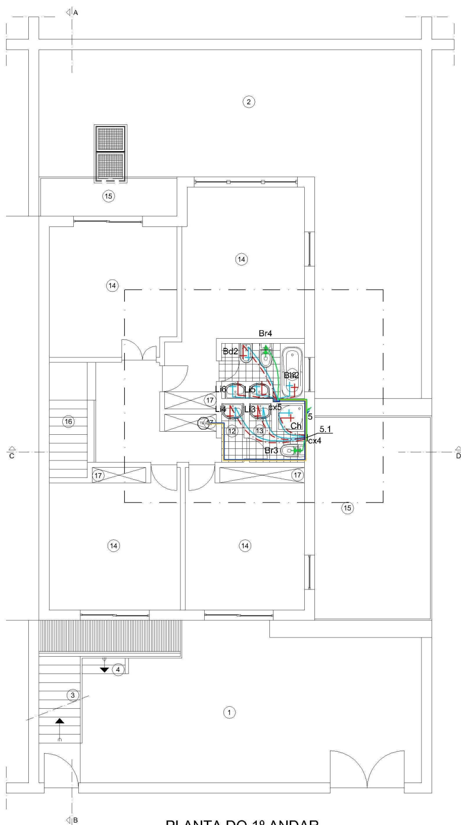
Figura B2.3: HIPÓTESE I – Planta do 1º andar
