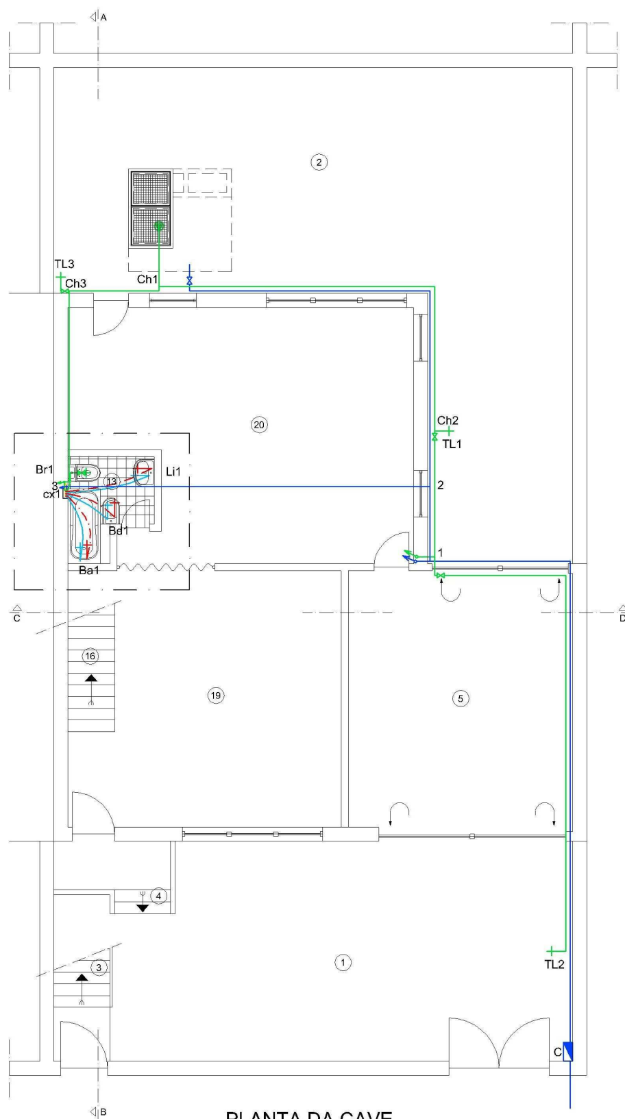
PLANTA DA CAVE
