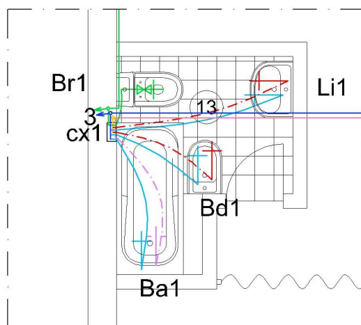
Figura B3.6: HIPÓTESE II – Pormenor do WC da cave
