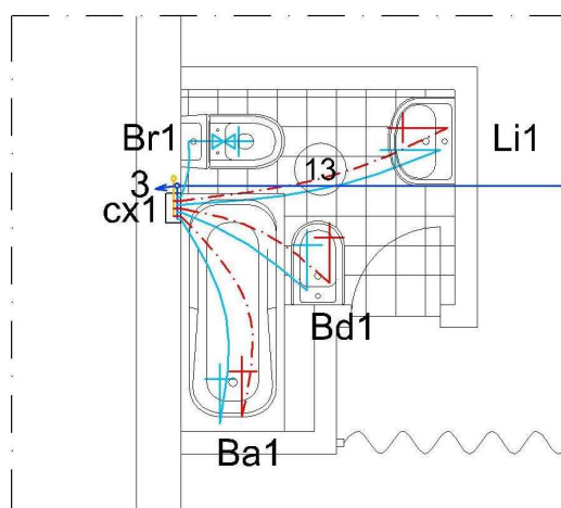
Figura B1.6: HIPÓTESE 0 – Pormenor do WC da cave
