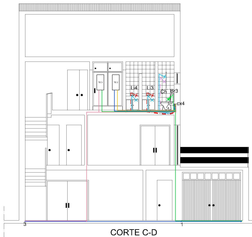
Figura B3.5: HIPÓTESE II – Corte C-D
