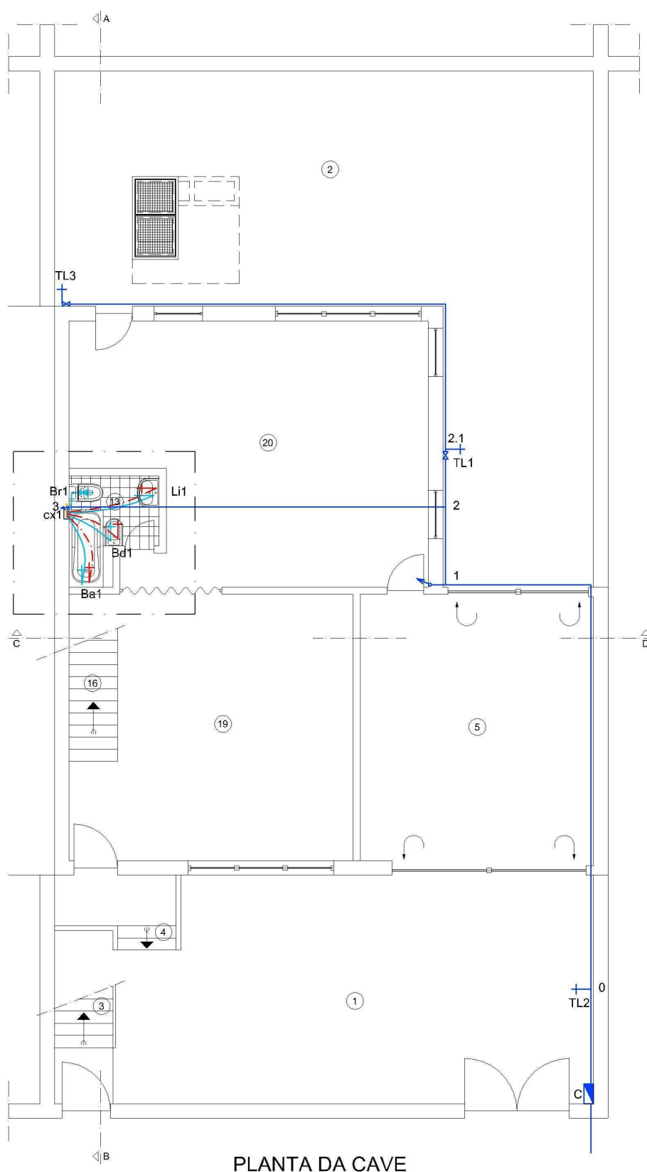
Figura B1.1: HIPÓTESE 0 – Planta da cave
