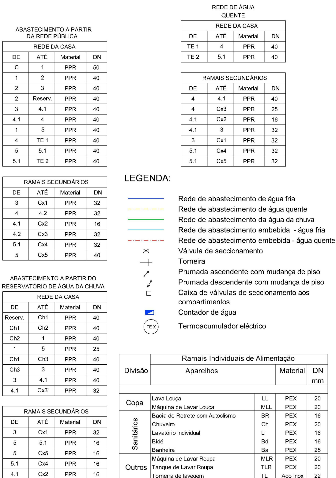
Figura B2.9: HIPÓTESE I – Legenda e quadros de dimensionamento
