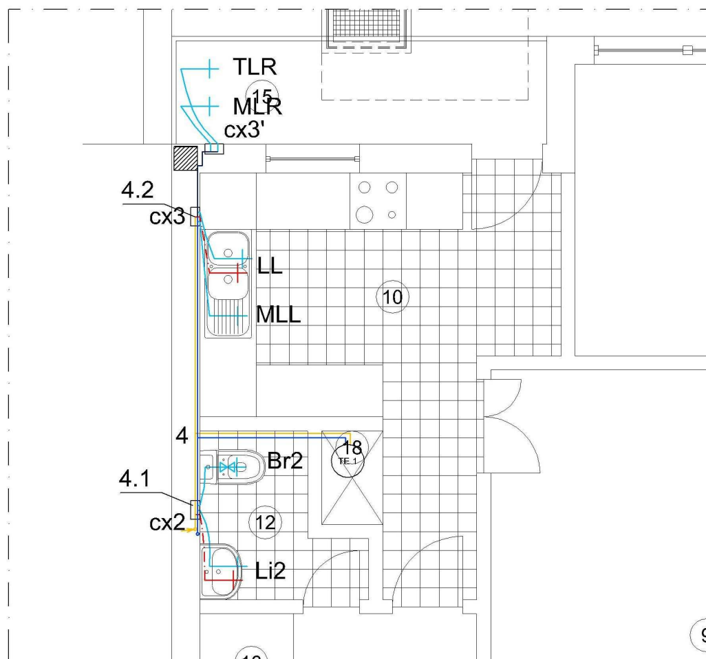
Figura B1.8: HIPÓTESE 0 – Pormenor da cozinha
