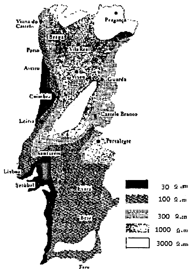
Figura 3.6 - Resistividade média do solo em Portugal [1].
