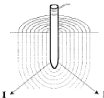
Figura 2.1 - Constituição genérica de uma ligação à terra.
