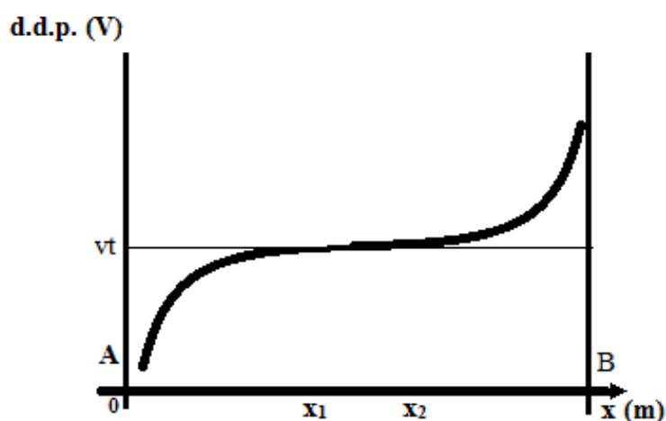
Figura 4.20 - Perfil do potencial na superfície do solo.
