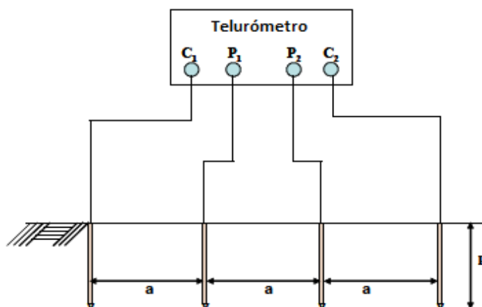
Figura 3.8 - Método de Wenner: aplicação do método.
