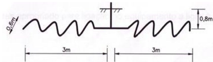
Figura 4.7 - Serpentina dupla [13].
