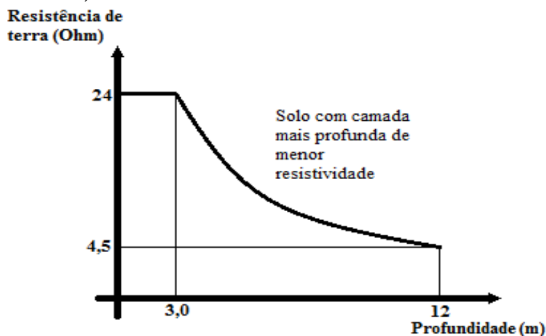
Figura 4.27 - Resistência de terra de um electrodo vertical em função da profundidade de colocação do mesmo, para um solo com uma camada inferior de menor resistividade.
