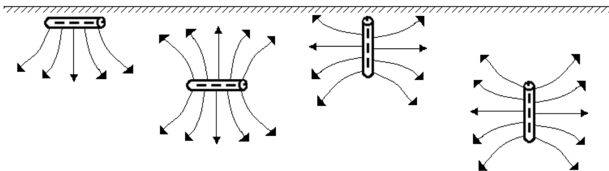
Figura 5.2 - Distribuição da corrente no solo para diferentes profundidades e diferentes disposições.
