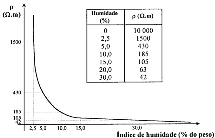
Figura 3.2 - Efeito da humidade na resistividade do solo [1].
