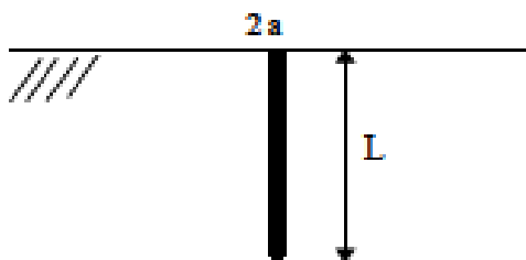
Figura 4.2 - Eléctrodo Vertical.
