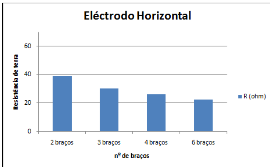
Figura A.9 - Resistência de terra do eléctrodo horizontal em função do número de braços.
