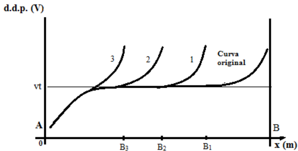
Figura 4.21 - Variação do perfil do potencial em função da distância entre eléctrodos de corrente [1].
