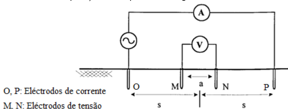
Figura 3.9 - Método de Schlumberger: aplicação do método.
