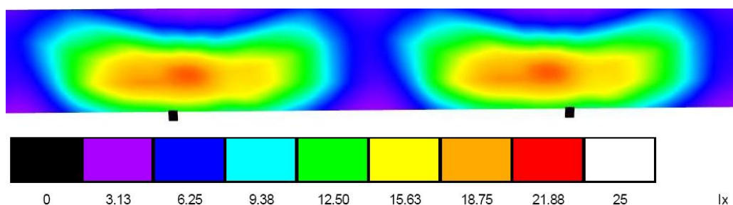
Figura 4.4 - Representação em cores falsas distribuição de iluminância “Coluna Solar”
