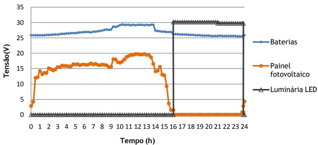
Figura 4.5 - Evolução da tensão em função do tempo “Coluna Solar”
