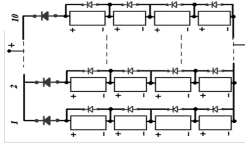
Figura 2.9 - Ligação de diodos de bloqueio [5]
