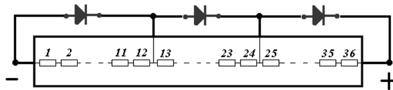
Figura 2.8 - Ligação de díodos de passo [5]
