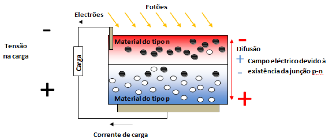
Figura 2.1 - Efeito fotovoltaico
