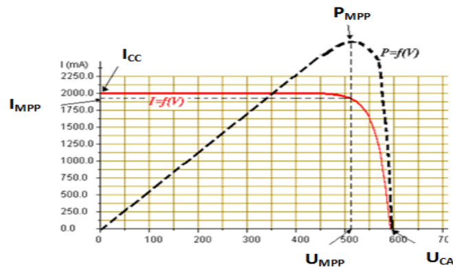
Figura 2.4 - Curvas características de uma célula fotovoltaica [adaptado de 5]
