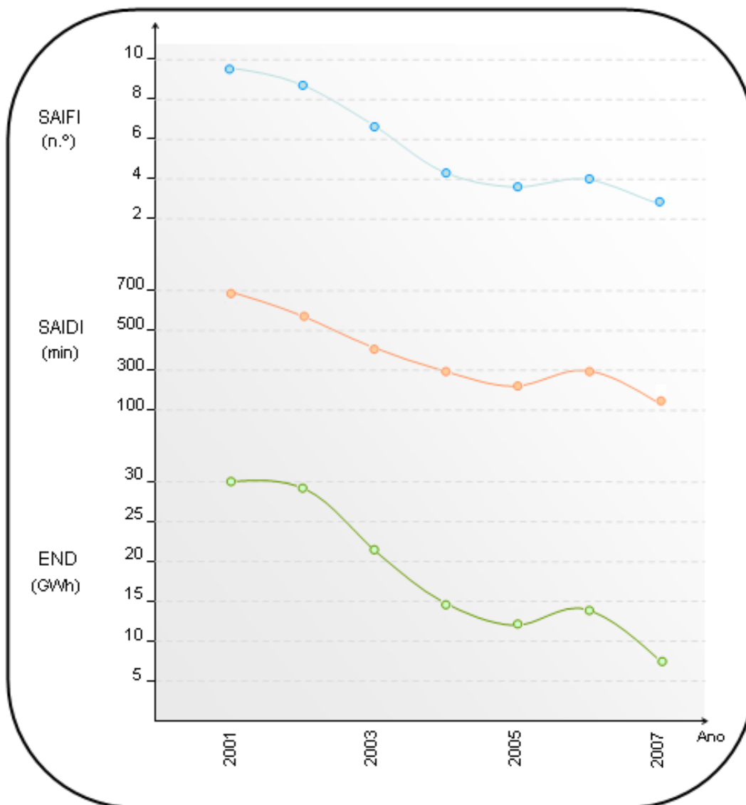
Figura 3.4 - Evolução dos índices SAIFI, SAIDI e END da rede de distribuição de média tensão da EDP na última década
