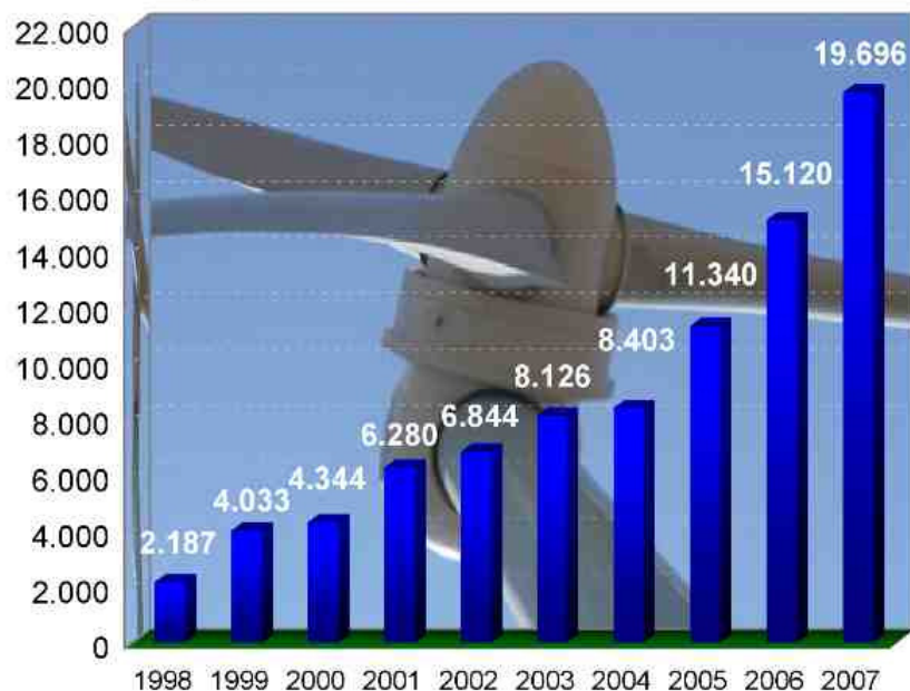
Figura 4 – Produção (em Mw) de novos aerogeradores nos últimos 10 anos
