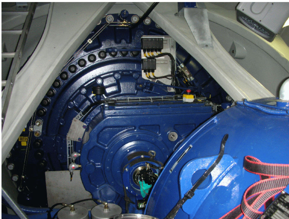
Figura 39 - Reparação na caixa de velocidades de um aerogerador
