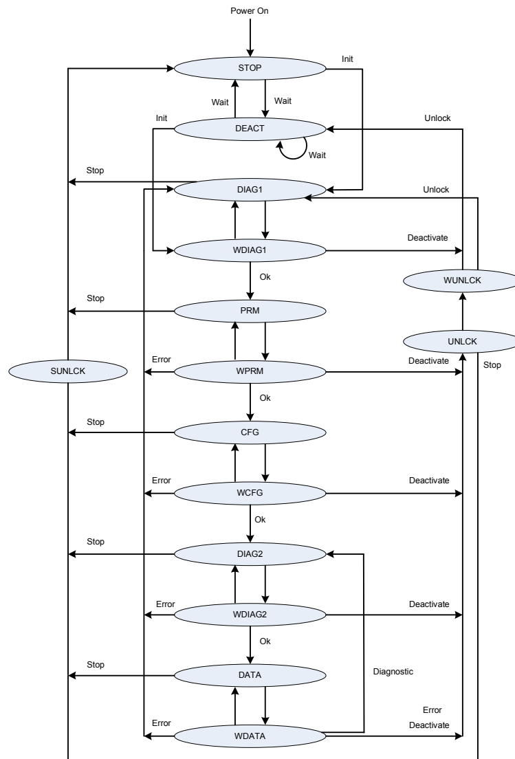
Figura 4.9 - Máquina de estados do módulo slave handler .
