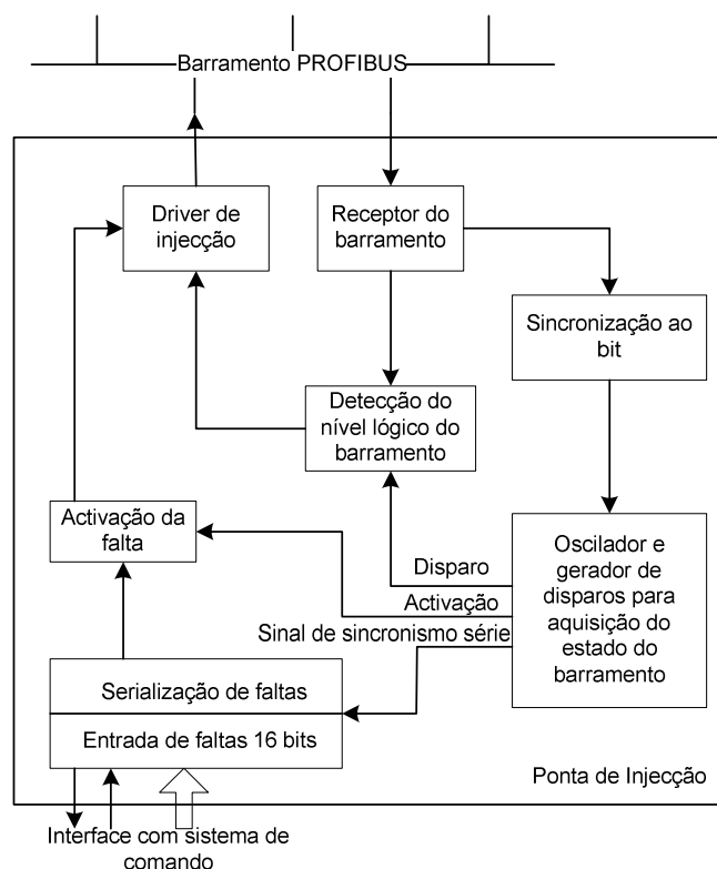
Figura 4.15 - Diagrama funcional da ponta de injeção de falhas.
