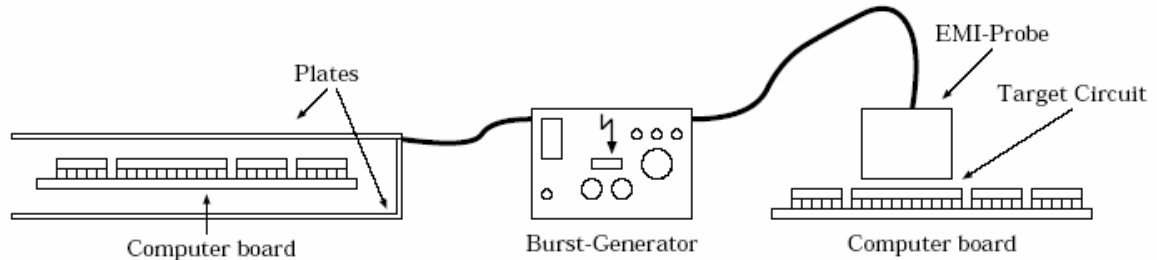
Figura 3.7 - Ferramenta de injeção de falhas por interferência electromagnética.
