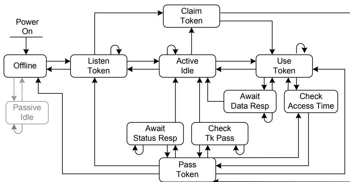
Figura 5.1 - Máquina de estados do controlo de acesso ao meio de uma estação activa PROFIBUS-DP.
