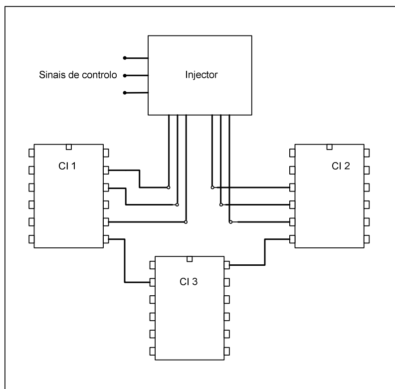
Figura 3.5 - Injector de falhas implementando a técnica de inserção de sinal.
