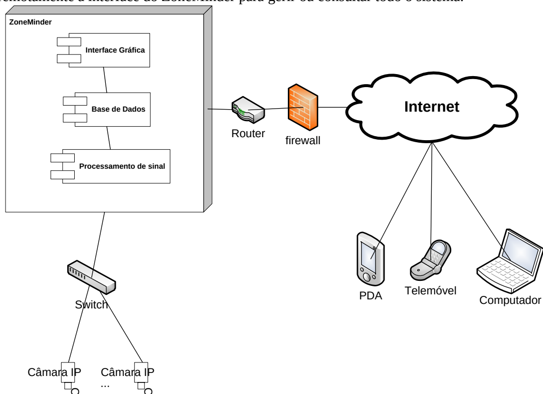
Fig. 28 - Arquitectura física
