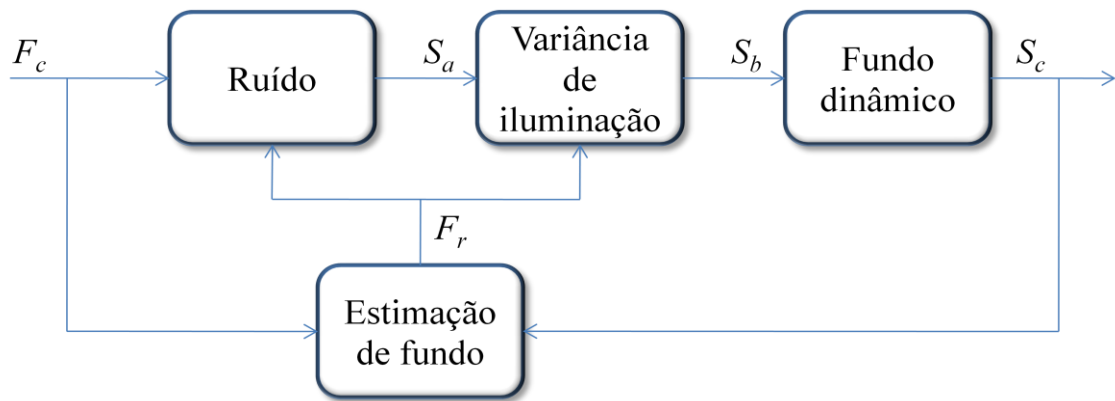
Fig. 31 - Diagrama de blocos do CMoG. (Teixeira et al., 2007)
