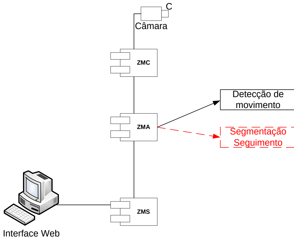
Fig. 32- Diagrama de componentes da implementação.
