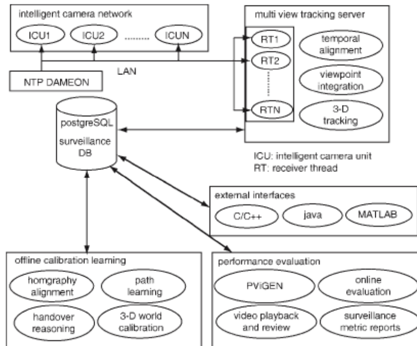
Fig. 5- Arquitectura de um sistema multi-câmara proposto por MaKris e tal. (2004).
