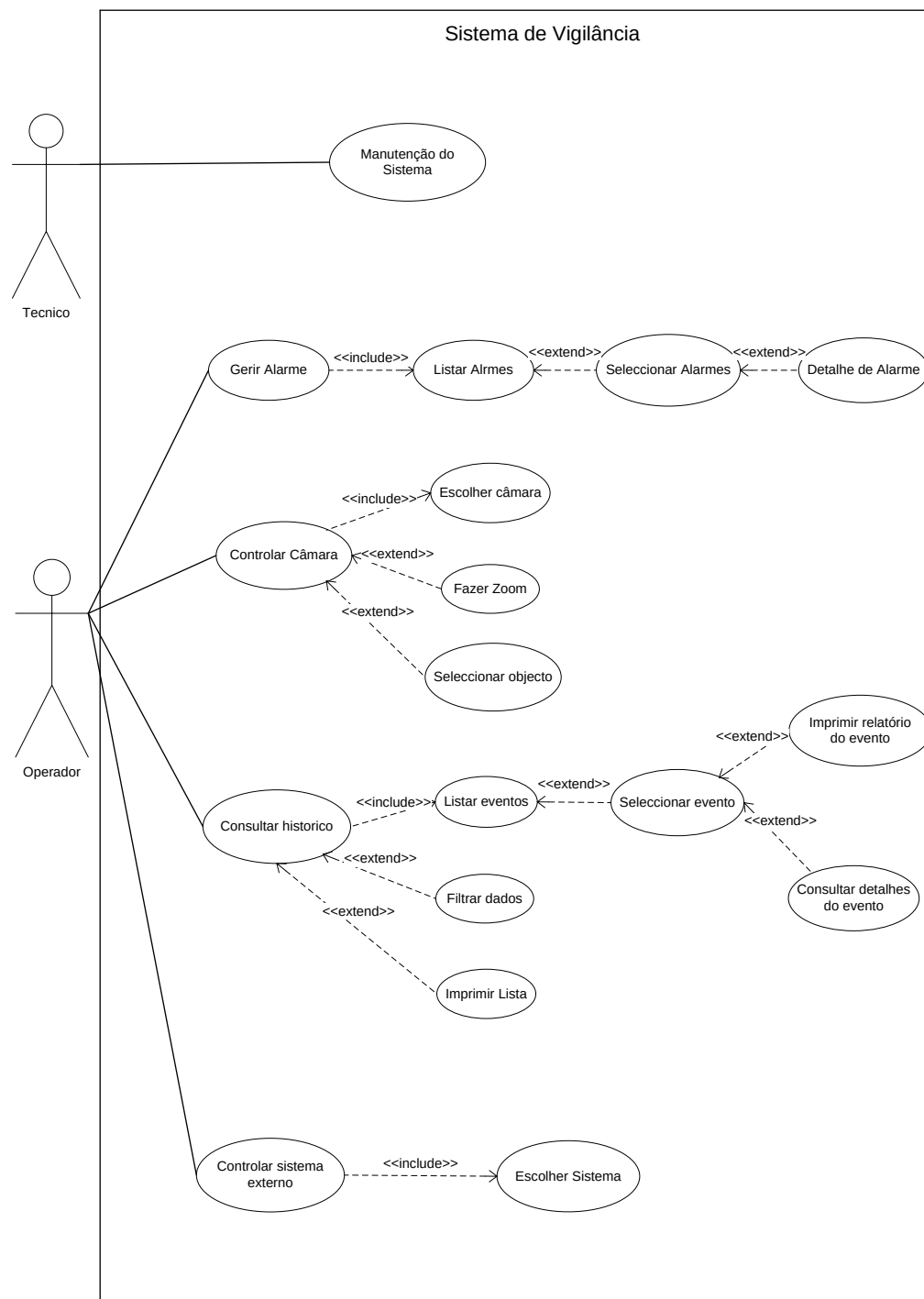
Fig. 15 - Diagrama de Casos de Utilização.
