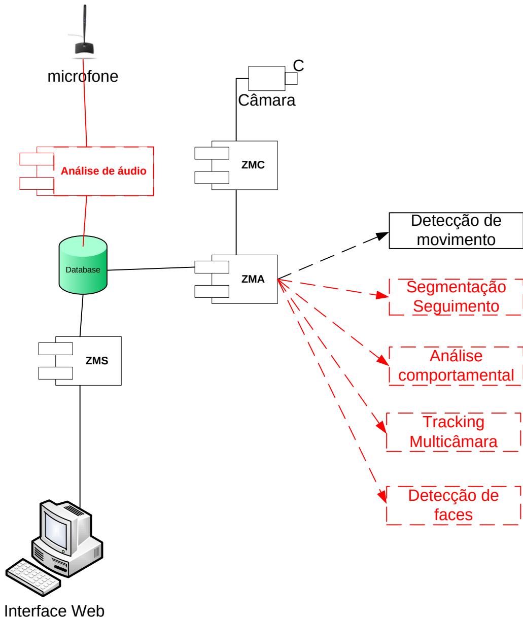
Fig. 33- Diagrama de componentes do trabalho a desenvolver no futuro.
