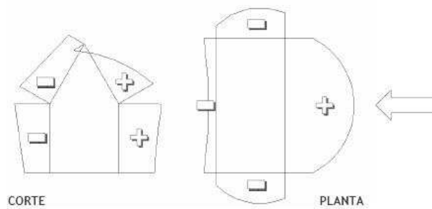
Figura 2.64: Esquema representativo da distribuição de pressões ao longo de um edifício com cobertura de duas águas inclinadas a 60° e vento incidente normal a uma fachada. Os sinais + representam zonas de sobrepressão e os sinais – zonas de subpressão [62].
