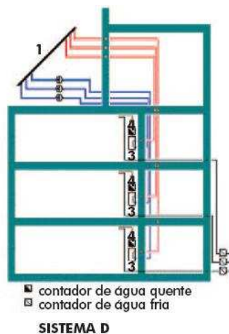
Figura 2.42: Esquema de um sistema monobloco [39].
