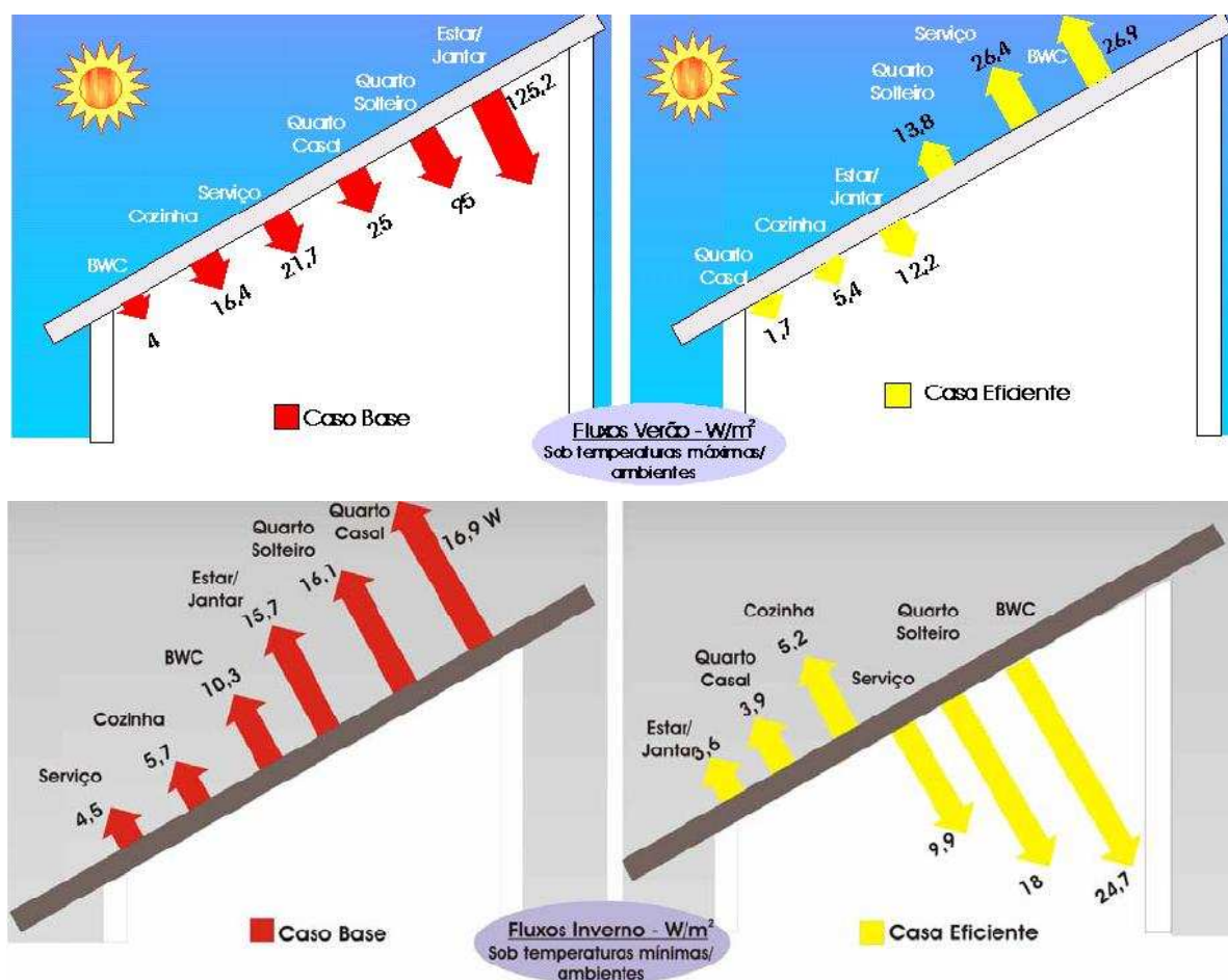
Figura 4.50: Fluxo de calor através da cobertura para diferentes ambientes, no modelo base e no modelo 10. Em cima: situação de Verão, em baixo: situação de Inverno. Os valores apresentados são em W/m^2 [85].
