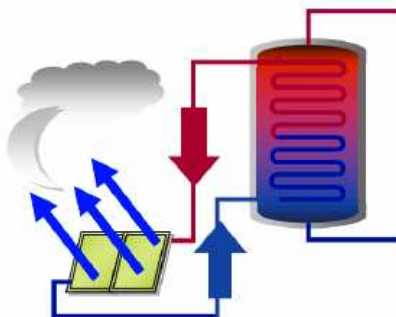
Figura 2.38: Esquema de circulação invertida em sistema de termossifão [40].
