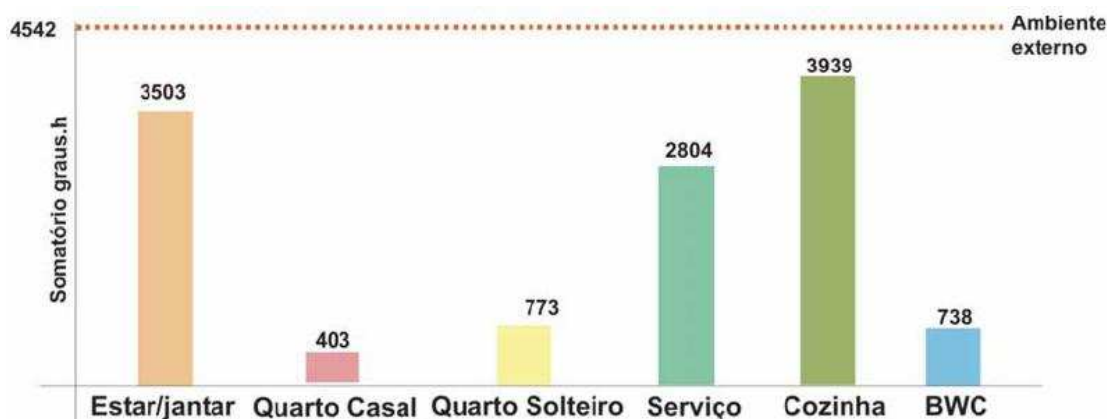
Figura 4.53: Somatório de graus.h necessários para arrefecimento, situação de Verão [85].
