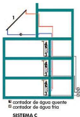
Figura 2.41: Esquema de um sistema de colectores centralizado [39].
