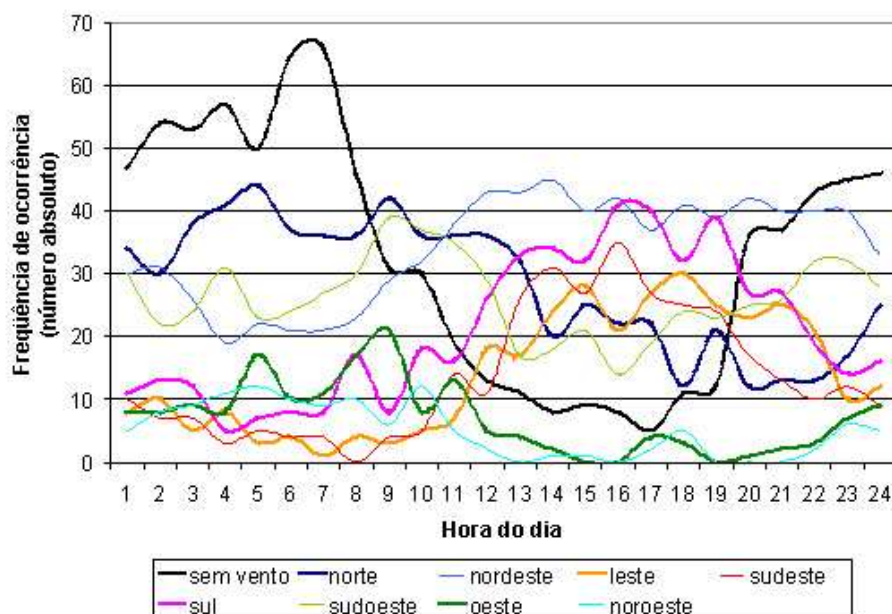
Figura 4.7: Frequência dos ventos segundo a direcção, para diferentes horas do dia. Dados relativos ao TRY [81].
