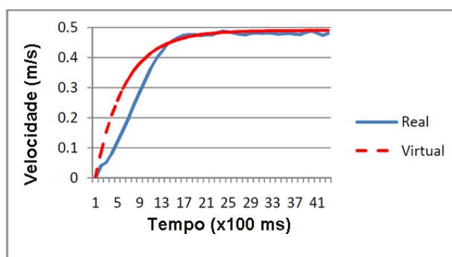
Figura 107: Curva de aceleração da cadeira de rodas real e virtual
