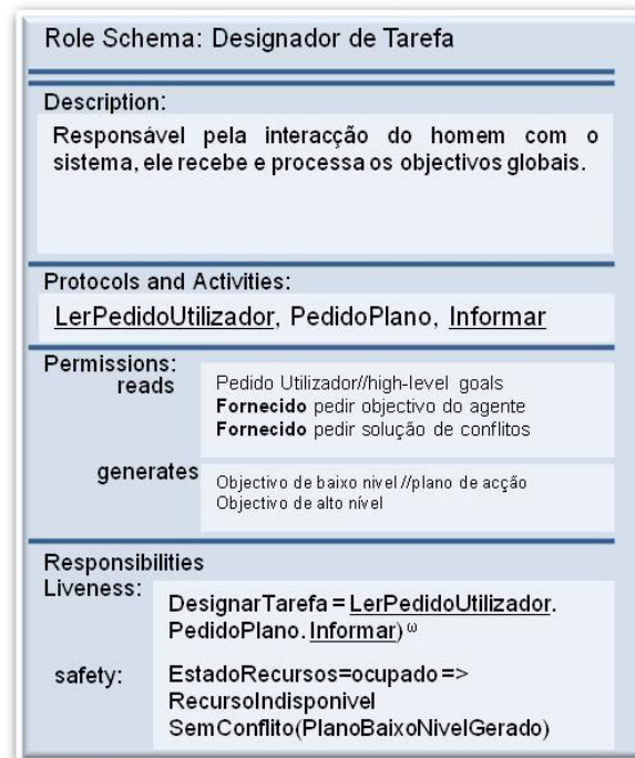
Figura 97: Papel Designador de tarefas
