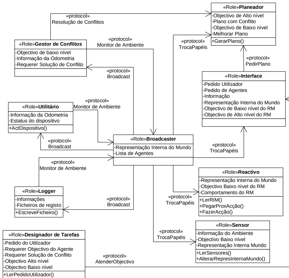
Figura 104: Diagrama dos papéis e interação
