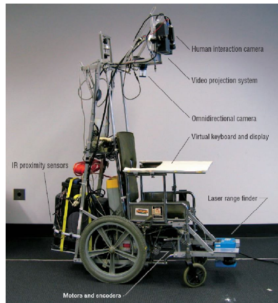
Figura 32: Protótipo Smartchair
