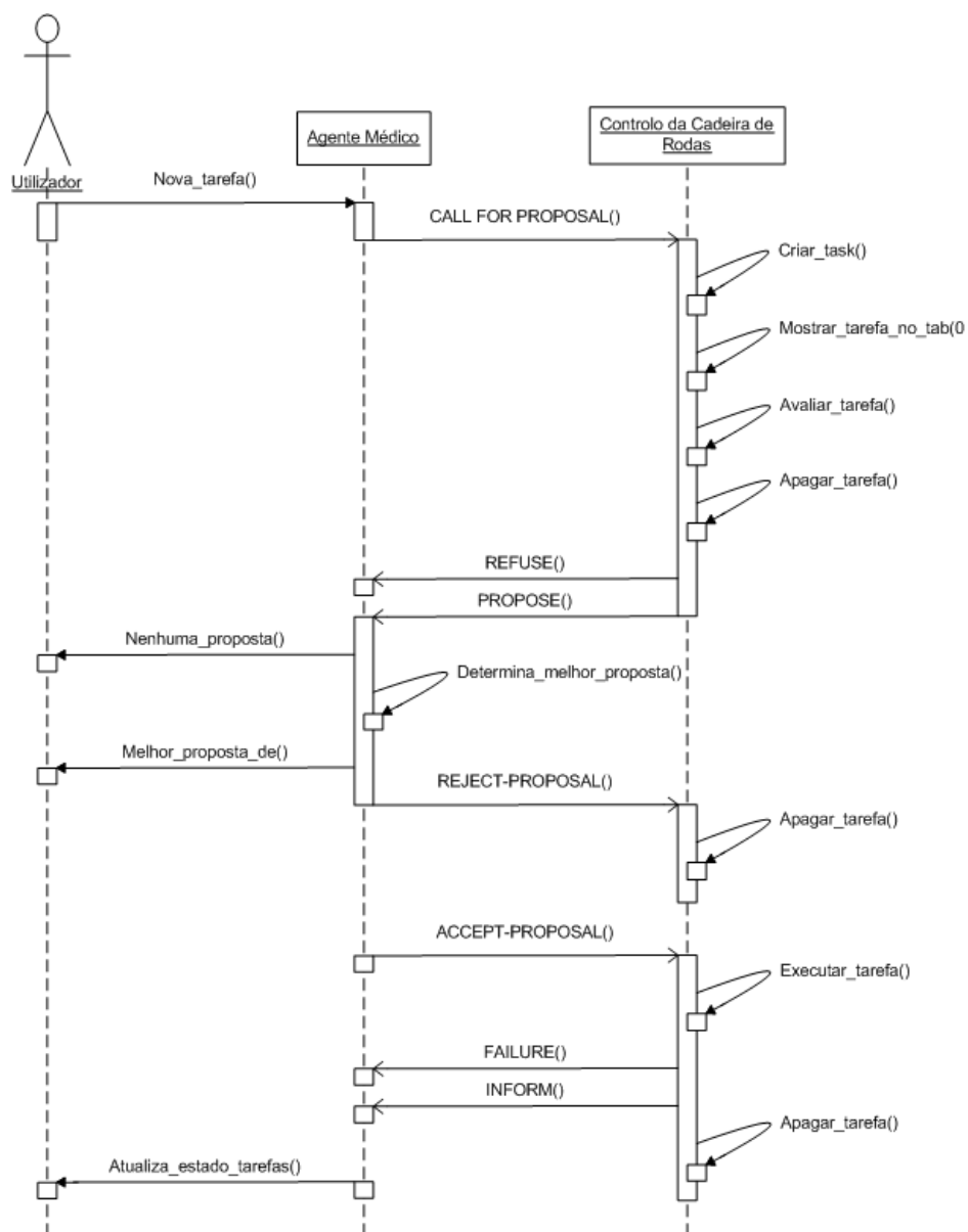
Figura 129: Diagrama de interacção entre os agentes Médico x Controlo
