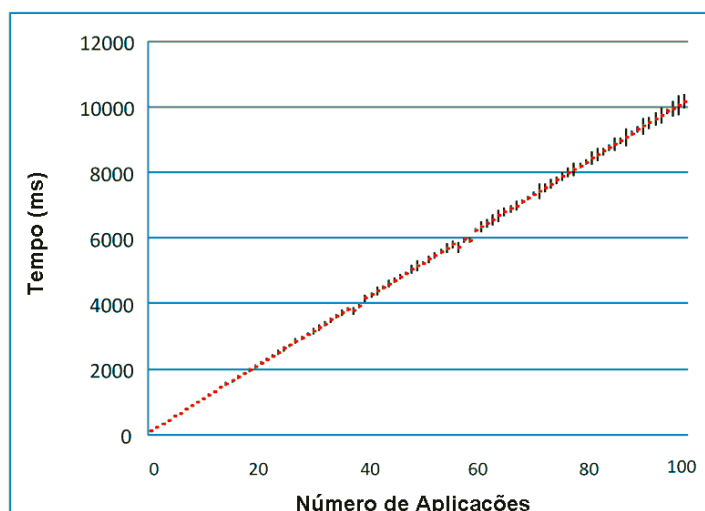
Figura 139: Tempo necessário para reunir todas as informações dos aplicativos e criar uma nova LAL
