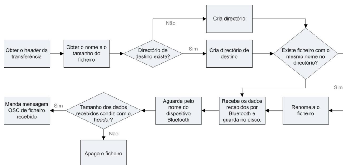
Figura 4.2 - Flowchart da class BTRquestHandler
