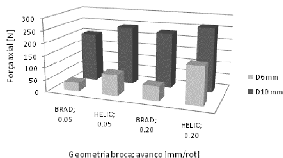
Figura 11a – Variação da força axial máxima em função do diâmetro da broca, geometria da broca e avanço.
