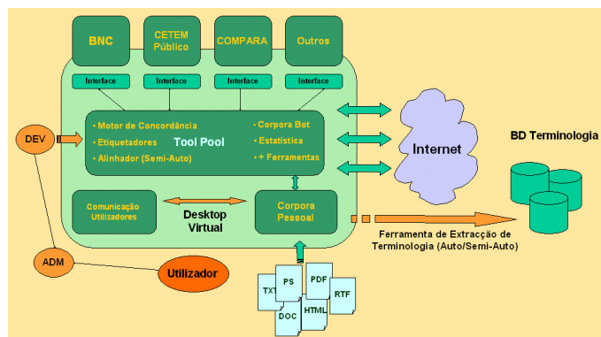
Figura 1 – A arquitectura geral do Gestor de Corpora
