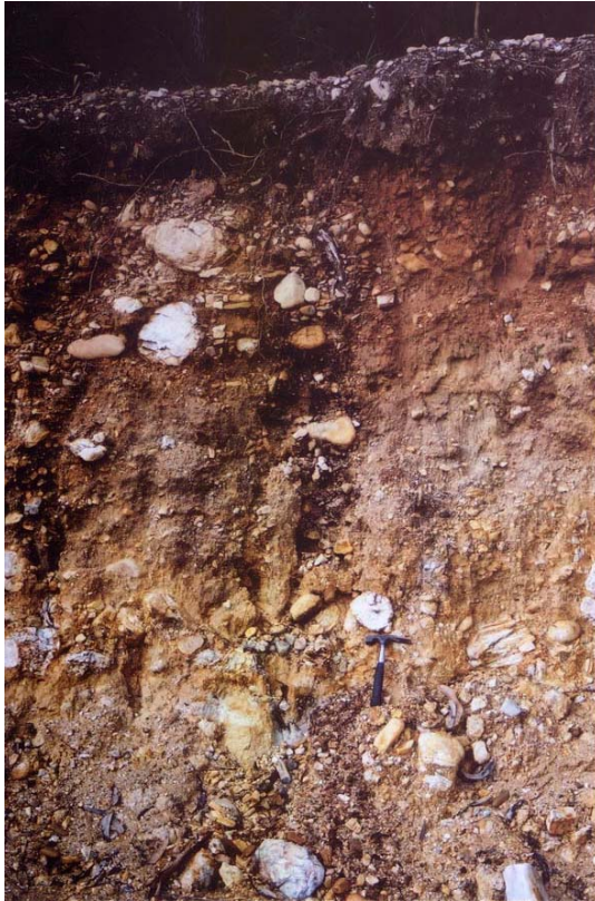
Fig. 4 – Depósito conglomerático que constitui uma pequena elevação no fundo da depressão de Soutelo. Fig. 4 – Conglomeratic deposit that formed a little hill on Soutelo's depression.
