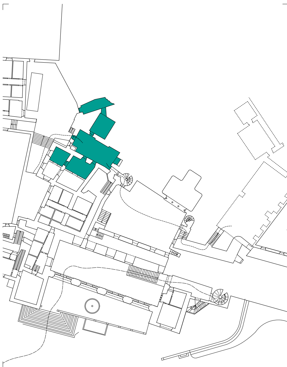
[Fig. 49] Planta parcial do piso à cota do Pátio do Leão do Palácio Real da Vila de Sintra (c. 1905), desenho da autora, 2024. Escala 1/500.
