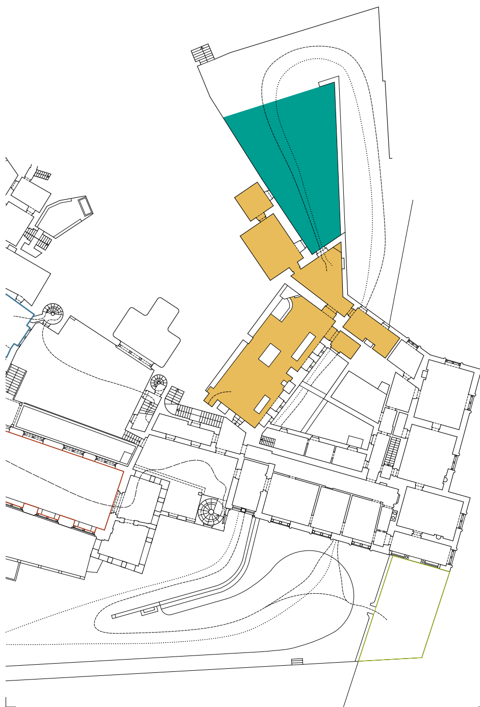
[Fig. 36] Planta parcial do piso nobre do Palácio Real da Vila de Sintra (c. 1905). Escala 1/500. Desenho da autora.
