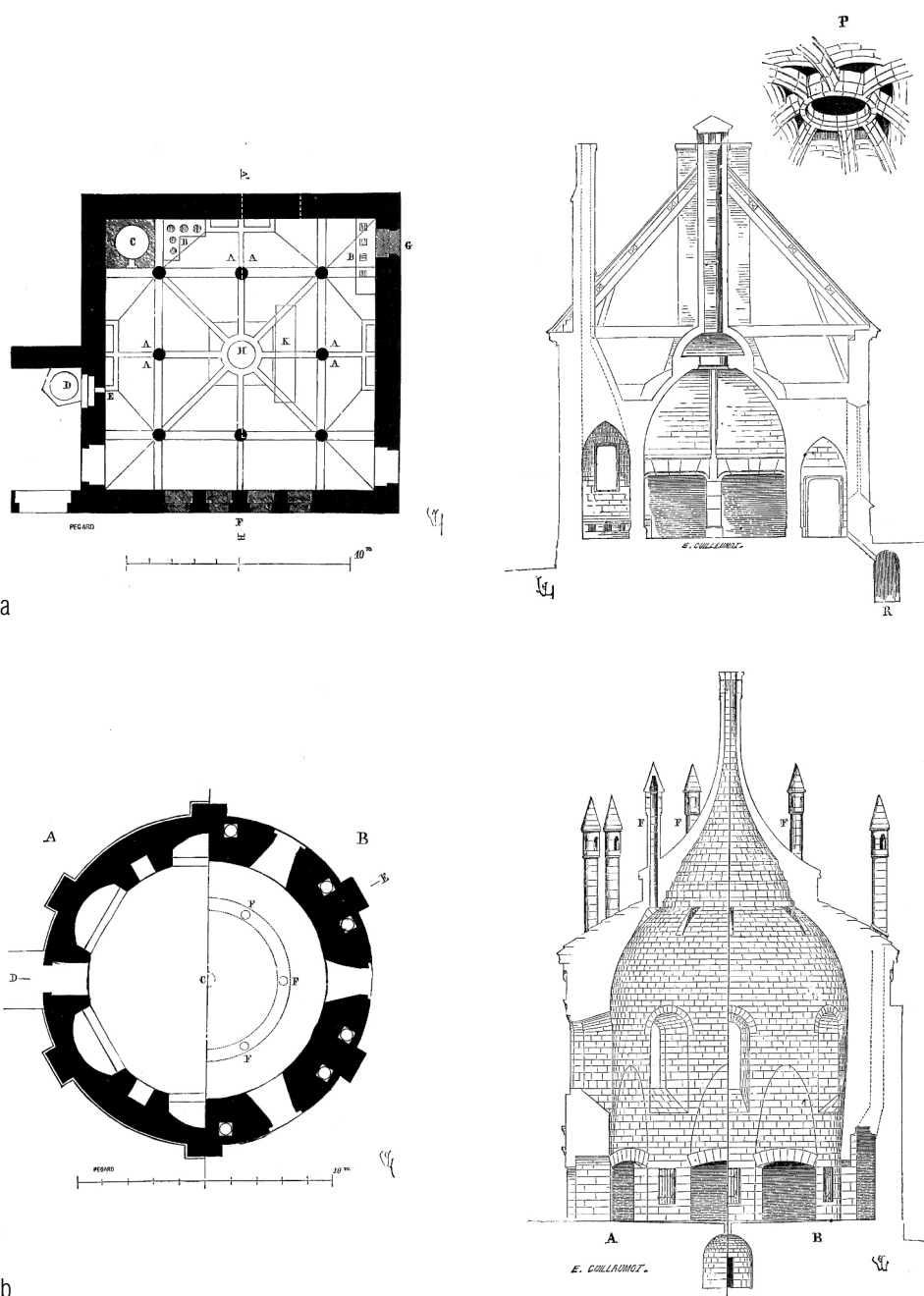
[Fig. 37] a – Planta e secção do volume da cozinha do Palácio dos Duques de Borgonha; b – Planta e secção do volume da cozinha da Abadia de Vendôme. Gravuras patententes na obra Espinet, M. (1984). El Espacio Culinario. De la taberna romana a la cocina profesional y doméstica del siglo XX . Tusquets Editores, pp. 55-57 e pp. 38-39, respetivamente.
