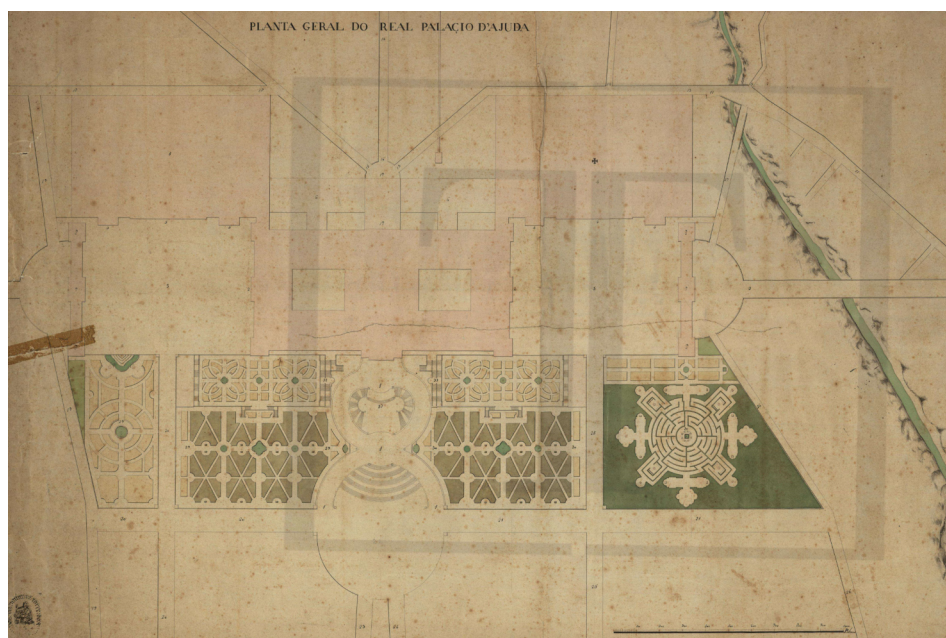
[Fig. 42] Planta do piso térreo do Palácio Real da Ajuda, Nicolau Pires (-), 1838. © ANTT, PT/TT/CR/E/001007-001/00054, Casa Real, Plantas, Almoxarifado da Ajuda, n.º 54.
