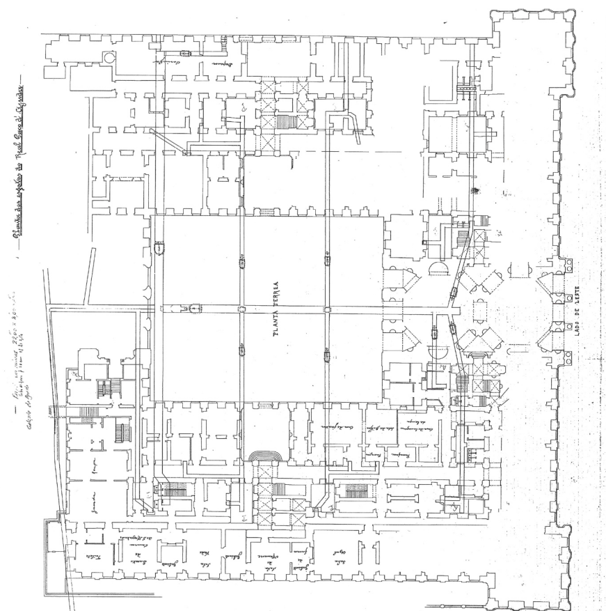
[Fig. 72] Planta do túnel sob o pátio central do Palácio Real da Ajuda, autor desconhecido, c. 1875. © ANTT, PT/TT/CR/E/001007-001/00088, Casa Real, Plantas, Almocharifado da Ajuda, n.º 88.
