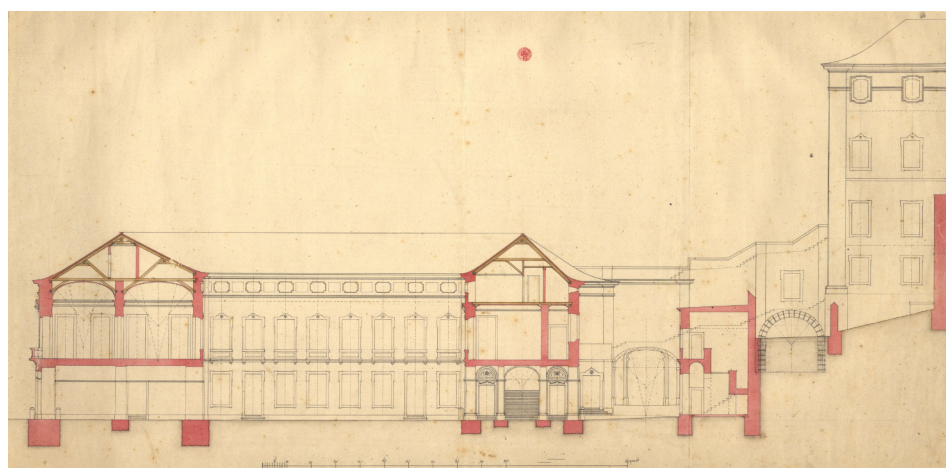
[Fig. 13] Planta dos aquedutos e canalizações que distribuem água aos diversos pontos na Real Quinta e Palácio Real das Necessidades, autor desconhecido, datação desconhecida. © ANTT, PT-TT-CR-007-008-00219, Casa Real, Plantas, Almojarifado das Necessidades, n.º 219.
