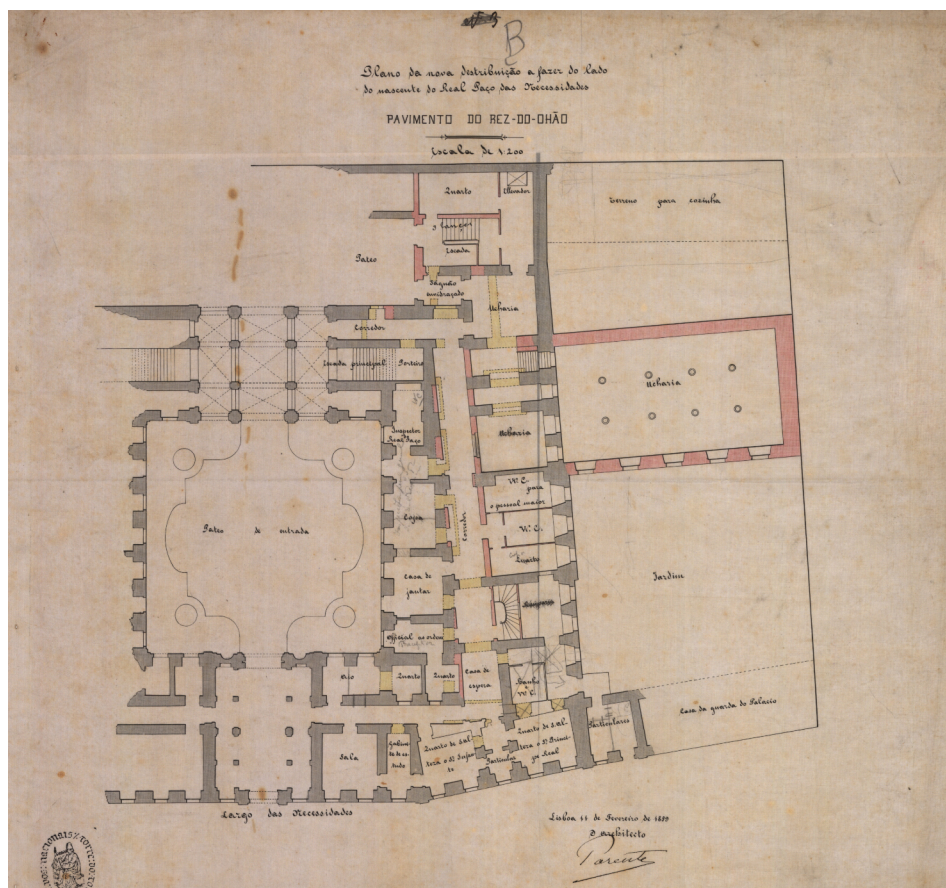
[Fig. 46] Planta do piso nobre do Palácio Real das Necessidades, Domingos Parente da Silva (1836-1901), 1899. © ANTT, PT-TT-CR-007-008-00246, Casa Real, Plantas, Almojarifado das Necessidades, n.º 246.
