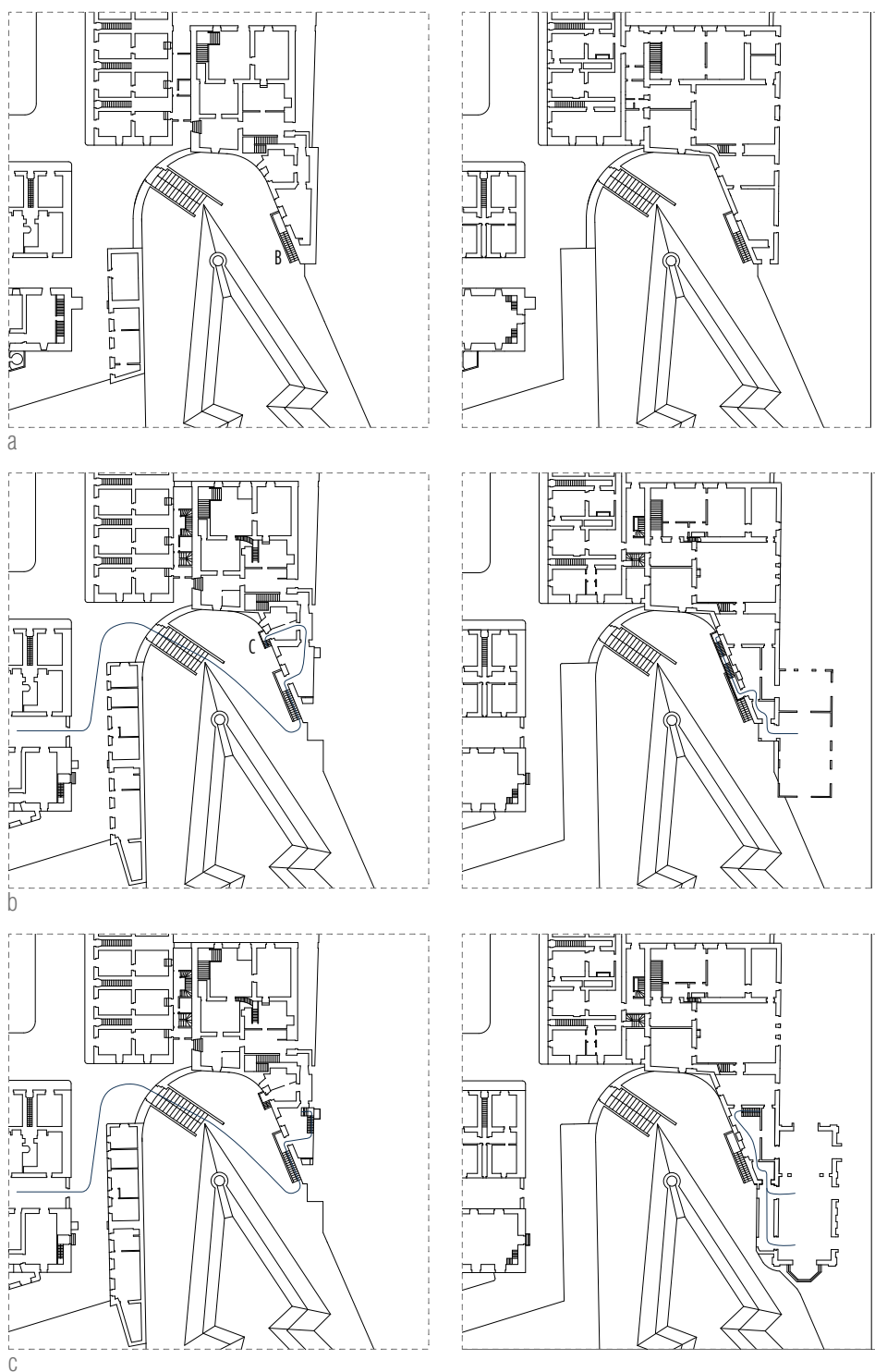
[Fig. 41] Proposta para a evolução da arquitetura dos pisos térreo e nobre do Pavilhão de S. Luís, do volume das cozinhas e do Palácio Real da Cidadela de Cascais: comunicação entre cozinha e sala de jantar principal, montagem e desenhos da autora, 2023. Escala 1/1200.
