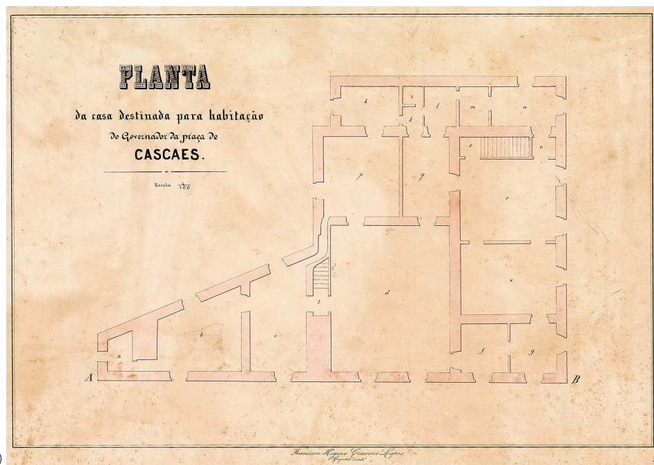
[Fig. 27] Planta da Praça de Cascaes e dos terrenos pertencentes à mesma, J. A. Esteves Vaz (-), 1864. © GEAEM, Direção de Infraestruturas do Exército 1064-1-8-12.
