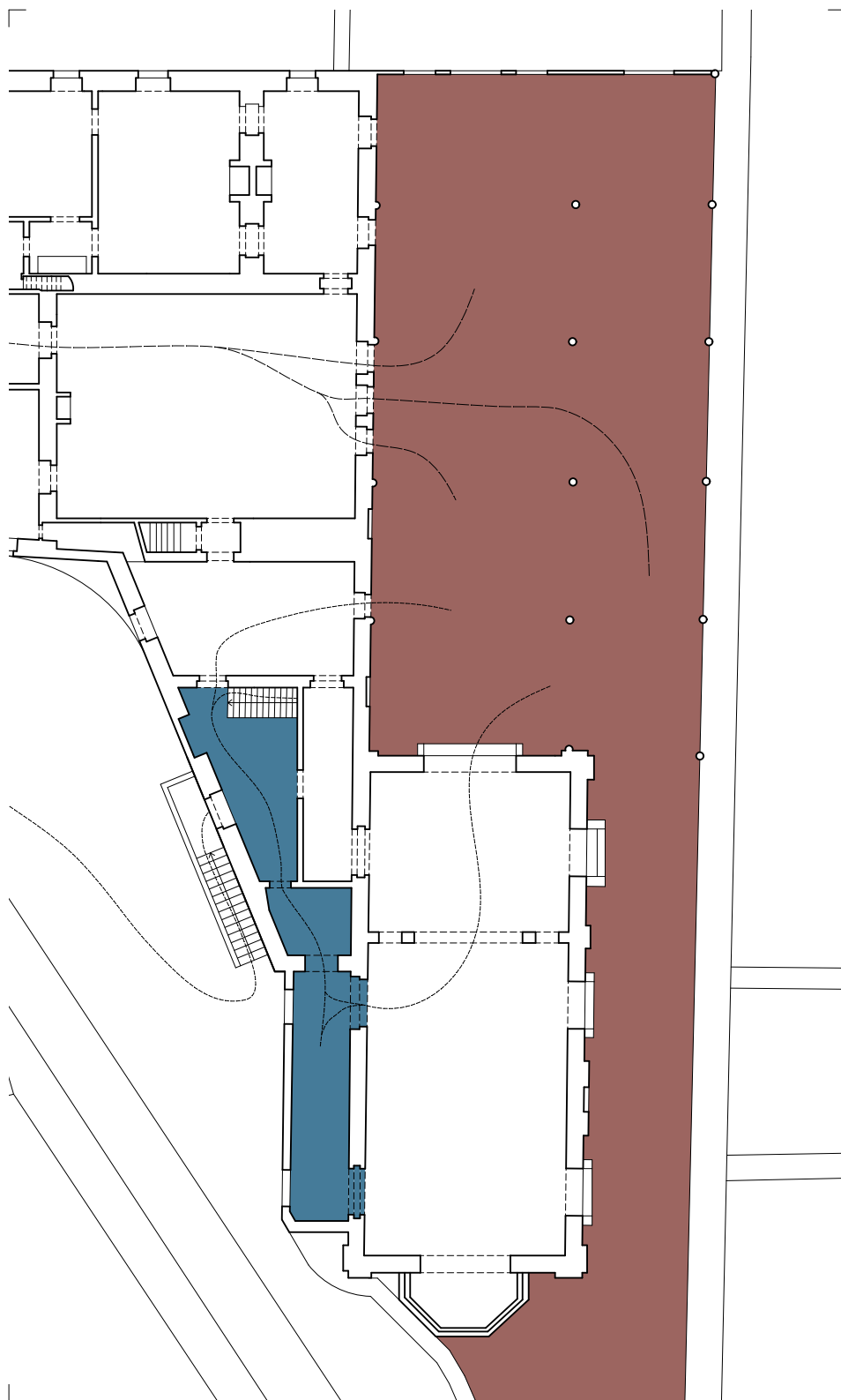
[Fig. 46] Planta parcial do piso nobre do Palácio Real da Cidadela de Cascais: salas de jantar, bilhar e terraço (c. 1900), desenho da autora, 2023. Escala 1/250.
