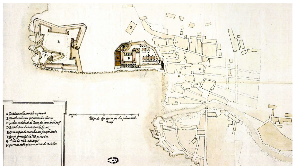
[Fig. 23 – página anterior] Planta da Cidadela e Vila de Cascais , cópia de G. D. C. Weyrother (-), datação presumível do séc. XIX. © GEAEM, Direção de Infraestruturas do Exército 114-6-82-115.
