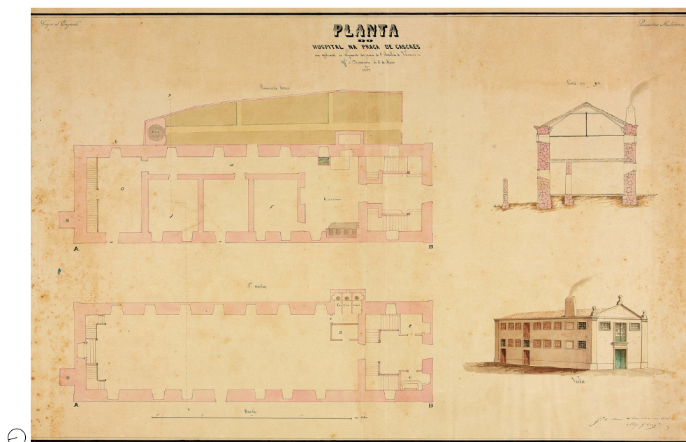
[Fig. 33] Planta da Cidadela de Cascais, Maximiano José da Serra (1750-1834), c. 1796. © GEAEM, Direção de Infraestruturas do Exército 8108-3-43-propria.
