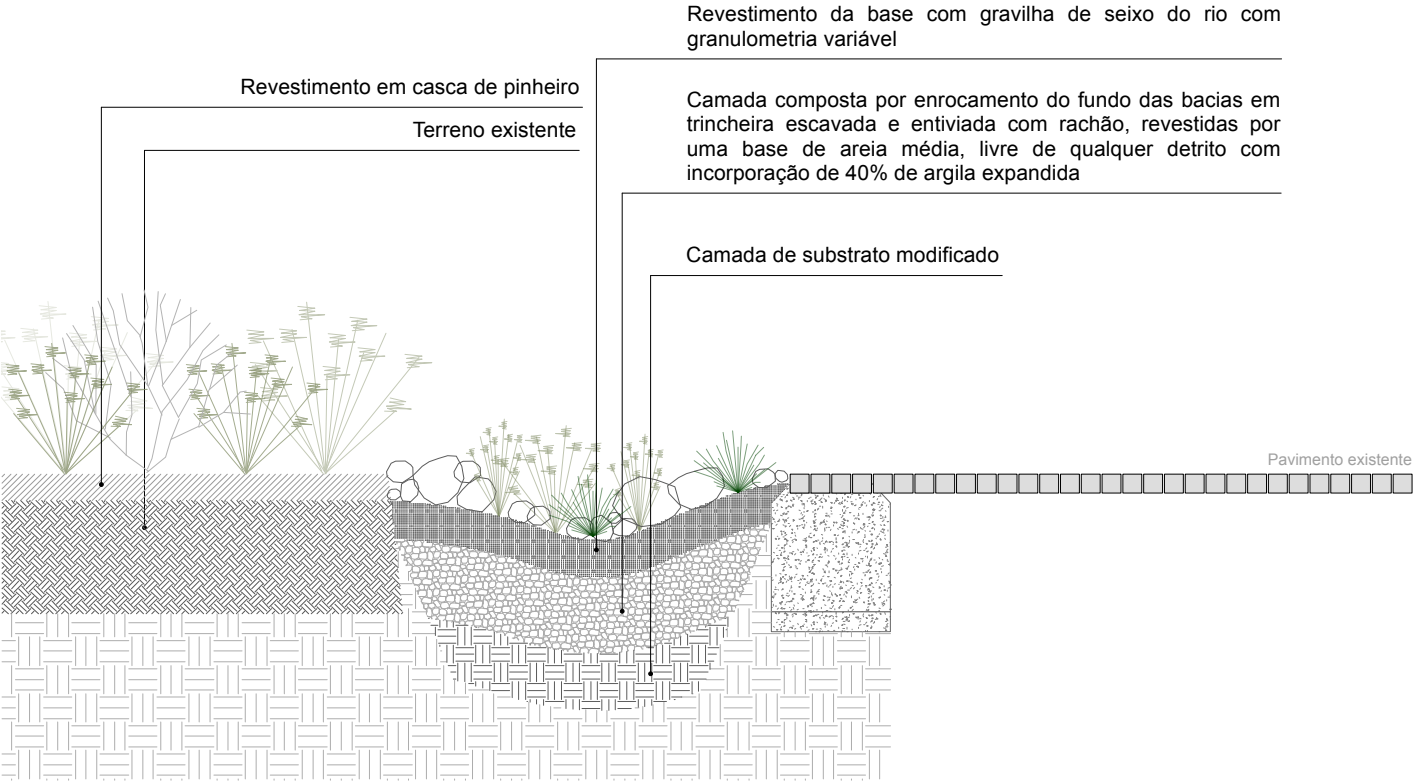
PORMENOR TIPO DE SISTEMA DE DRENAGEM ESCALA 1:20
