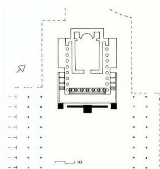
Fig 13. Planta Geral do Templo de Vênus Genetrix (Roma). As fontes consagradas às ninfas estão identificadas a preto. Segundo Ulrich (1986). Fonte: Dylan Rogers (2015, p. 624).
