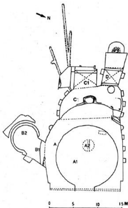
Fig 14. Planta Geral do Ninfeu de Bergantino (Castel Gandolfo). Segundo Letzner (1990). Fonte: Mónica Montoro Castillo (2008, p. 495).
