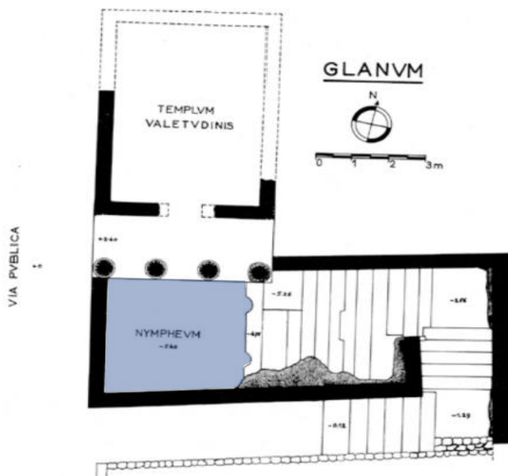
Fig 20. Planta Geral da Fonte de Glanum e Templo de Valetudo (França). Segundo H. Rolland, 1958. Fonte: Dylan Rogers (2015, p. 710).
