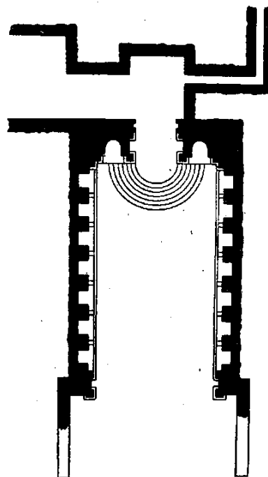
Fig 3. Planta Geral do Ninfeu Dórico (Castel Gandolfo). Segundo Lugli (1913). Fonte: Lucía Gómez Robles (2014, p. 87).
