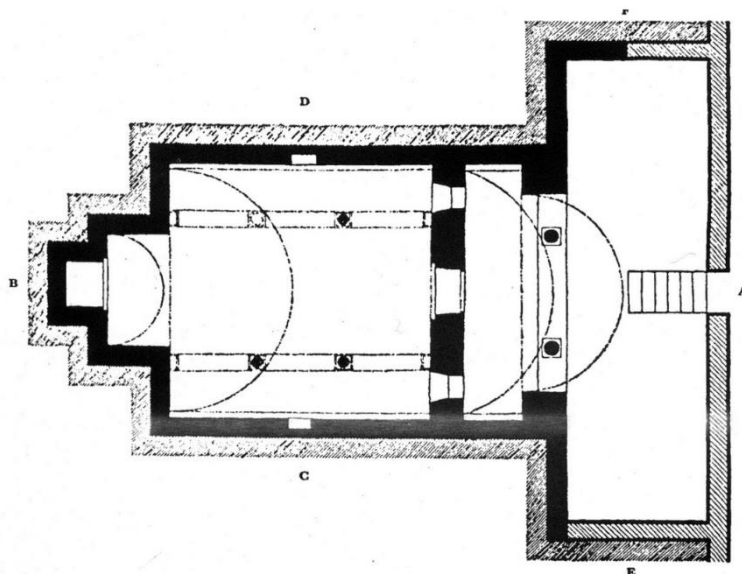
Fig 30. Planta Geral do Templo de Santa Eulália de Bóveda (Lugo). Segundo H. Hanson. Fonte: Mónica Montoro Castillo (2008, p. 192).
