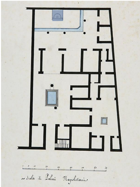
Fig 5. Planta Geral da Casa da Fonte Pequena (Pompeia). Segundo Carlos Bonucci (Séc. XIX). Fonte: Catálogo generale Beni Culturali.
