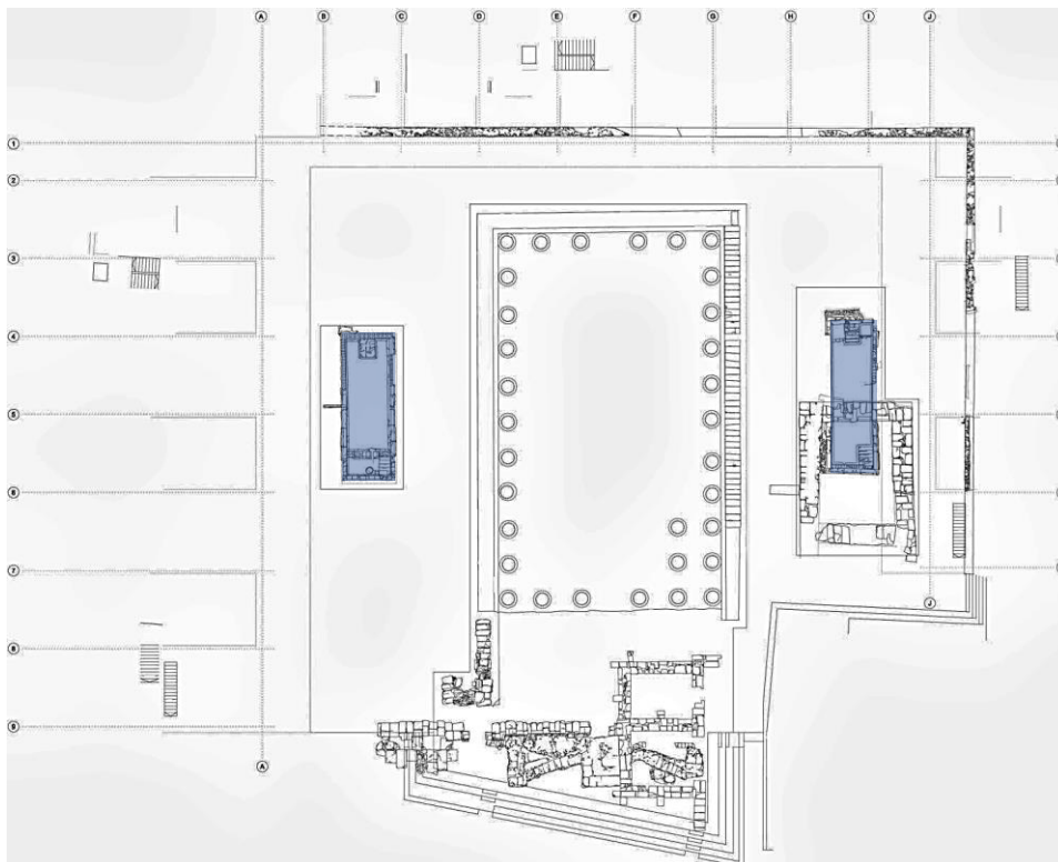
Fig 35. Planta Geral do Templo de Diana (Mérida). Fonte: Arquitecto José Maria Sánchez García, Aib Architecture_Obras.
