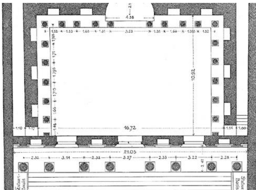
Fig 8. Planta Geral da Biblioteca de Celso (Éfeso). Desenho de W. Wilberg. Fonte: Ferit Cakir (2022, p. 6).
