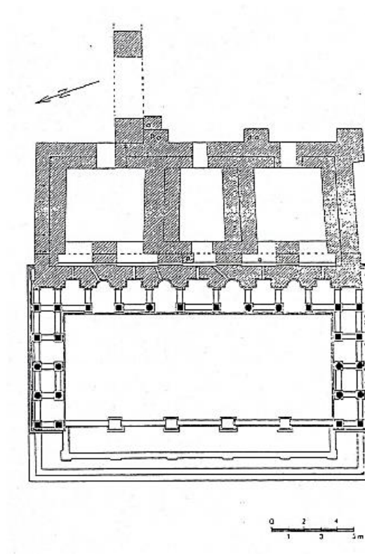
Fig 12. Planta Geral do Ninfeu de Mileto. Segundo J. Hülsen. Fonte: Pierre Gros (1996, p. 480).
