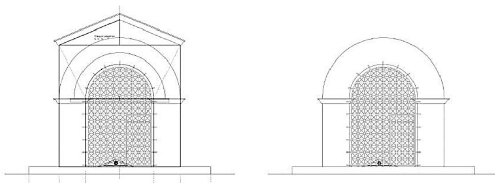
Fig 31. Propostas de Reconstituição do Alçado Principal do Ninfeu das Termas Romanas de Chaves. Fonte: César Figueiredo (2022, p. 234).
