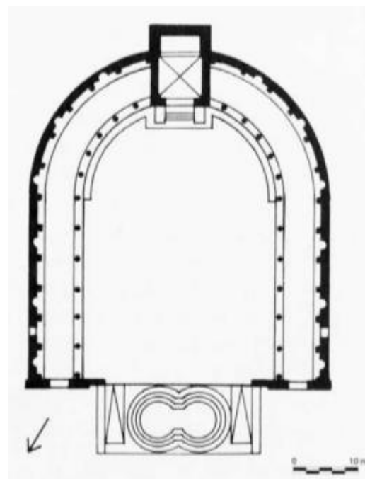
Fig 18. Planta Geral do Templo das Águas (Zaghouan). Segundo B. Longfellow (2011). Fonte: Dylan Rogers (2015, p. 692).
