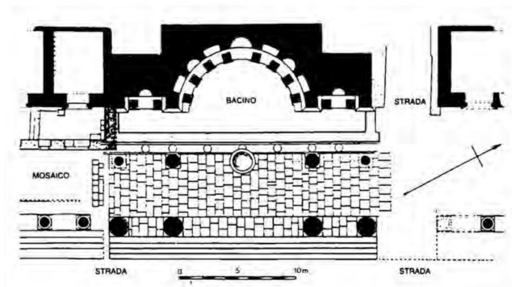
Fig 4. Planta Geral do Ninfeu de Gérasa. Segundo C. S. Fischer. Fonte: Pierre Gros (1996, p. 479).
