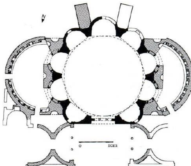
Fig 7. Planta Geral do Templo de Minerva Médica (Roma). Segundo Richardson (1992). Fonte: Mónica Montoro Castillo (2008, p. 140).
