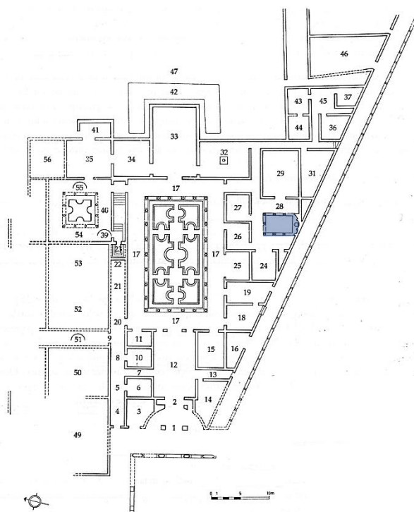
Fig 33. Planta Geral da Casa dos Repuxos (Conímbriga). Fonte: J. M. B. Oleiro (1992, est. 1).
