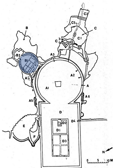
Fig 2. Planta Geral da Gruta de Tibério (Sperlonga). Segundo Letzner (1990). Fonte: Mónica Montoro Castillo (2008, p. 99).
