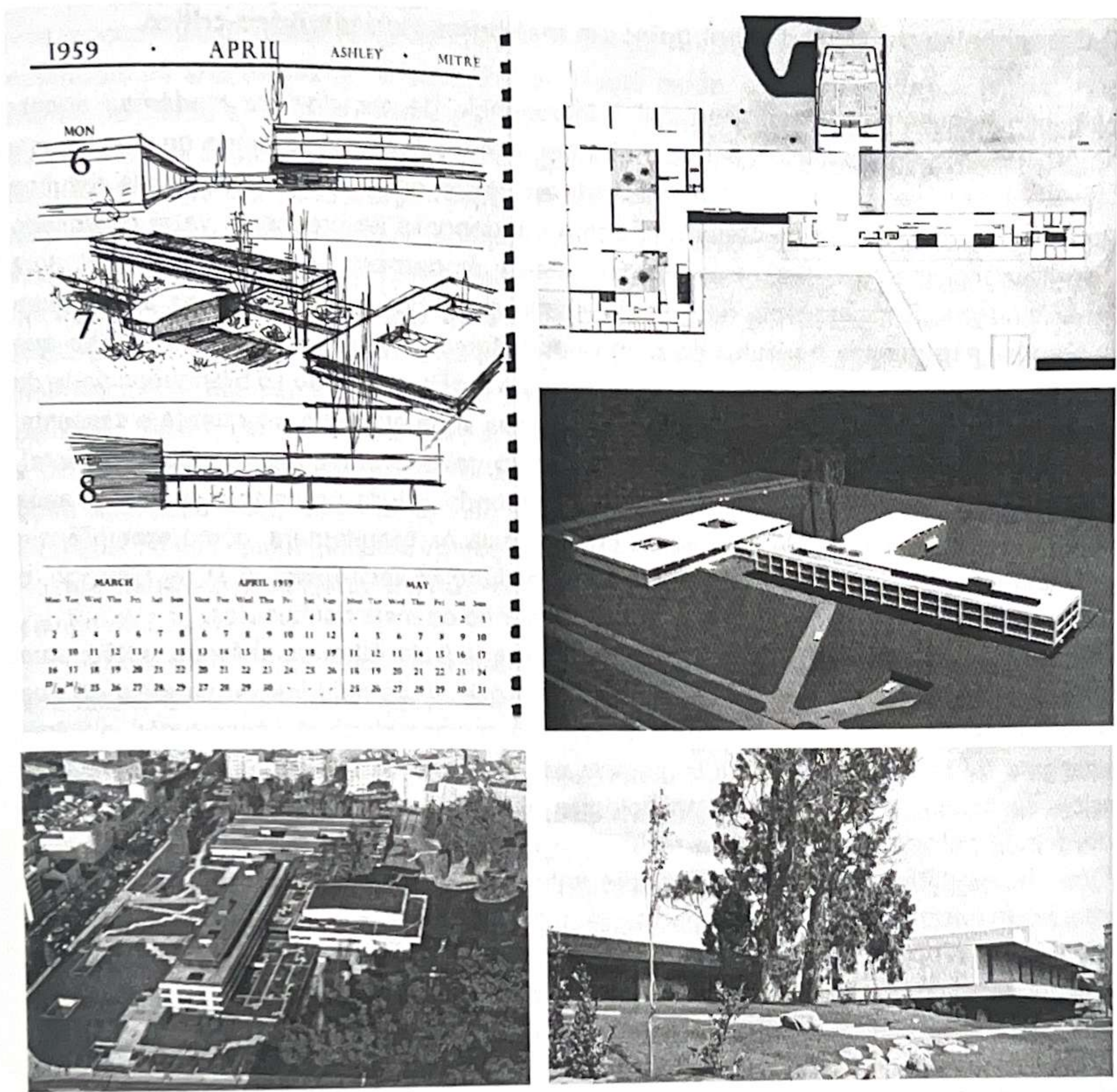
Figuras 1 a 5: Desenho, planta, maquete e fotografias de época. Fundação Calouste Gulbenkian. Fonte: Arquivo Ruy Athouguia.
