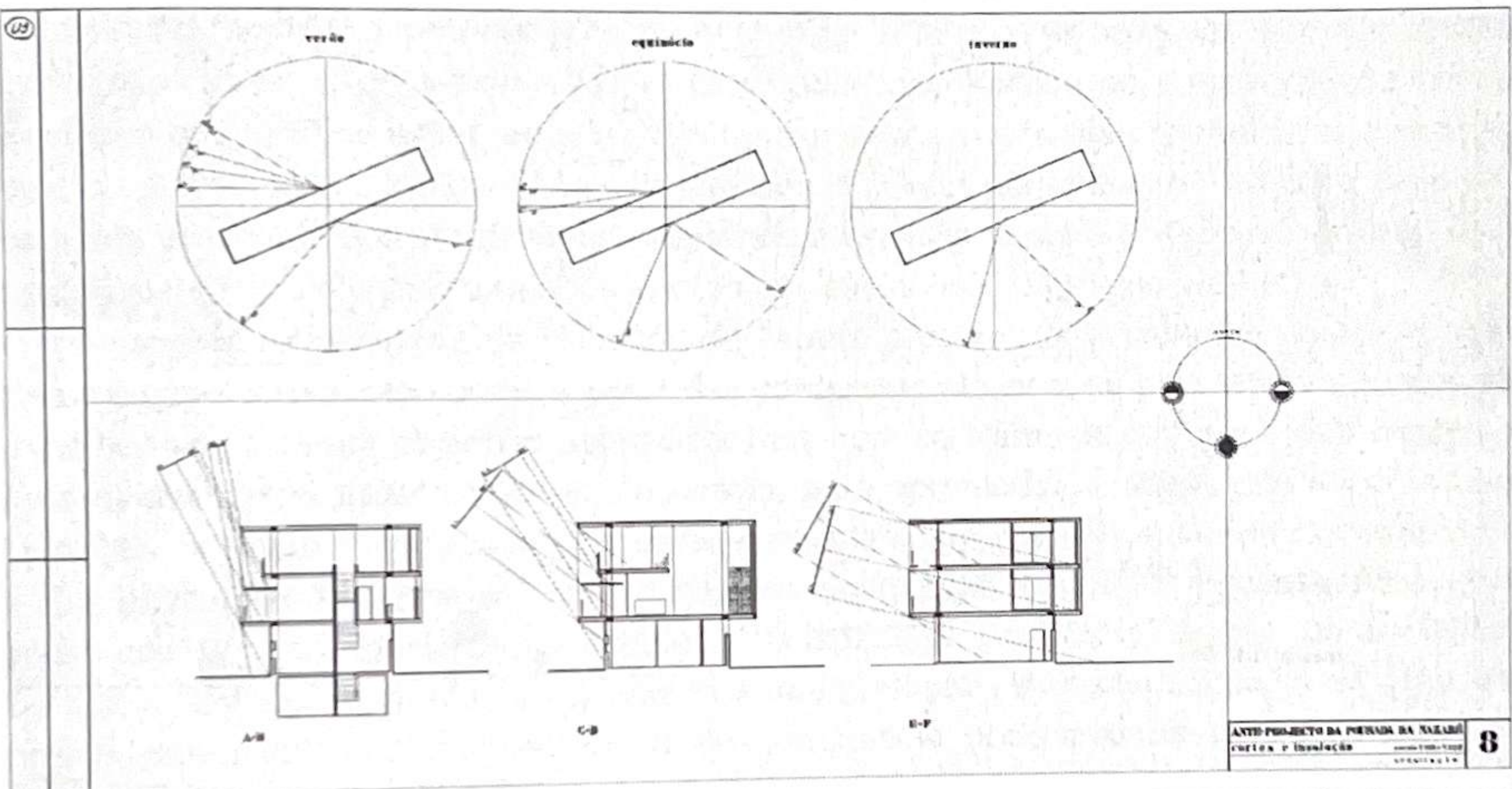
Figuras 10, 11, 12 e 13: Segunda versão da Pousada da Nazaré. Planta, estudos de orientação solar e perspectivas. Fonte: Arquivo Ruy Athougua.
