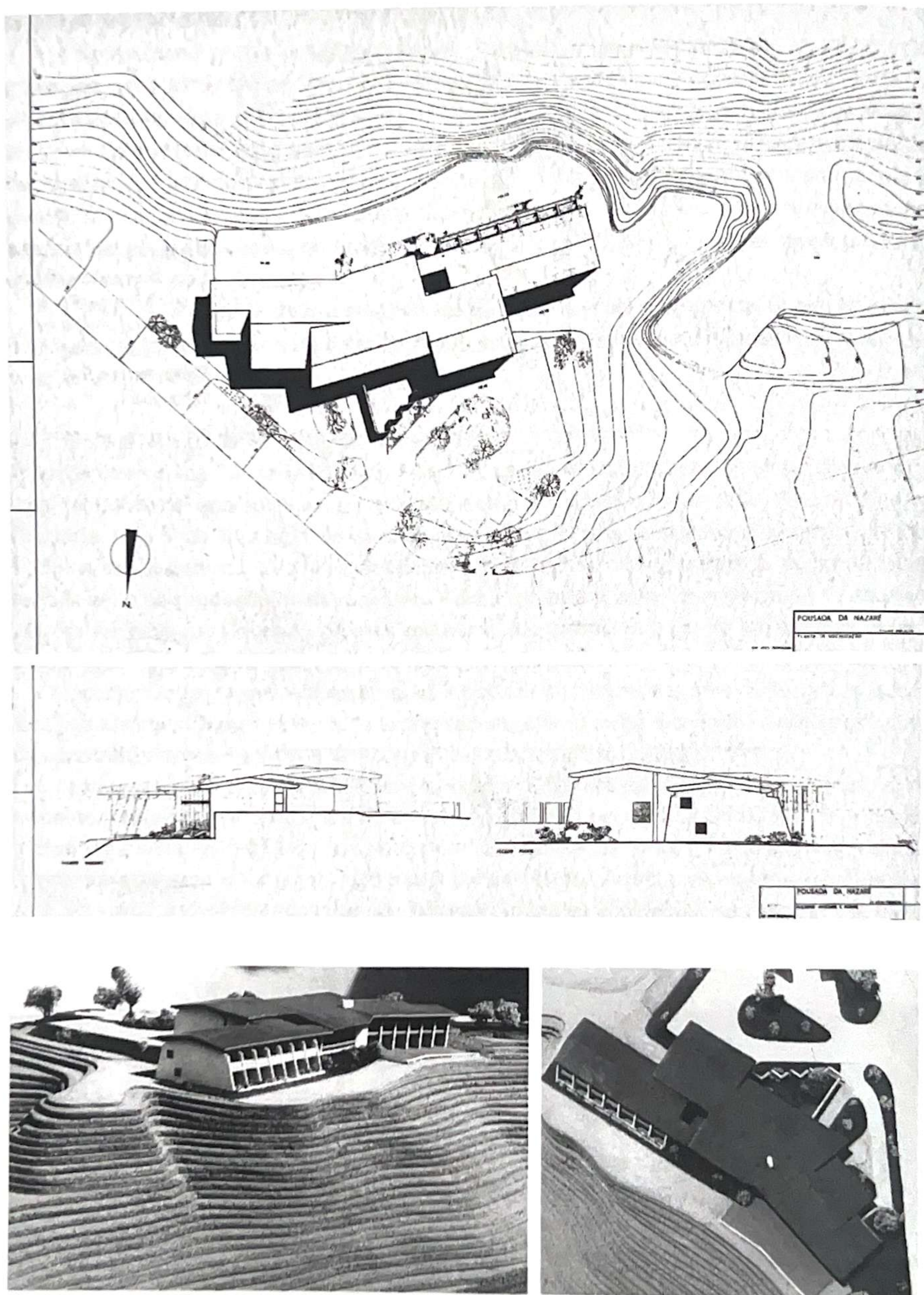
Figuras 14, 15, 16 e 17: Terceira versão. Planta, alçados e imagens da maquete. Pousada da Nazaré. Fonte: Arquivo Ruy Athouguia.
