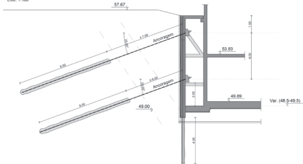
SEÇÃO TRANSVERSAL - 2 ANCORAGENS ESC. 1:100
