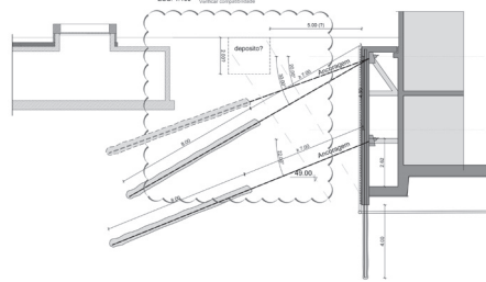
SEÇÃO TRANSVERSAL - 2 ANCORAGENS JUNTO AO EXISTENTE ESC. 1:100
