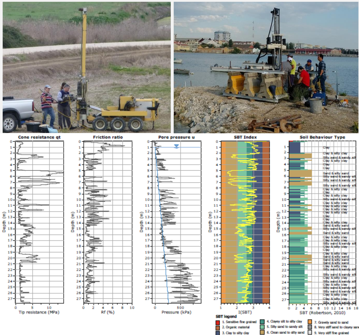
Figura 7 - Ensaios CPTu e registo da informação
