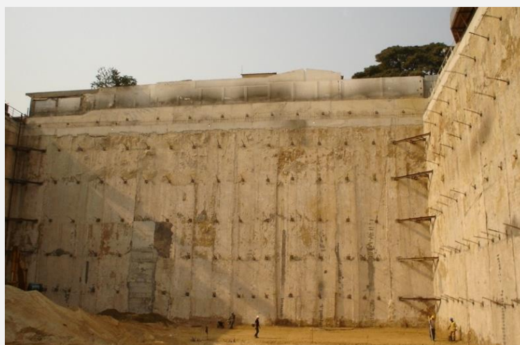
Figura 6 - Contenção com painéis de parede moldada, com espessura de 0,50 m, ancorados em 6 níveis em edifício de escritórios em Luanda, 2005
