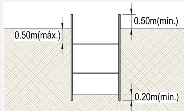
Figura 10 – Disposições construtivas a observar em valas entevadas
