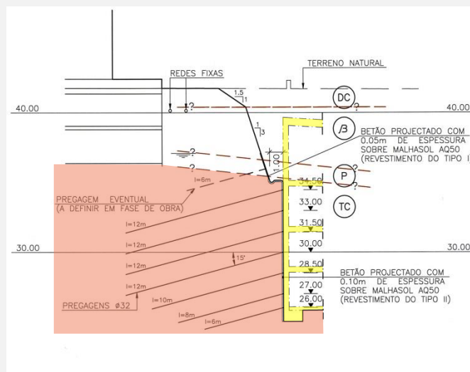
Figura 12 - Perfil transversal de uma contenção com revestimento de betão projetado pregado no Parque de Estacionamento de Miraflores, 2000
