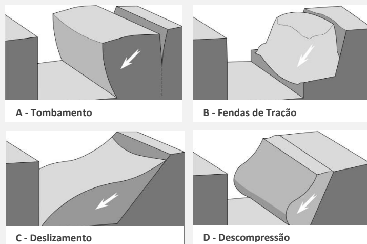
Figura 5 – Principais modos de rotura de taludes de escavação
