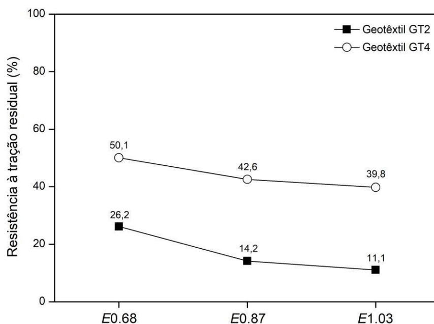
Figura 3 – Comparação das Resistências à Tração Residuais dos Geotêxteis GT2 e GT4 Após os Ensaios Climáticos E0.68 , E0.87 e E1.03 .
