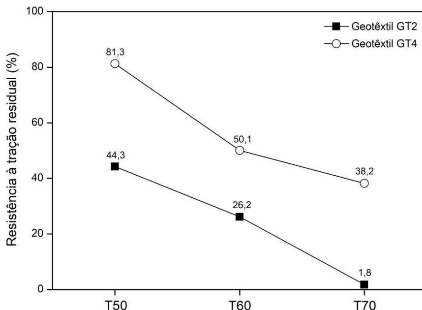
Figura 2 – Comparação das Resistências à Tração Residuais dos Geotêxteis GT2 e GT4 Após os Ensaios Climatéricos T50, T60 e T70.
