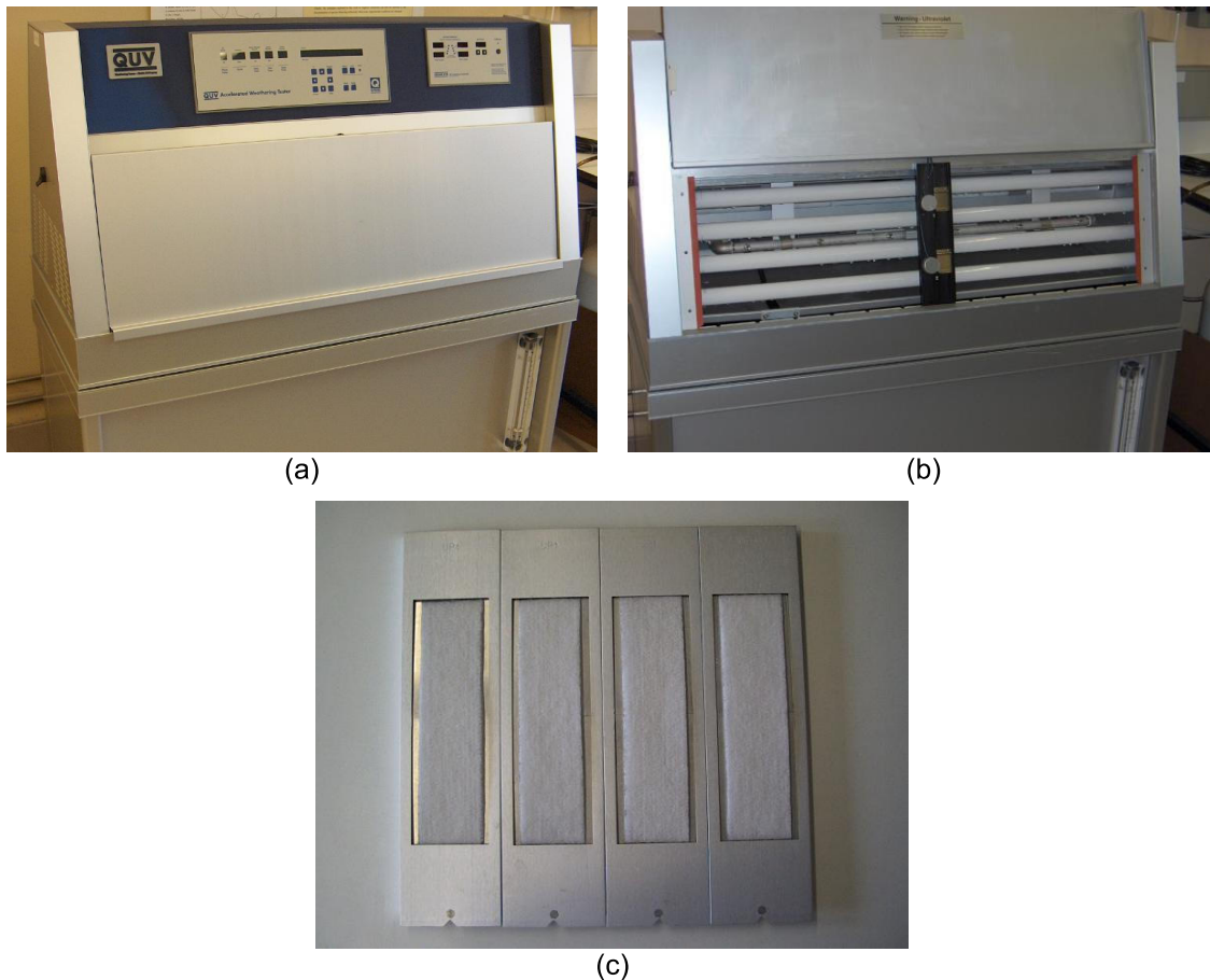
Figura 1 – Simulador QUV Weathering Tester: (a) Aspeto Exterior; (b) Antes da Colocação dos Suportes com Geotêxteis (Lâmpadas UVA-340); (c) Geotêxteis Colocados nos Suportes.
