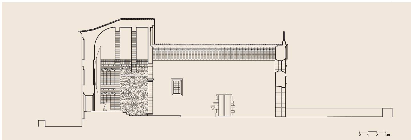
Corte longitudinal
