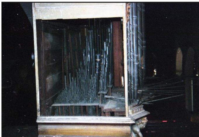
Figura 53. A parte lateral da caixa aberta; registo «em chamada» na fachada. Fonte: AOEO.
