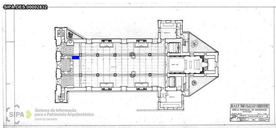
Figura 21. Planta de Igreja do Bom Jesus de Matosinhos com localização do órgão de tubos. Plana retirada de: www.monumentos.gov.pt/Site/APP_PagesUser/SIPAArchives.aspx?id=092910cf-8eaa-4aa2-96d9-994cc361eaf1&nipa=IPA.00004963 . [Consulta realizada em 26/05/2023].
