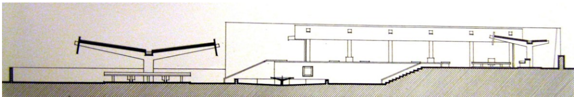
Fig. 10 Corte do Mercado da Vila da Feira, Arquitecto Fernando Távora, 1953-1959
