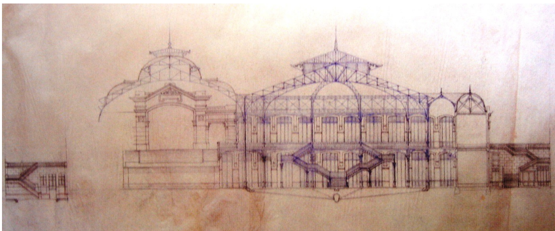
Fig 17 Corte longitudinal do Mercado do Bolhão, Ante-projecto, Eng. Xavier Esteves
