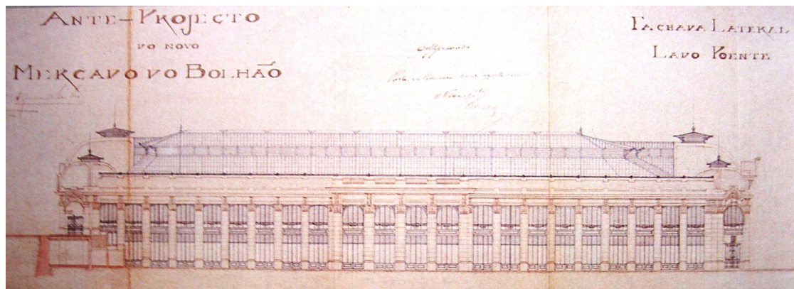
Fig 16 Fachada lateral poente do Mercado do Bolhão, Ante-projecto, Eng. Xavier Esteves
