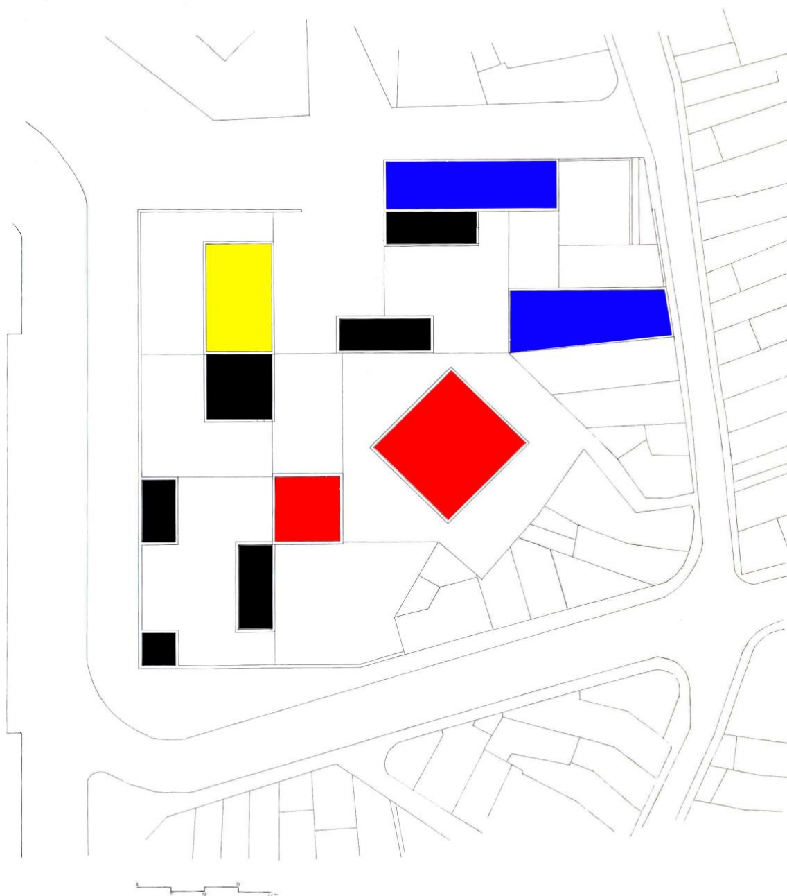
Planta de Coberturas Rúben Pinheiro | Projeto II | Centro de Mobilidade Internacional da Universidade do Porto | FAUP 2019/2020 | Escala 1:200
