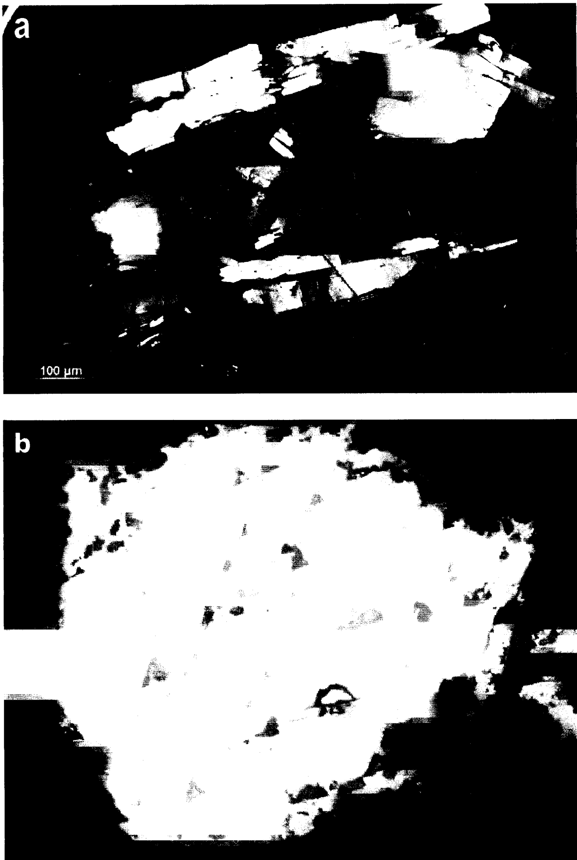
Fig. 2.14 - Imagens ao microscópio de reflexão de superfícies polidas de minério da mina do Borrageiro, com cristais de molibdenite em a) (em nicóis cruzados) e blenda com a substituição típica de calcopirite (amarela) em b) (em nicóis paralelos).
