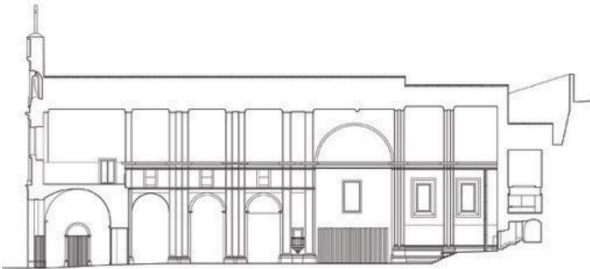
Fig. 5.6 - corte longitudinal da igreja de São Francisco
