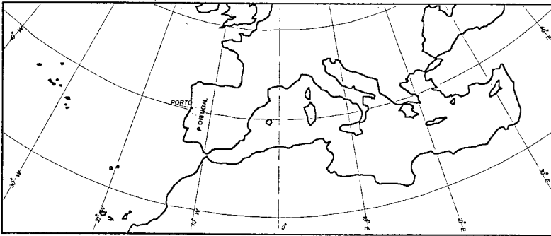
Fig. 2 – Localização de Portugal na cintura das perturbações de oeste.
