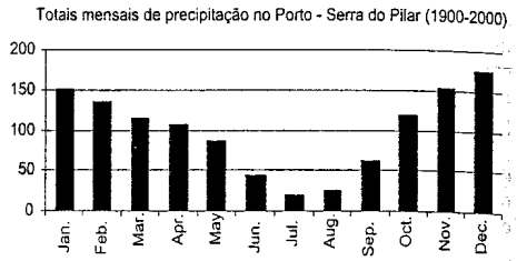
Fig. 7 - Precipitação total mensal no Porto durante o séc. XX.
