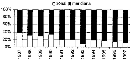
Fig. 6 - Comparação entre a frequência de ocorrência de situações de circulação zonal e meridiana em altitude sobre Portugal (1987-97).
