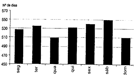
Fig. 8 - Frequência de ocorrência de precipitação no Porto em cada um dos dias da semana (1978-98).
