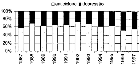
Fig. 5 - Comparação entre a frequência de ocorrência de situações anticiclónicas e de depressão na baixa atmosfera em Portugal (1987-97).
