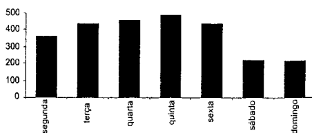
Fig. 9 – Número de dias em que a concentração de CO, NO x , SO 2 , C x H y ou Pb ultrapassou o percentil 90 na Área Metropolitana do Porto (1989-97).
